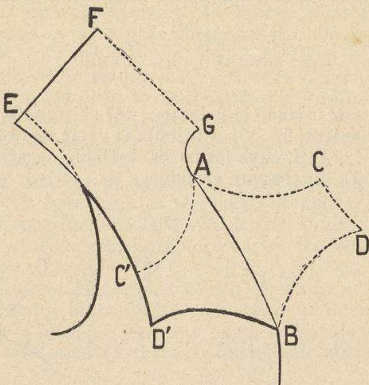
Fig. 152 ( \frac{1}{5} del tamaño real).—Parte posterior del cuello.
