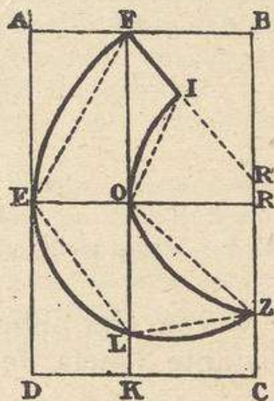
Fig. 118 ( \frac{1}{5} del tamaño real). Cuello de bordes redondos.
