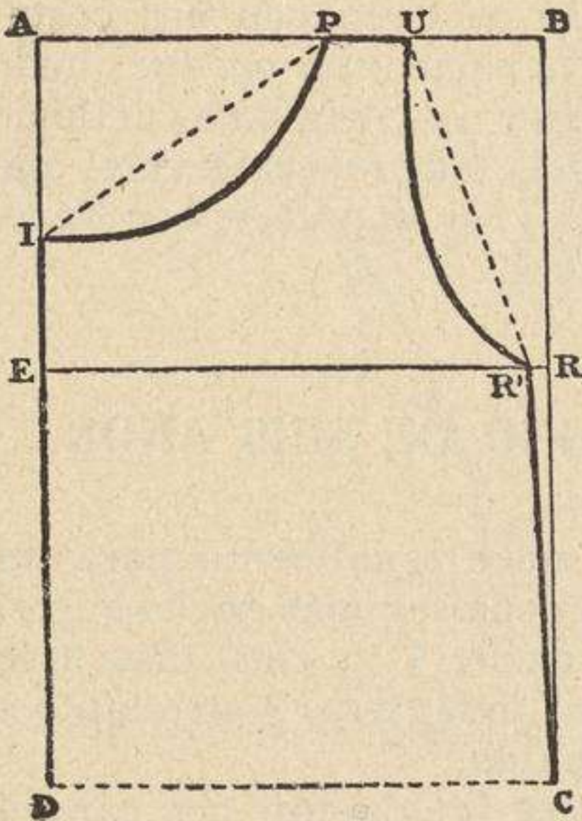
Fig. 154 ( \frac{1}{5} del tamaño real). Espalda del delantal.
