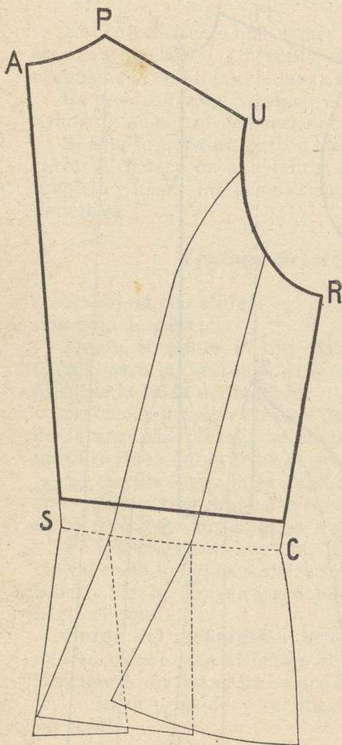
Fig. 36.—Espalda del bolero
