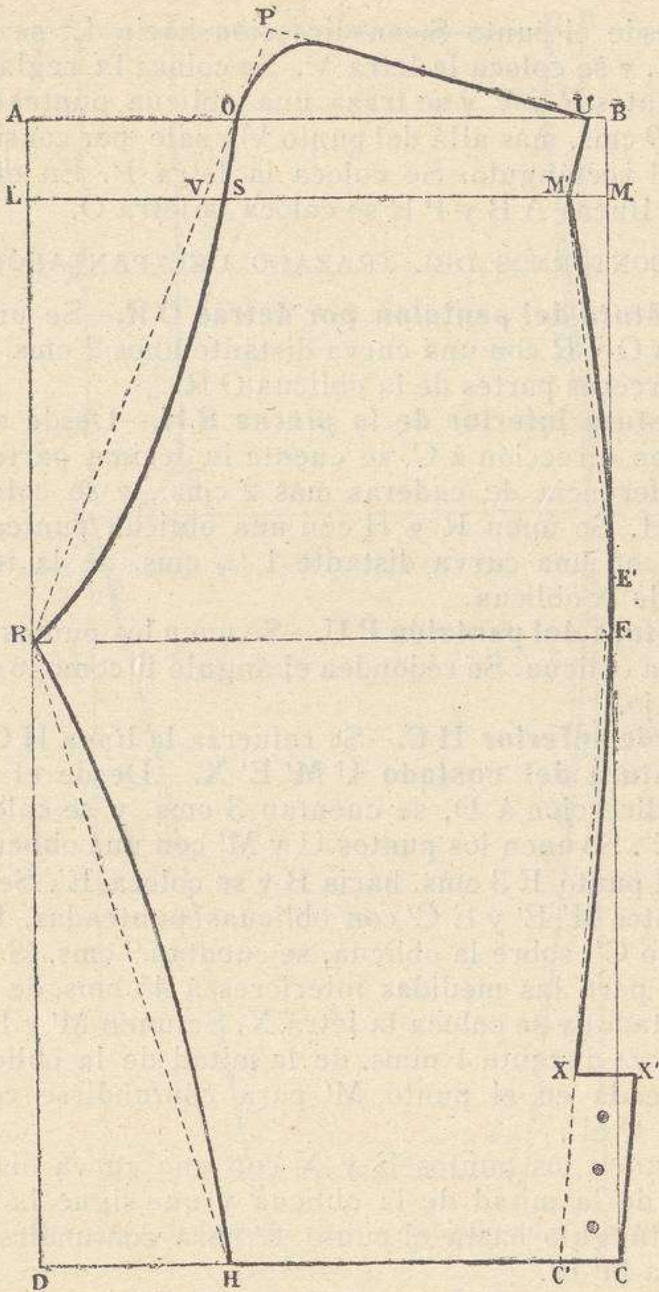
Fig. 79 ( \frac{1}{5} del tamaño real).—Parte posterior del pantalón.
