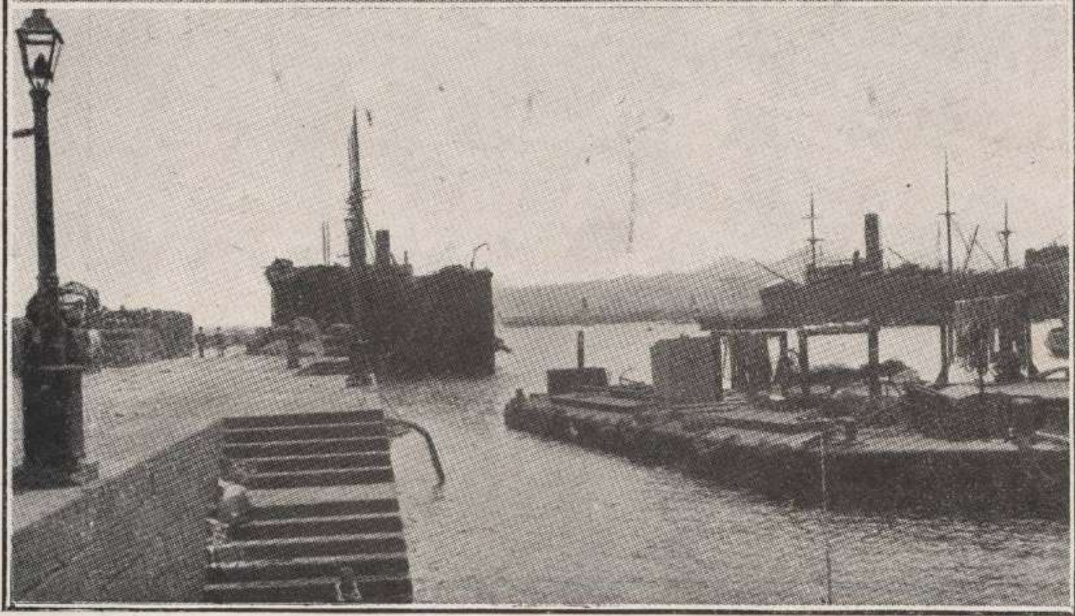
1.º Depósito de 64.000 metros cúbicos de capacidad para regular el servicio. 2.º Instalación para el abastecimiento de buques, capaz para suministrar doscientas toneladas por hora.
