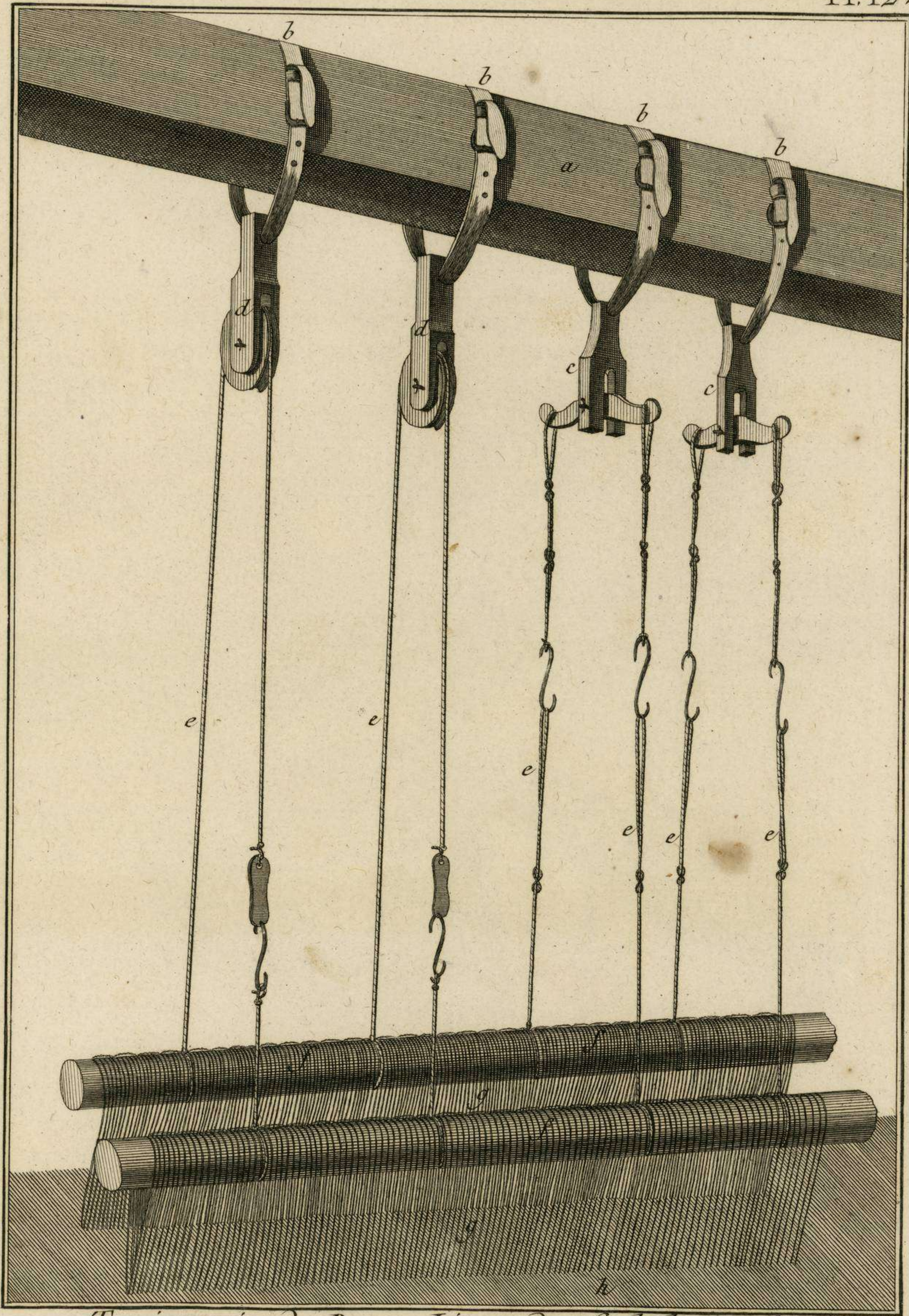
Tapissérie de Basse Lisse des Gobelins, Service des Sautriaux ordinaires avec les Poulies
