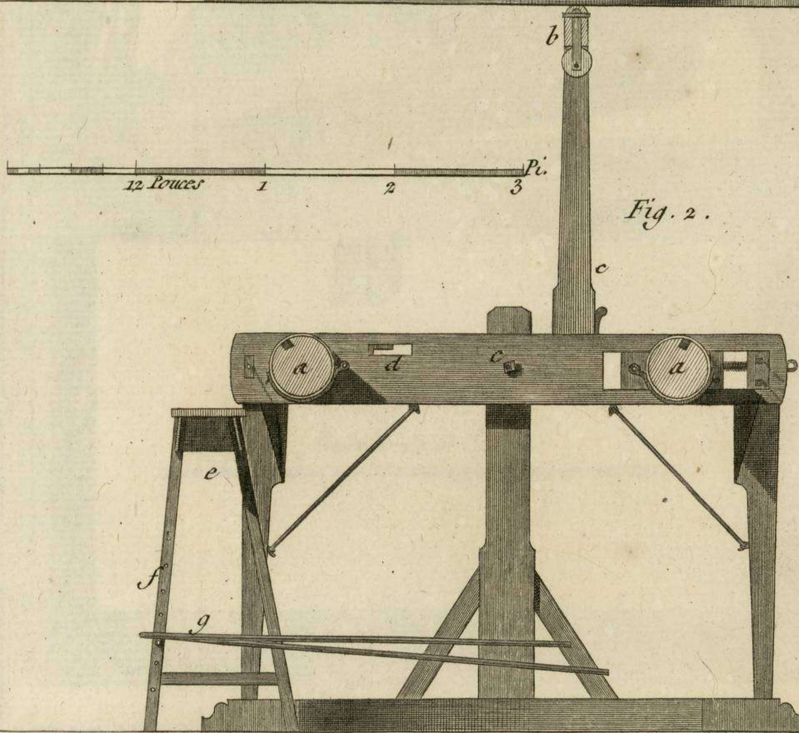
Tapissierie de Basse Lisse des Gobelins. Benard diract Elevation Latérale et Coupe Géométrale du petit Métier pour les Jeunes Eleves.
