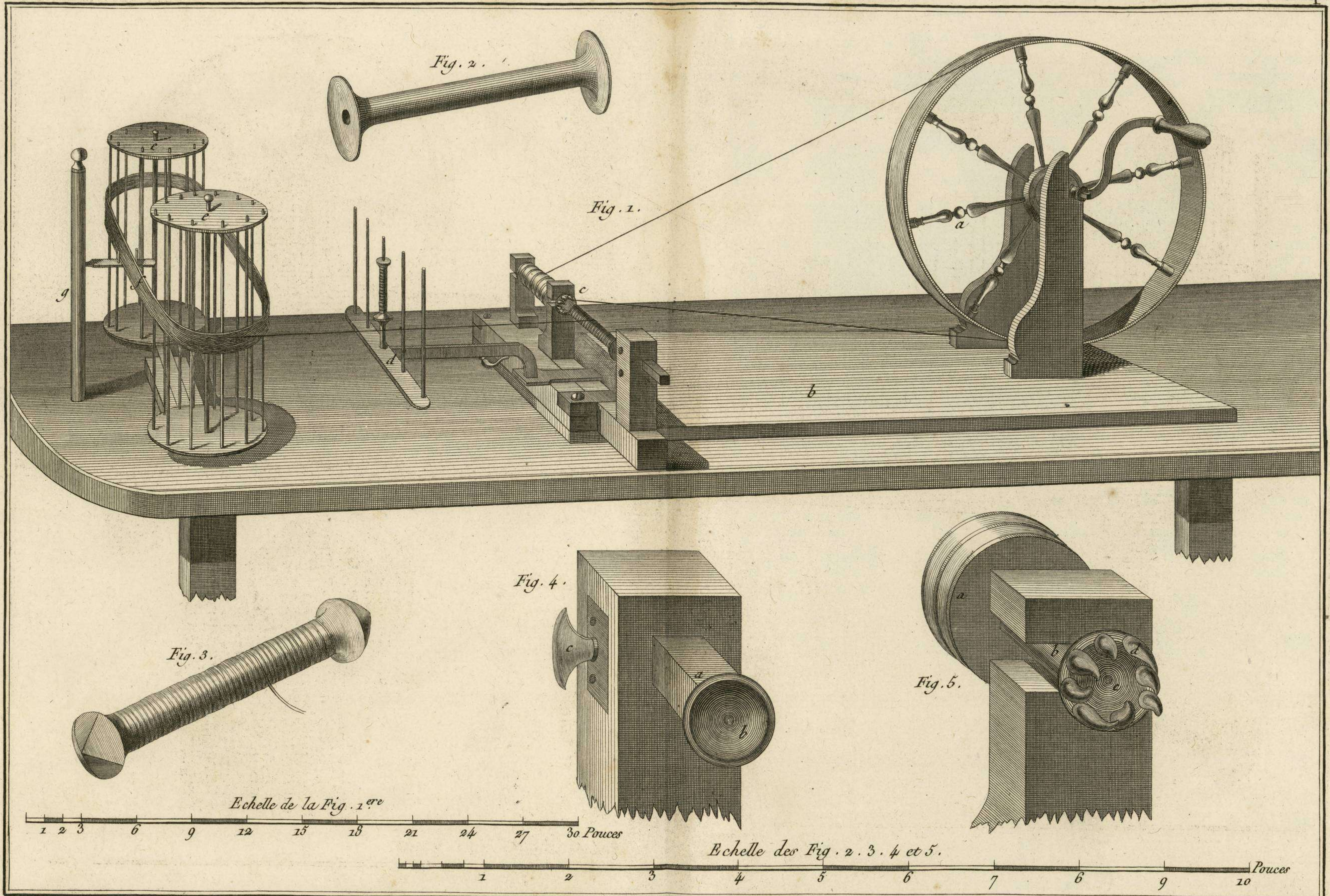
Tapisserie de Basse Lisse des Gobelins, Rouet à diviser les Laines sur les Bobines et sur les Flûttes, et 2 Développemens.
