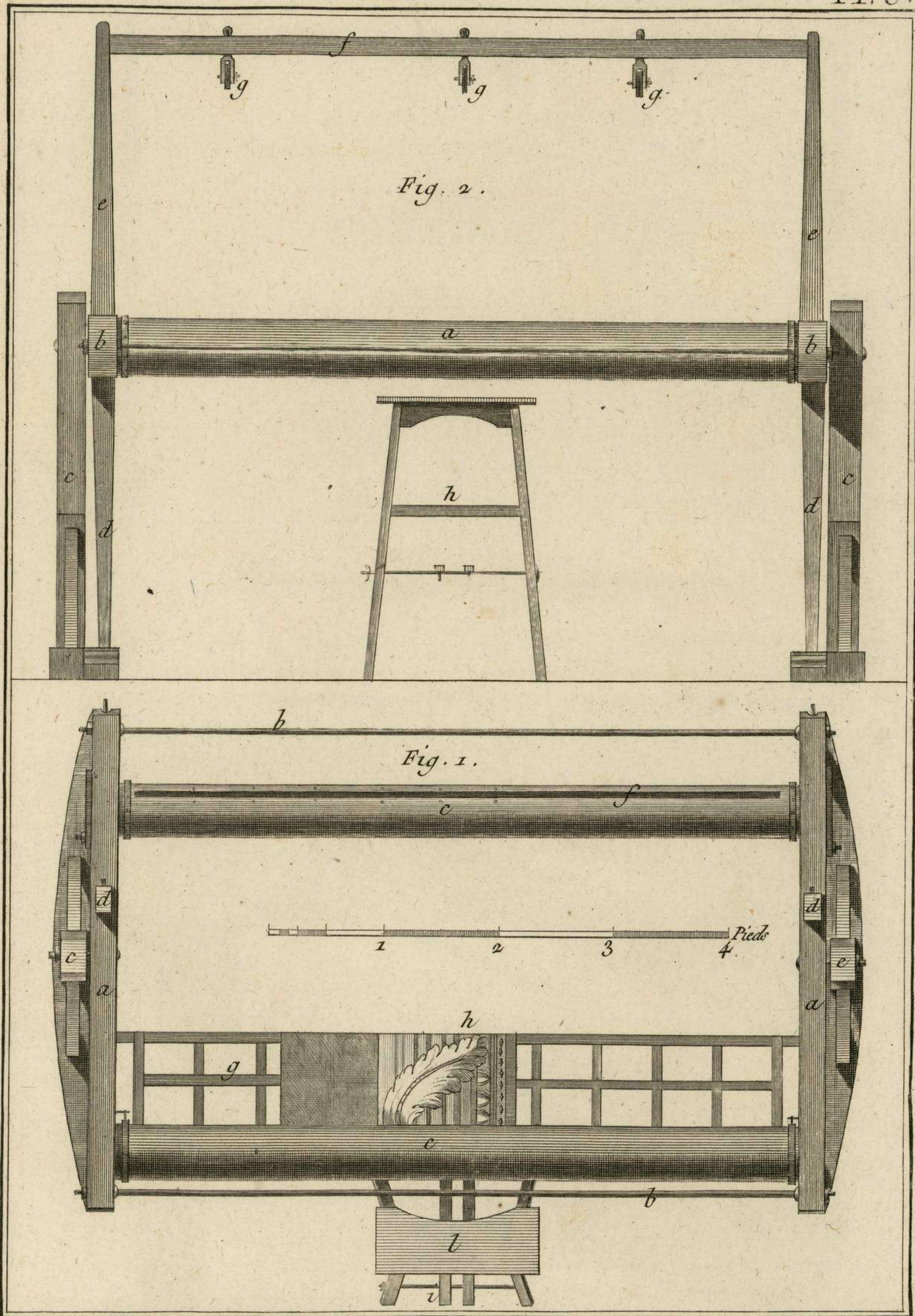
Tapisserie de Basse Lisse des Gobelins, Bernard Directeur Plan et Elevation du petit Metier pour les jeunes Eleves.
