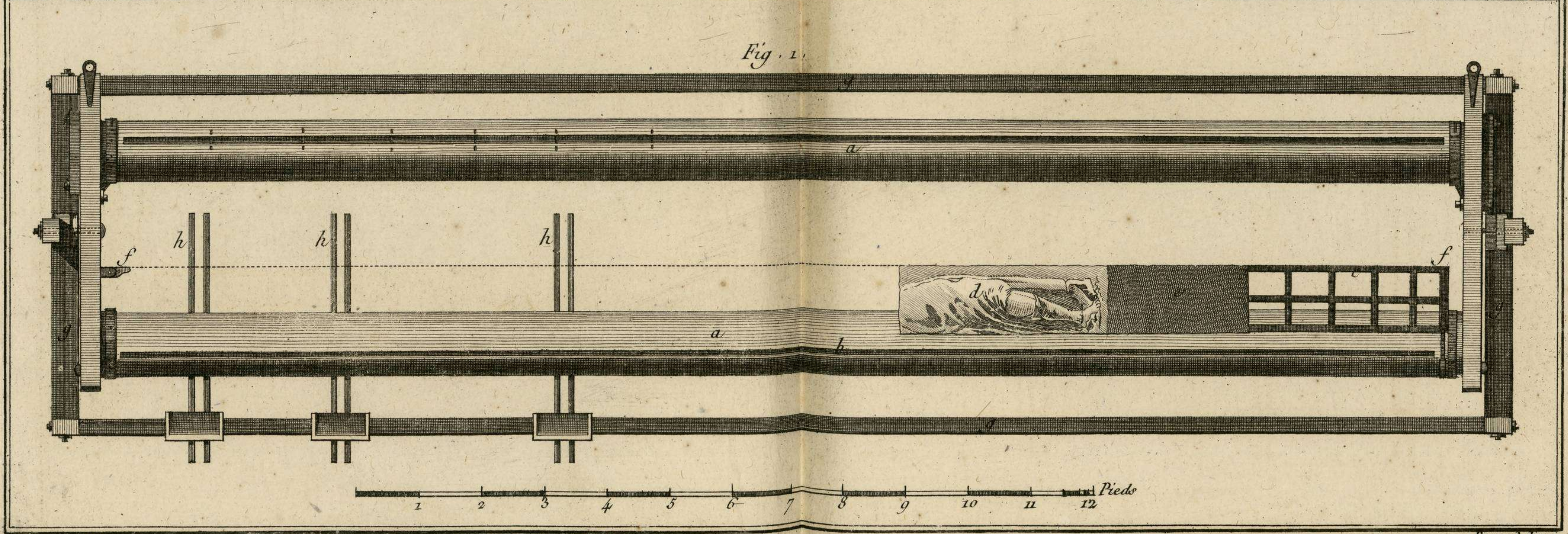
Tapisserie de Basse Lisse des Gobelins, Plan et Elevation du Metier de Basse Lisse de la composition de M. de Vaucanson.
