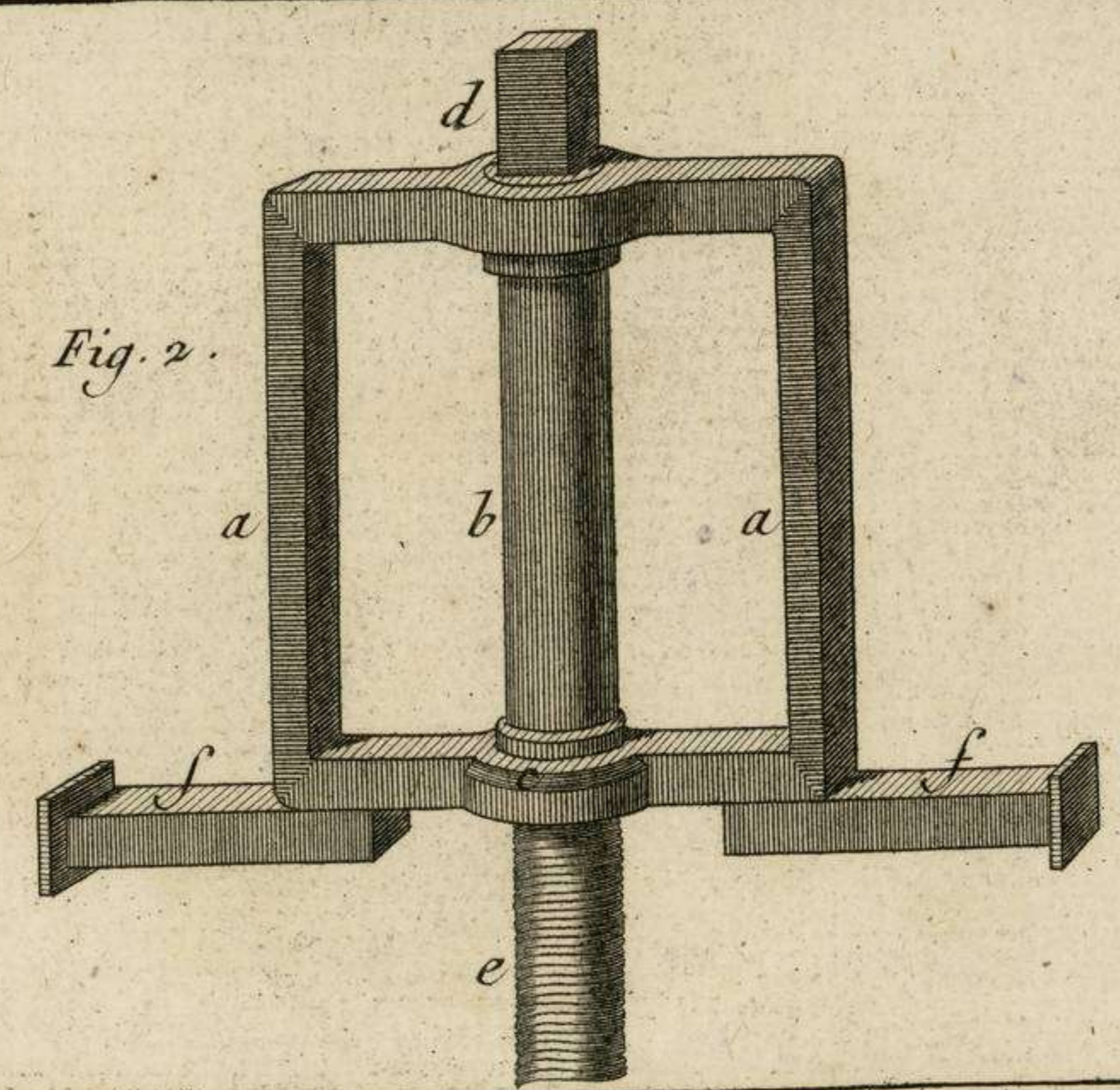
Tapissierie de Haute Lisse des Gobelins, Vue du Metier monte' avec la nouvelle Machine pour faciliter le bandage des fils et avec 2 hommes seulement. Developpement de cette Machine
