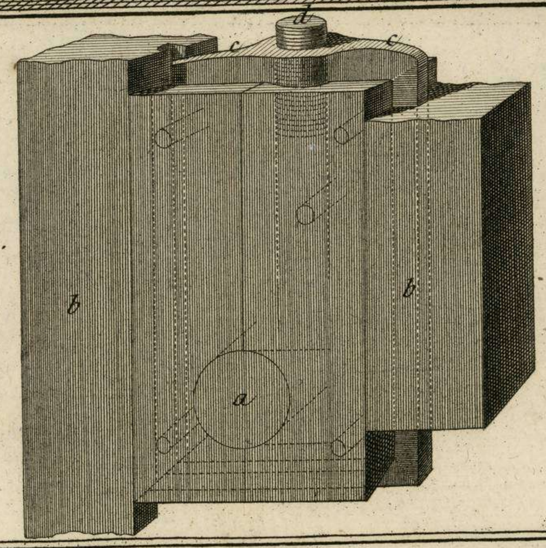
Tapissierie de Haute Lisse des Gobelins, Vue du Metier monte' avec la nouvelle Machine pour faciliter le bandage des fils et avec 2 hommes seulement. Developpement de cette Machine
