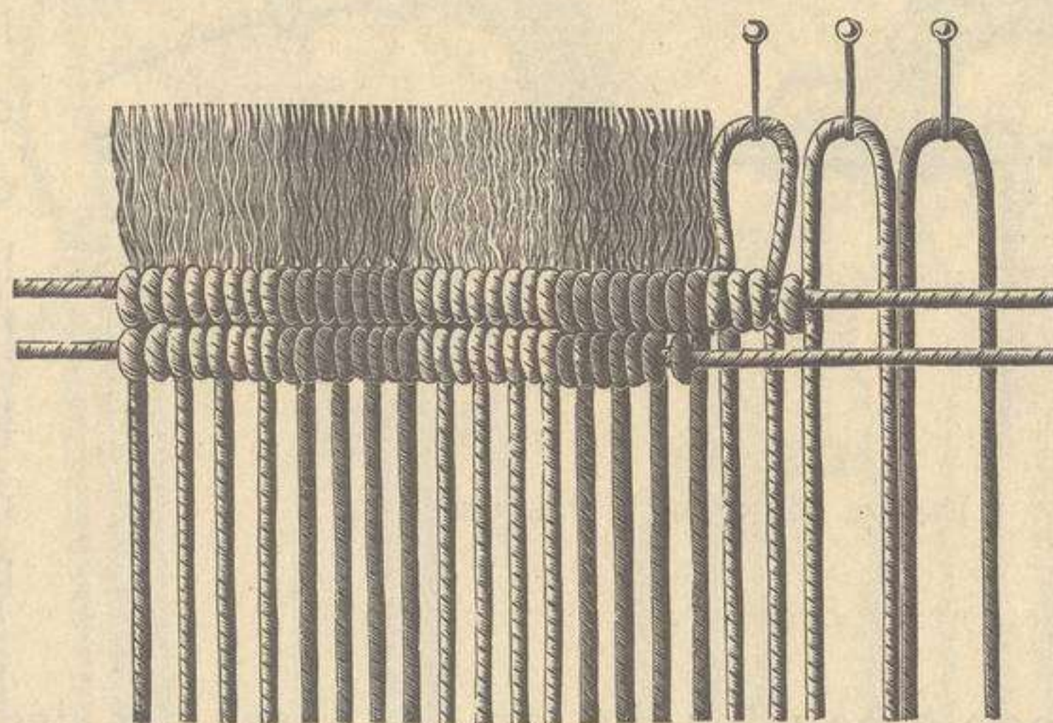
FIG. 5. MONTAGE A TÊTES FRANGÉES.
