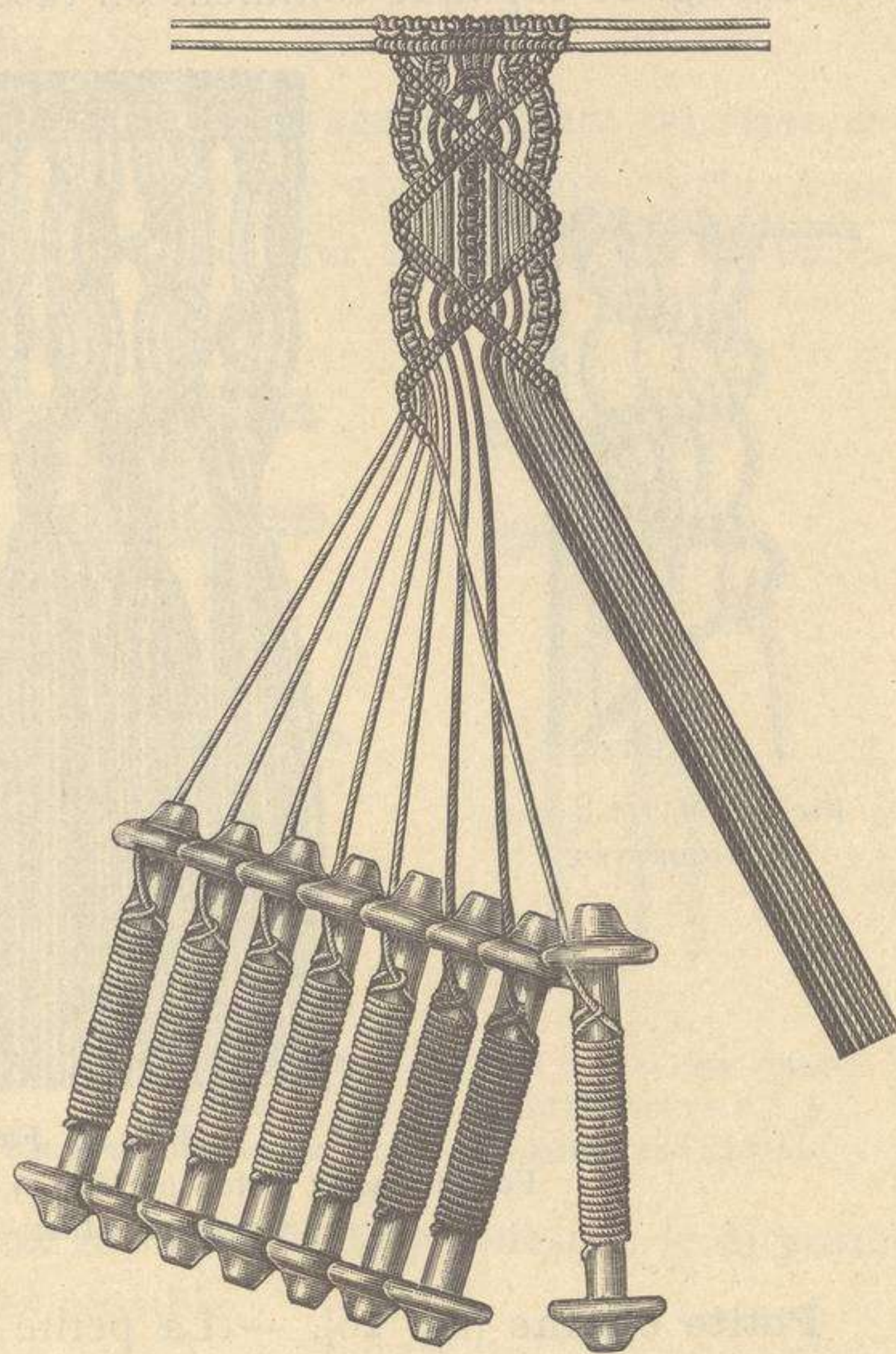
FIG. 32. GALON CONFECTIONNÉ AVEC LA NAVETTE A MACRAMÉ.
