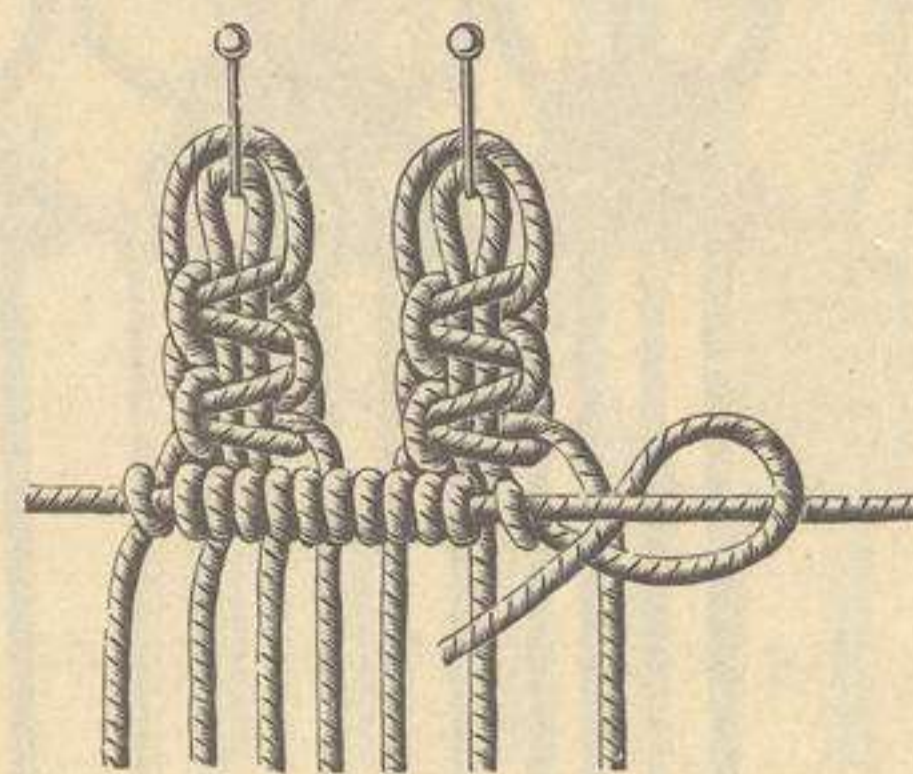
FIG. 7. MONTAGE A PICOTS AVEC DEUX NŒUDS PLATS.
