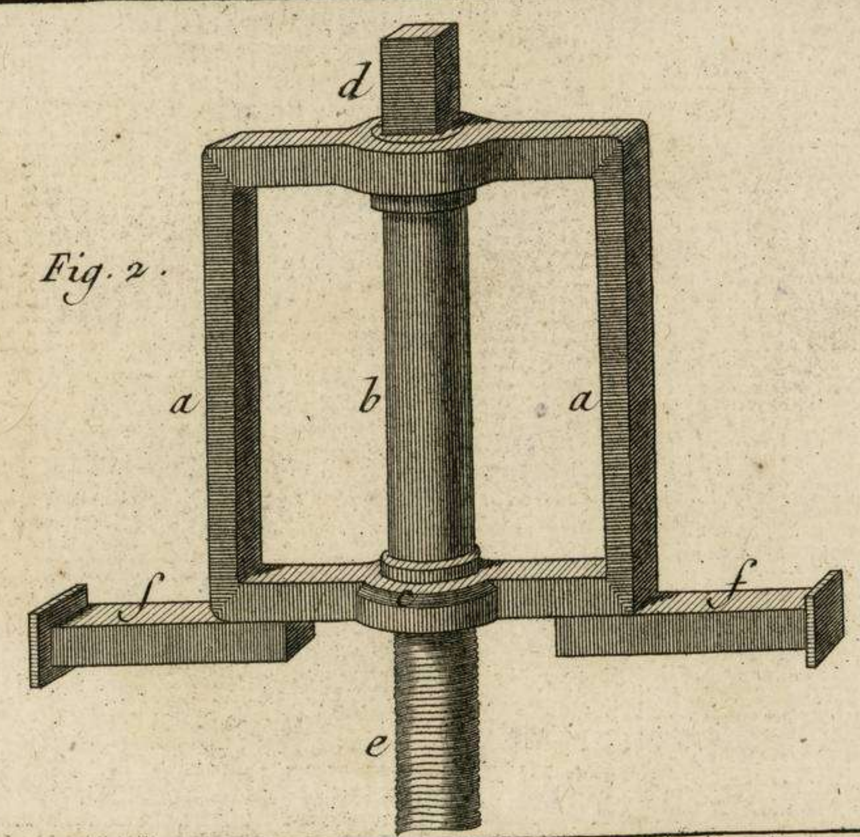
Tapissierie de Haute Lisse des Gobelins, Vue du Metier monte' avec la nouvelle Machine pour faciliter le bandage des fils et avec 2 hommes seulement. Developpem t de cette Machi ne
