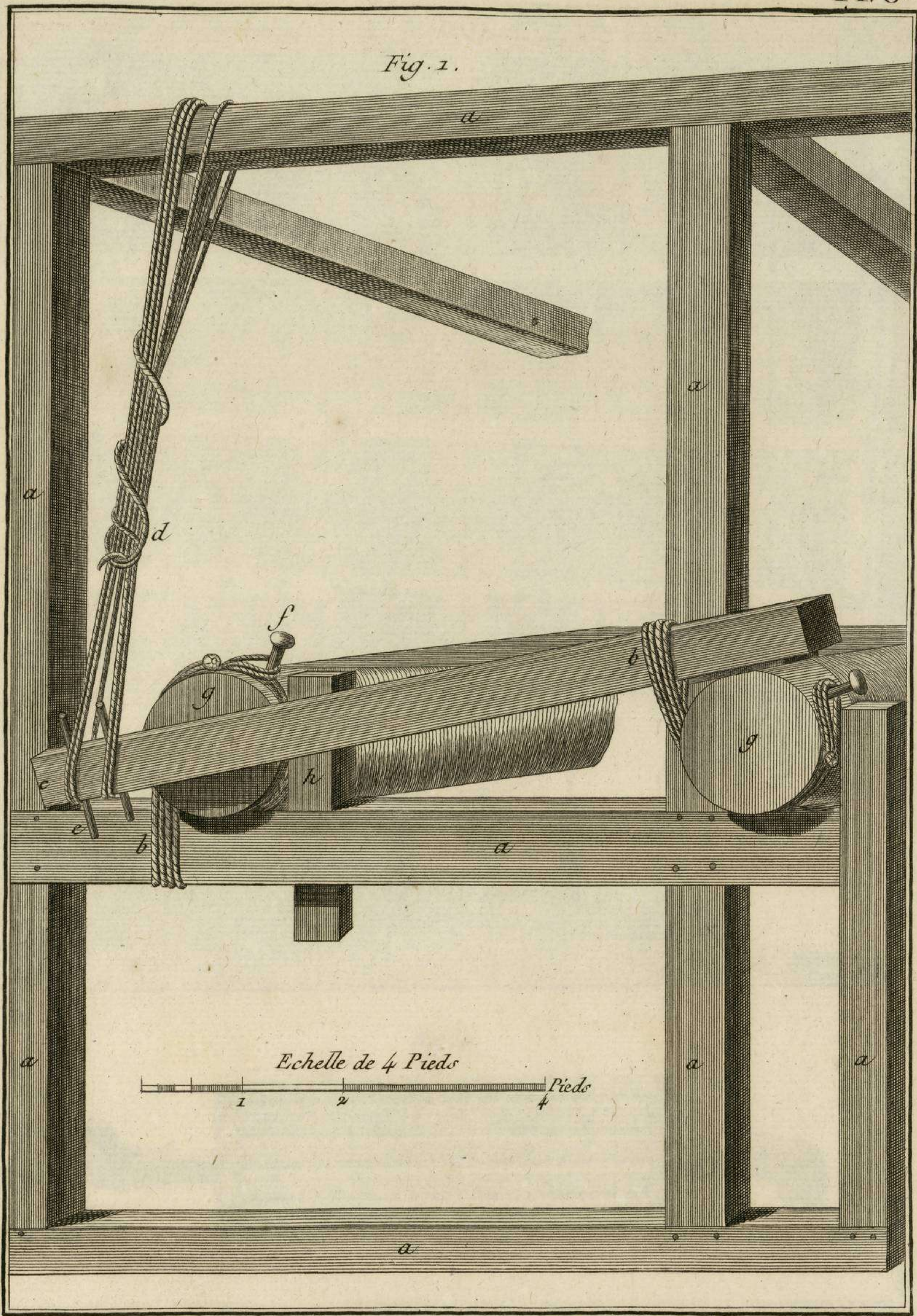
Tapisserie de Basse Lisse des Gobelins, Benard diract Ancienne maniere de Bender avec le Tentoir les Rouleaux des Metiers 175
