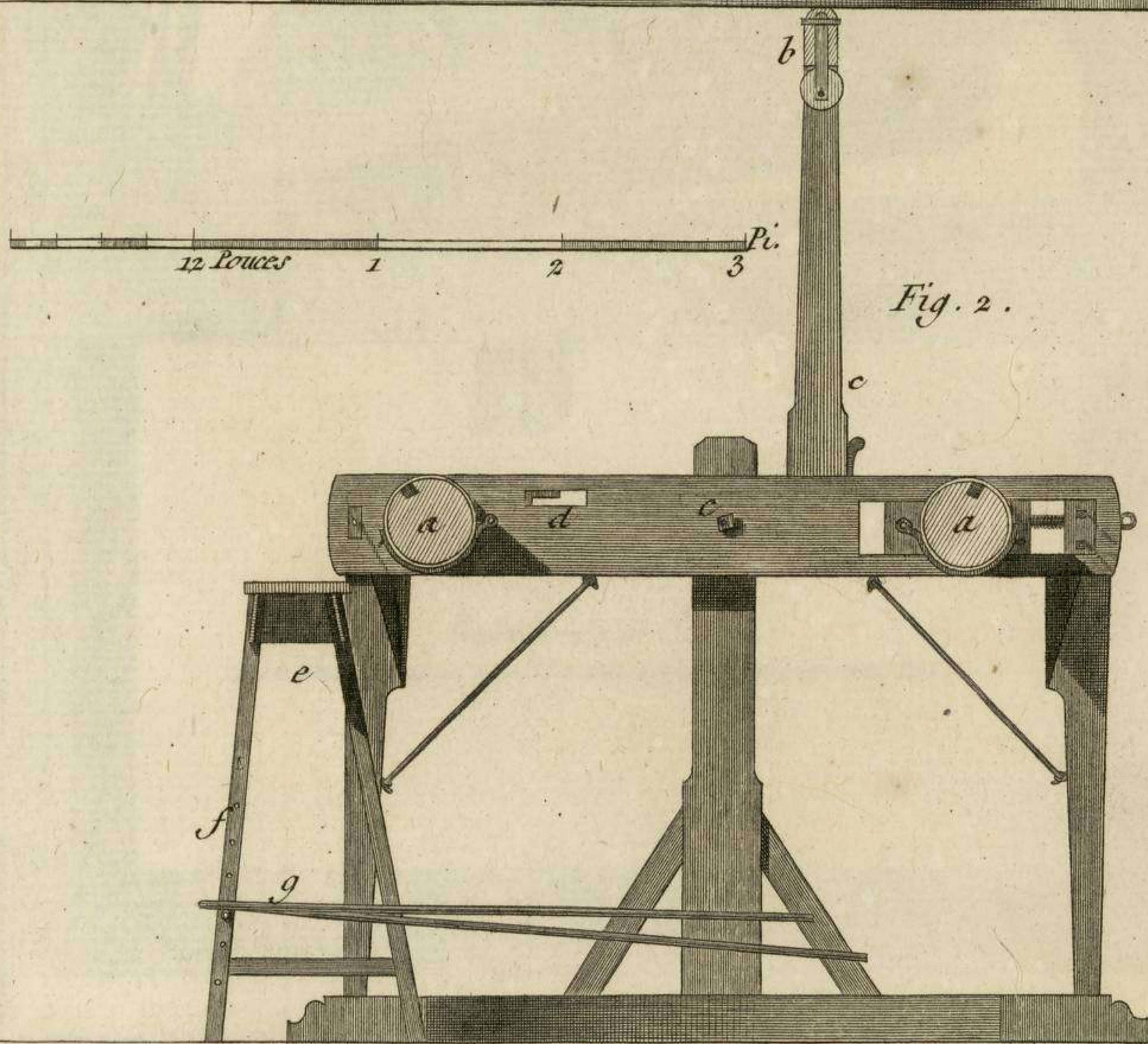
Tapissierie de Basse Lisse des Gobelins. Elevation Latérale et Coupe Géométrale du petit Métier pour les Jeunes Eleves.
