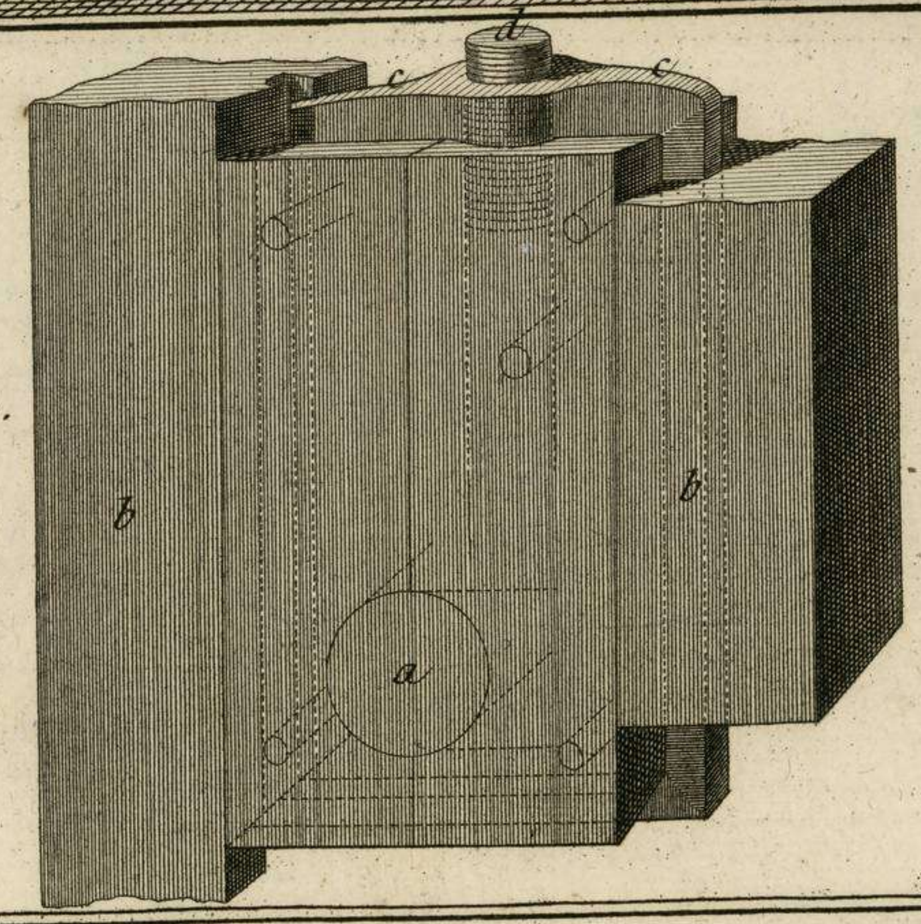
Tapissierie de Haute Lisse des Gobelins, Vue du Metier monte' avec la nouvelle Machine pour faciliter le bandage des fils et avec 2 hommes seulement. Developpem t de cette Machi ne
