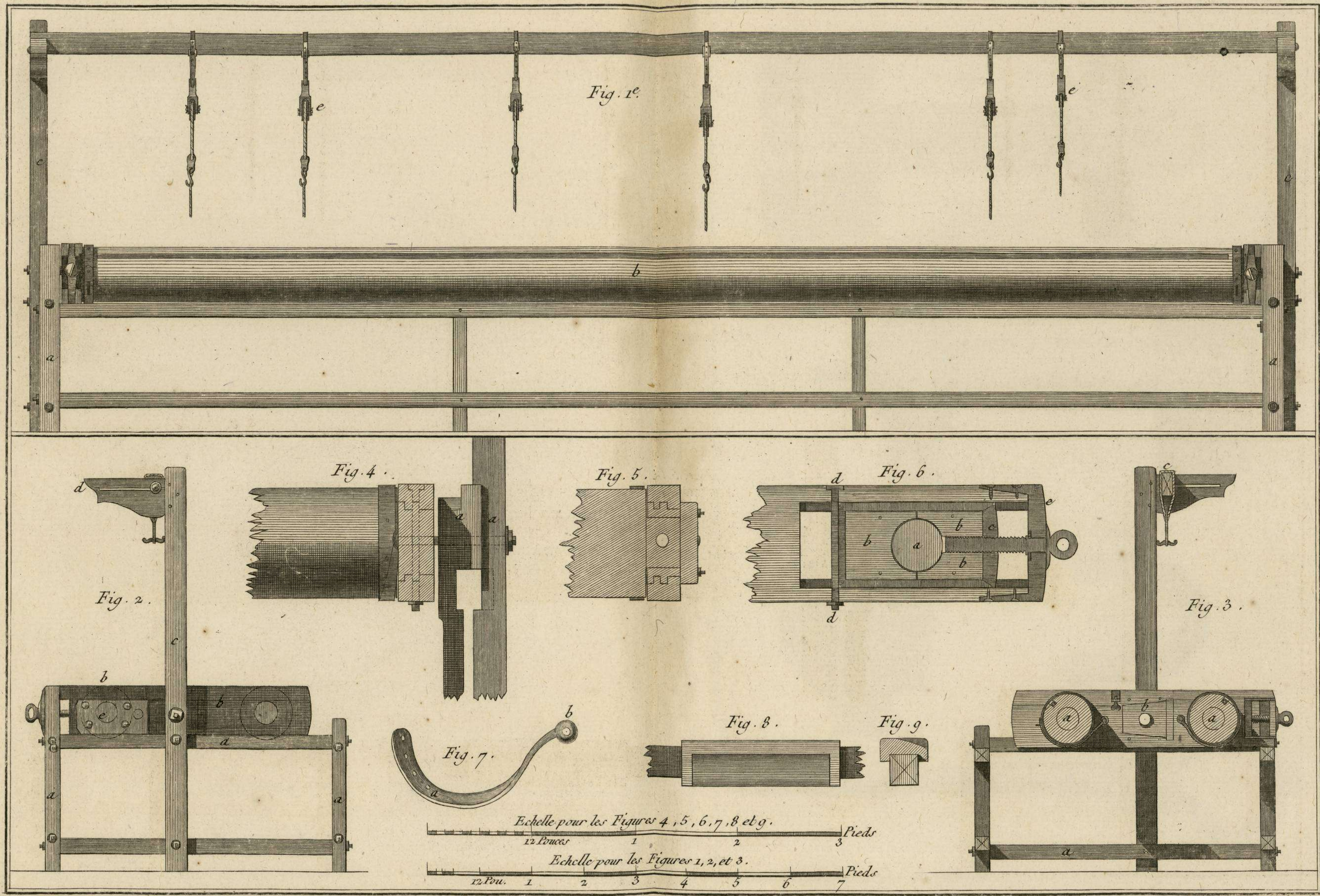
Tapisserie de Basse Lisse des Gobelins, Elevations et proportions Géométrales, Coupes, et Développemens du Métier de Basse Lisse.
