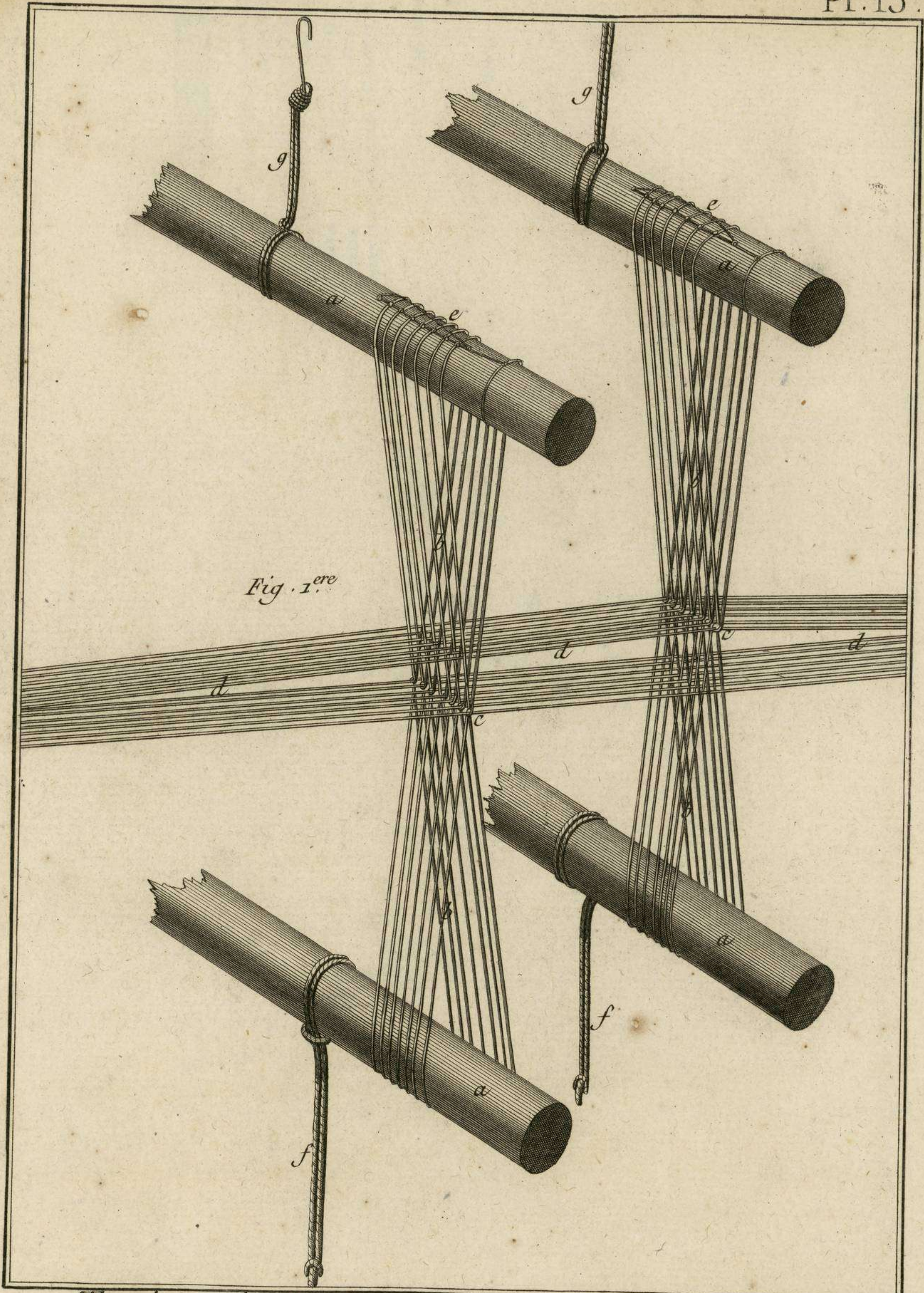
Tapisserie de Basse Lisse des Gobelins Benard directeur Construction des Lames et Fils de Croisure pour le passage de la Flûte 178
