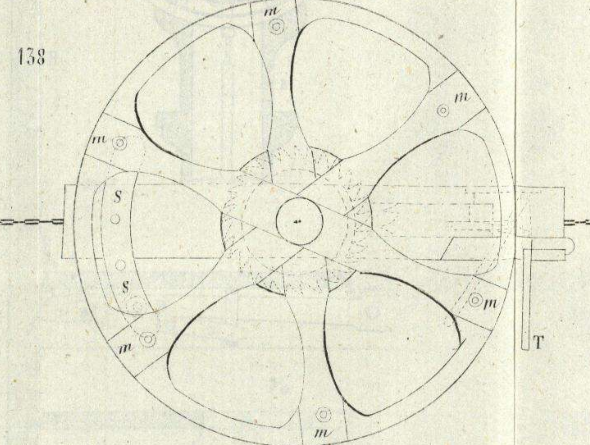
Seccion de un carro para riego.
