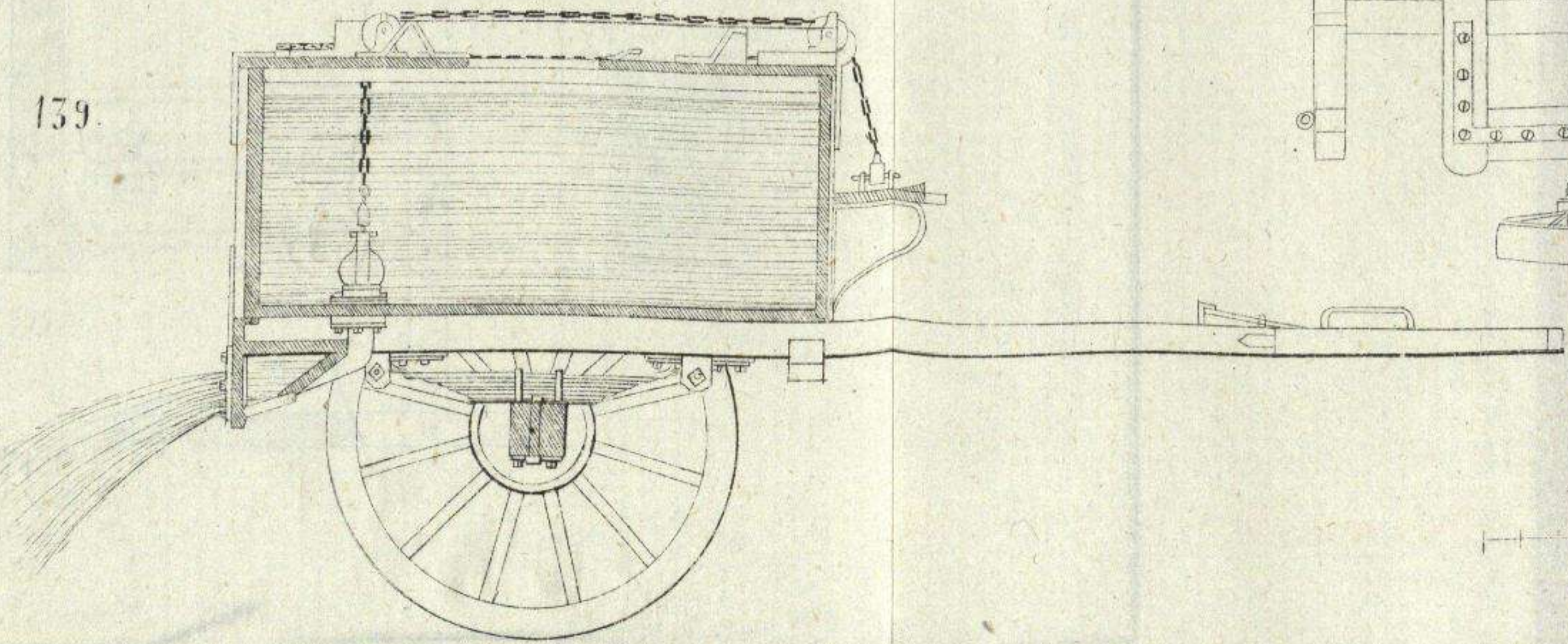
Seccion de un carro para riego.
