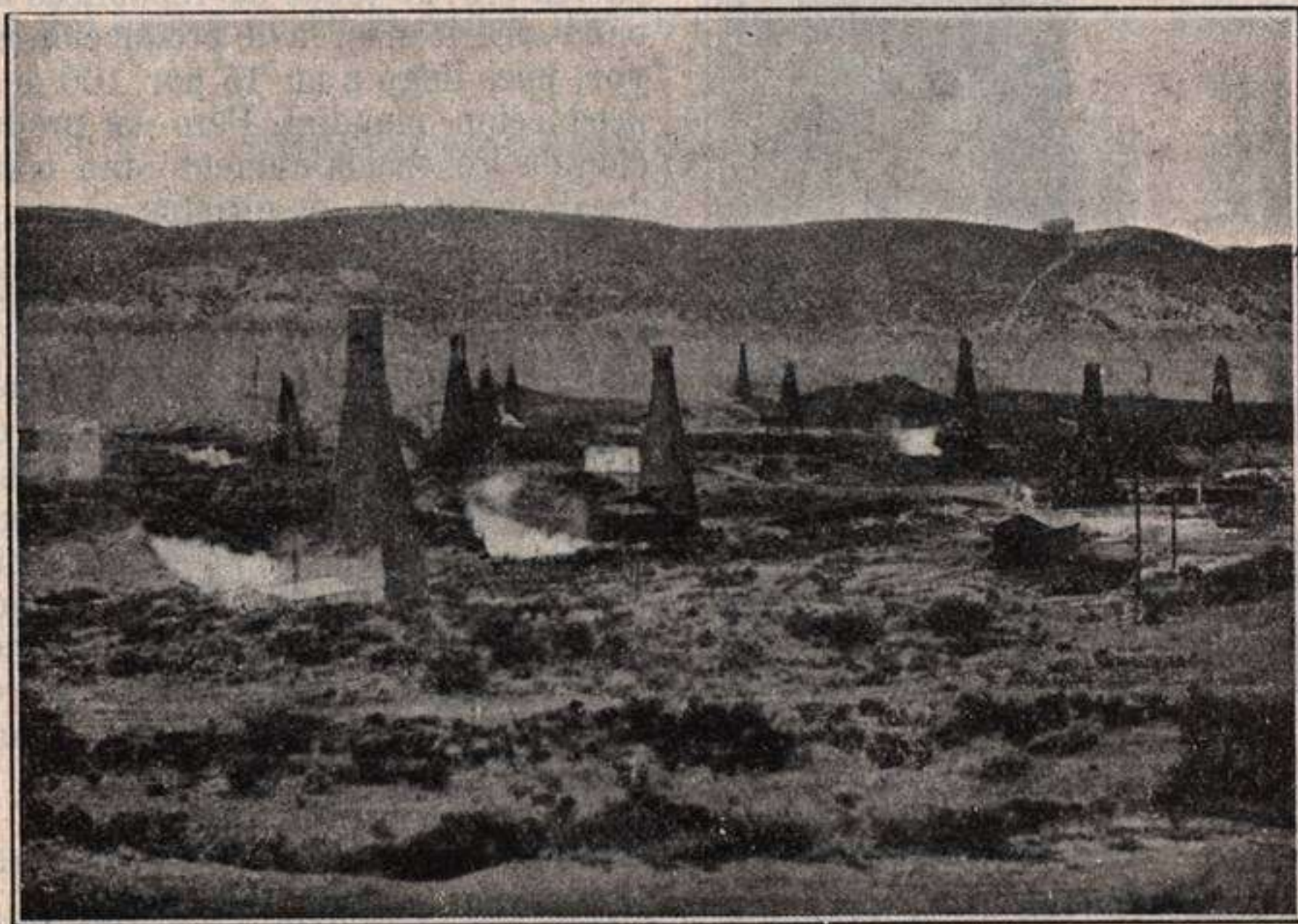
Fig. 248.—Yacimientos de petróleo de Comodoro Rivadavia (Argentina). Vista general de la mayoría de los pozos productivos de la Compañía Astra. (Fot. J. M. Sobral, comunicada por el ingeniero L. E. Vicart).
