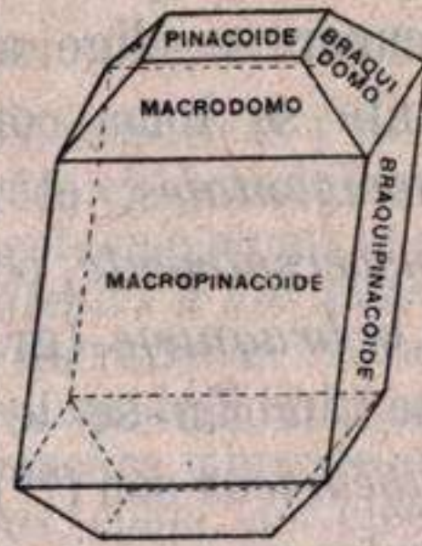
Fig. 113.-Forma compuesta de pinacoides y domos.
