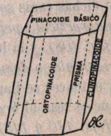
Fig. 117.—Combinación de pinacoides y prisma oblicuo.
