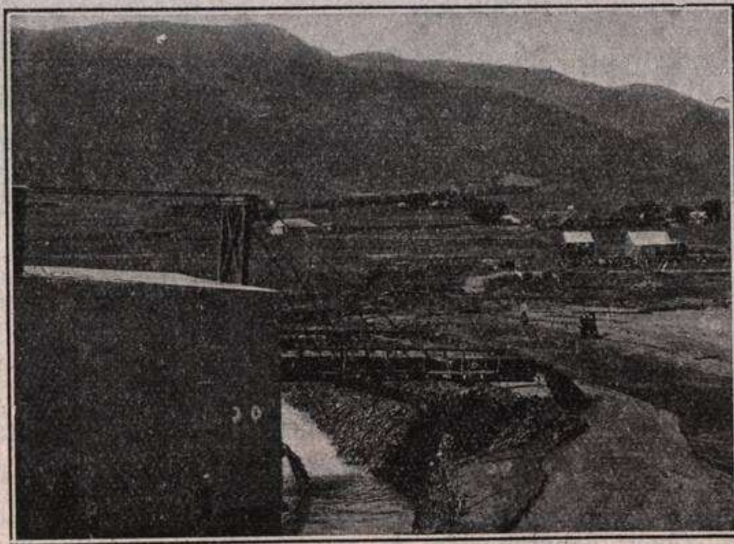
Fig. 198.—Draga-lavadero en los terrenos auríferos de Araluen (Nueva Gales del Sur-Australia). (Fot. comunicada por el profesor australiano Dr. O. Dalton).
