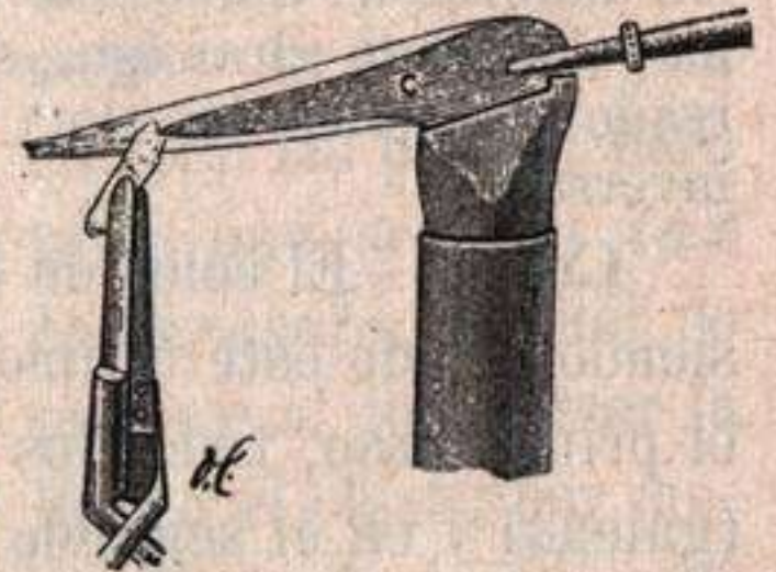
Fig. 169.—Pinzas de presión constante con puntas de platino. Fig. 170.—Ensayo de la fusibilidad. (De la obra Prácticas de Mineralogía y Geología , por J. Royo y O. Cendrero).
