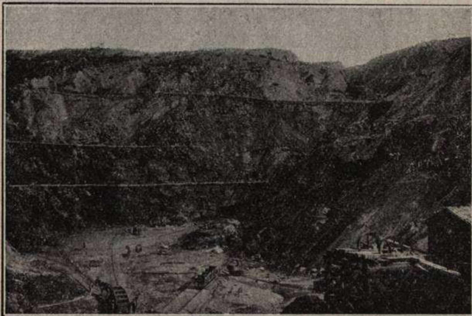
Fig. 215.—Otro aspecto de la explotación de una mina de Limonita en Setares (Castro Urdiales-Santander). (Fot. com. por el Dr. J. del Arco).
