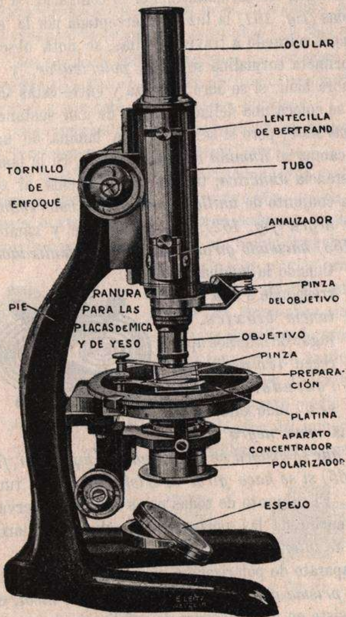
Fig. 167. — Microscopio polarizante o petrográfico de Leitz. (De la obra Prácticas de Mineralogía y Geología , por J. Royo y O. Cendrero).
