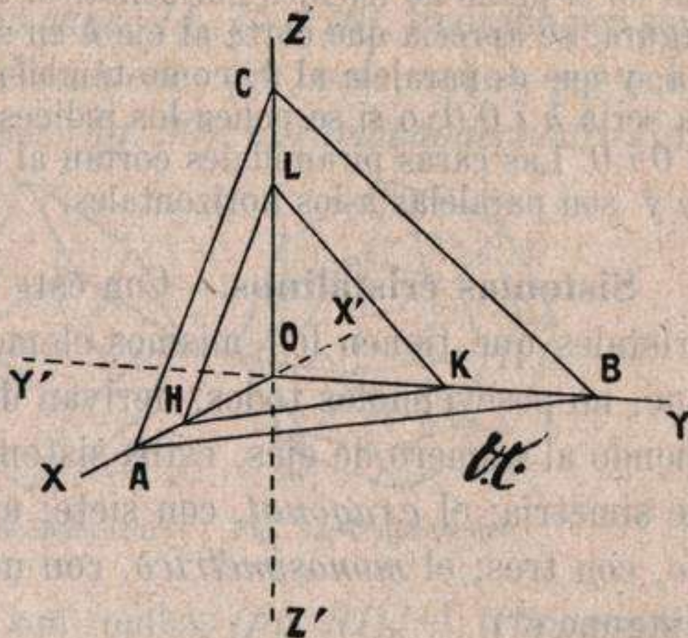
Fig. 88.—Notación de Miller.—A B C, cara unidad: H K L, cara cuyo símbolo se busca.
