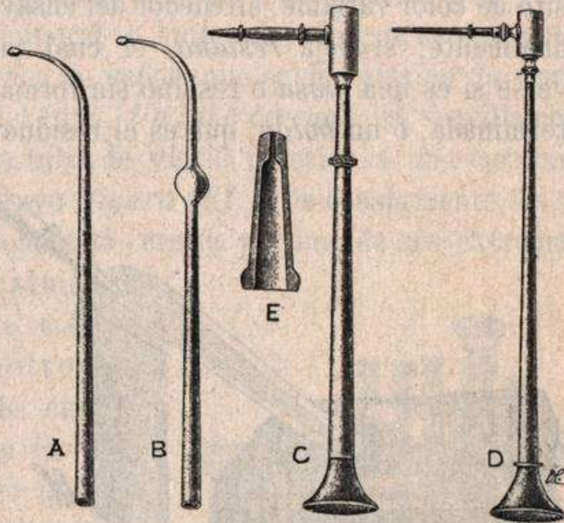
Fig. 175.—Varias clases de sopletes de boca.—A, de latón sin depósito; B, de latón con depósito; C y D, con depósito y punta de platino; E, punta de platino de C, aislada. (De la obra Prácticas de Mineralogía y Geología , por J. Royo y O. Cendrero).
