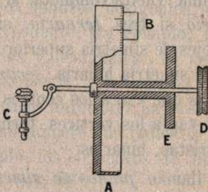
Fig. 73.—Goniómetro de reflexión de Wollaston y esquema explicativo. (De la obra Prácticas de Mineralogía y Geología , por J. Royo y O. Cendrero).
