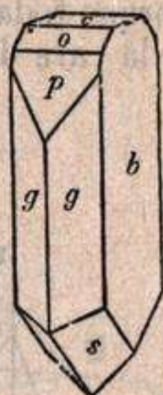
Fig. 82. Dos formas hemimórficas. (De Tschermak).
