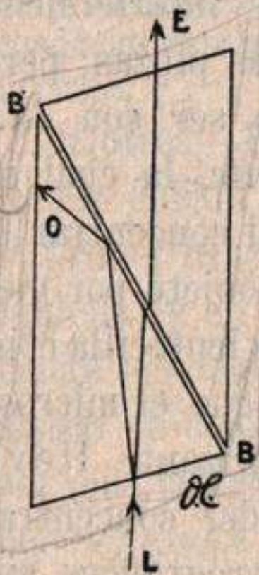
Fig. 166.—Sección de un Nicol con la trayectoria de los rayos de luz. (De la obra Prácticas de Mineralogía y Geología , por J. Royo y Orestes Cendrero).
