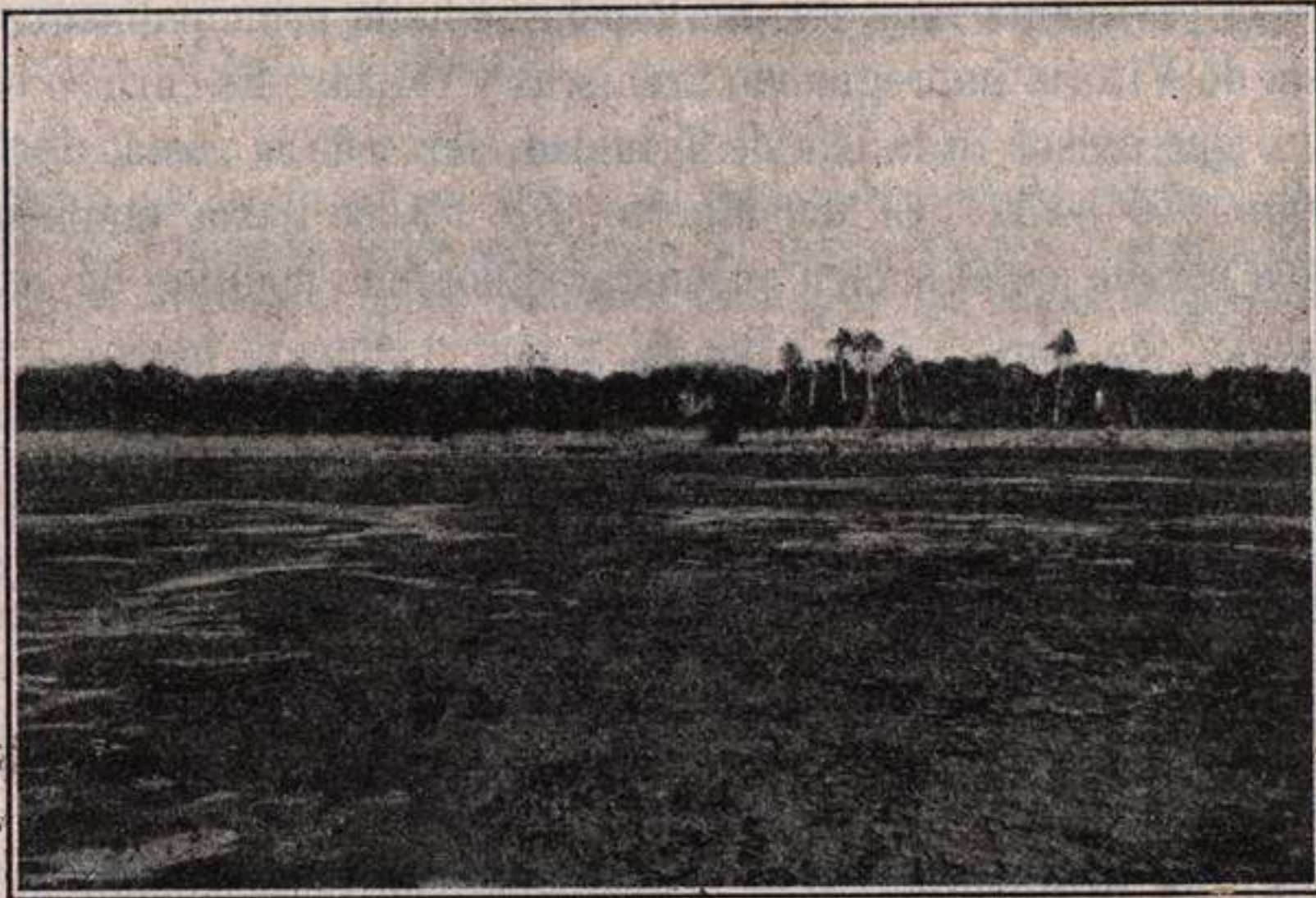
Fig. 250.—Lago de asfalto de la isla de Trinidad (costa de Venezuela): dicho lago es circular y mide unas 400 áreas de superficie. (Fot. com. por el profesor venezolano G. Delgado Palacios).
