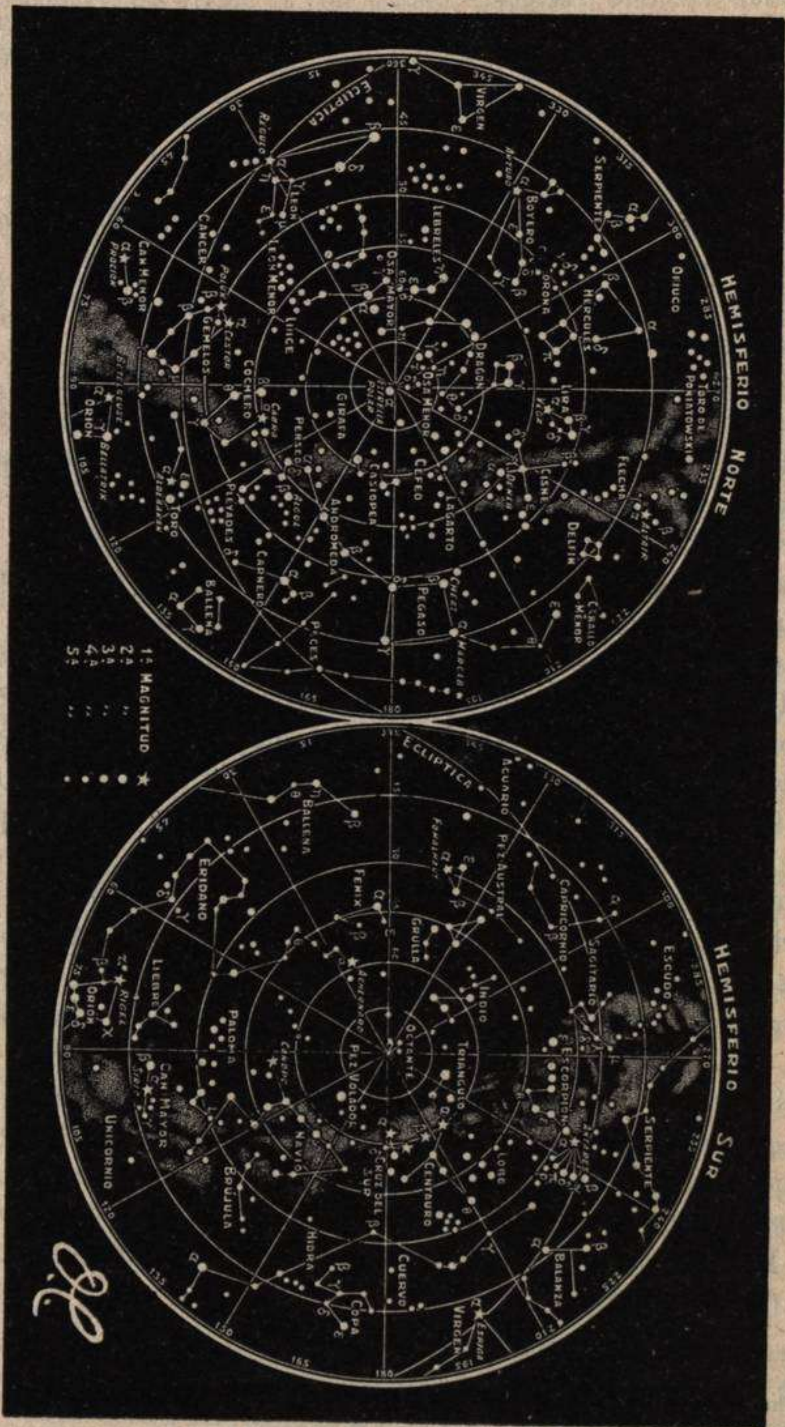
Fig. 10.—Esquema de un planisferio celeste con las principales constelaciones y las estrellas de las cinco primeras magnitudes. Los nombres de las constelaciones están escritos con letra mayor y vertical y los de algunas estrellas con letra menor e inclinada.
