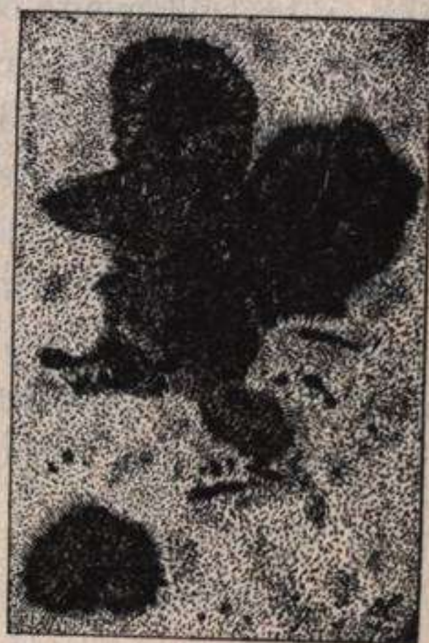
Fig. 13.—Manchas solares.
