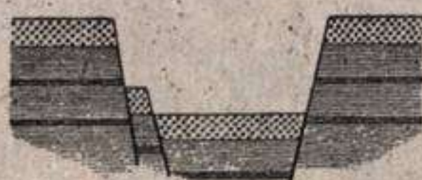
Fig. 392.—Fosa.
