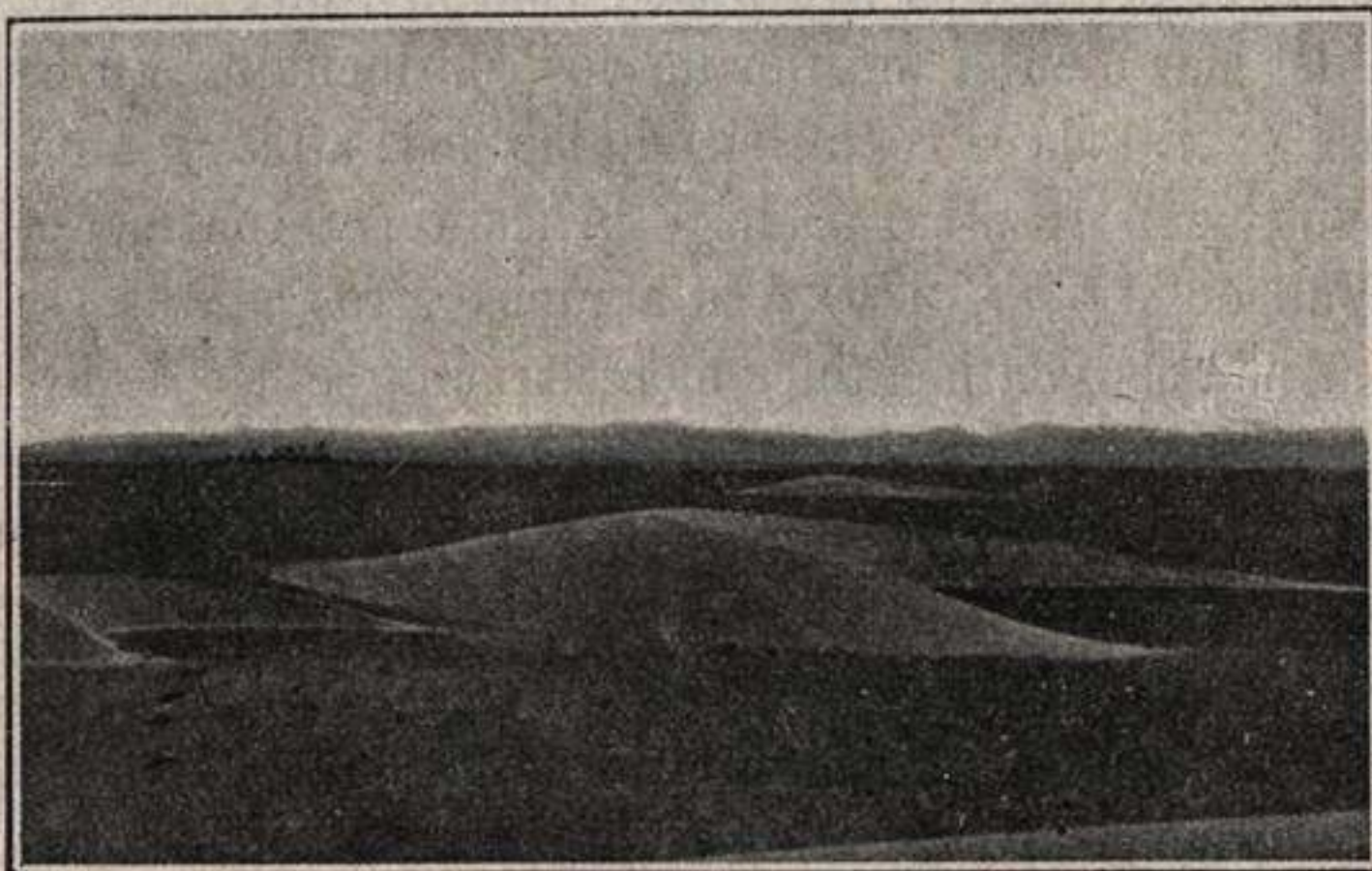
Fig. 273.—Dunas elementales de la Joya, entre Mollendo y Arequipa (Perú) (Fot. Dereims, en Haug).
