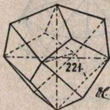
Fig. 98. Deltoedro.
