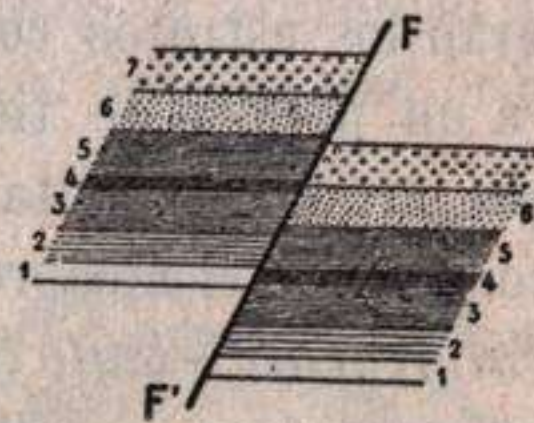
Fig. 387.—Falla inversa.
