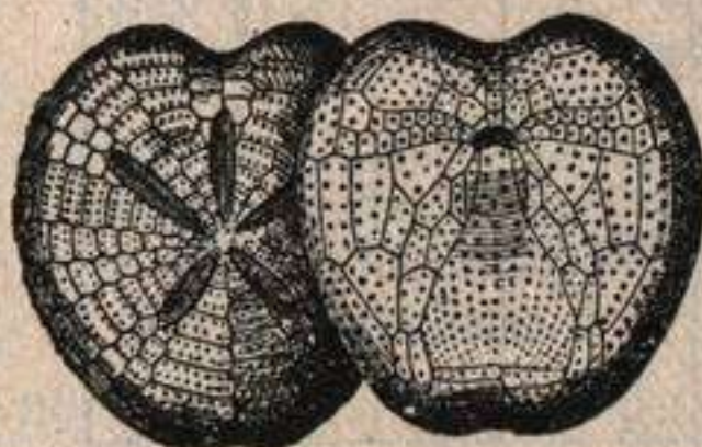
Fig. 524.— Micraster coranquinum ; erizo de mar del Cretácico.
