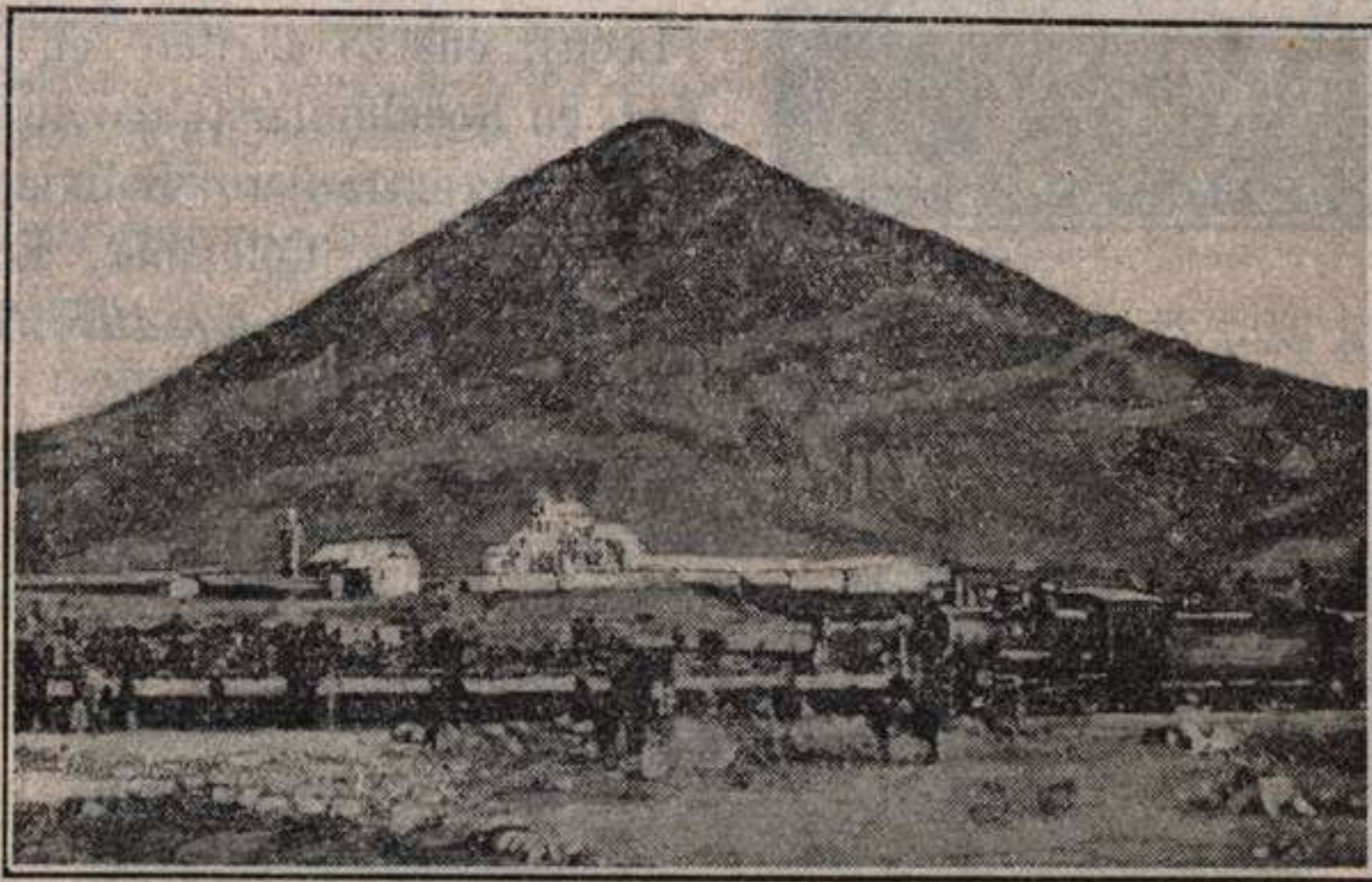
Fig. 196.—La célebre «Montaña de Plata» de Potosí (Bolivia), que se calcula ha producido, desde la conquista por los españoles, unos 900 millones de pesetas. En ella existe plata nativa asociada a otros minerales de plata. (Fot. comunicada por el profesor boliviano Dr. J. T. Oropeza).
