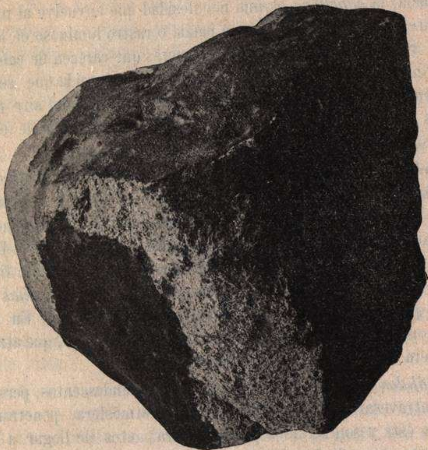
Fig. 30.—Meteorito (litito) caído en Olivenza (Badajoz) el 19 de julio de 1924. Trozo de 36 \frac{1}{2} kg. con superficies frescas y costra fundida. (Fot. F. Navarro).
