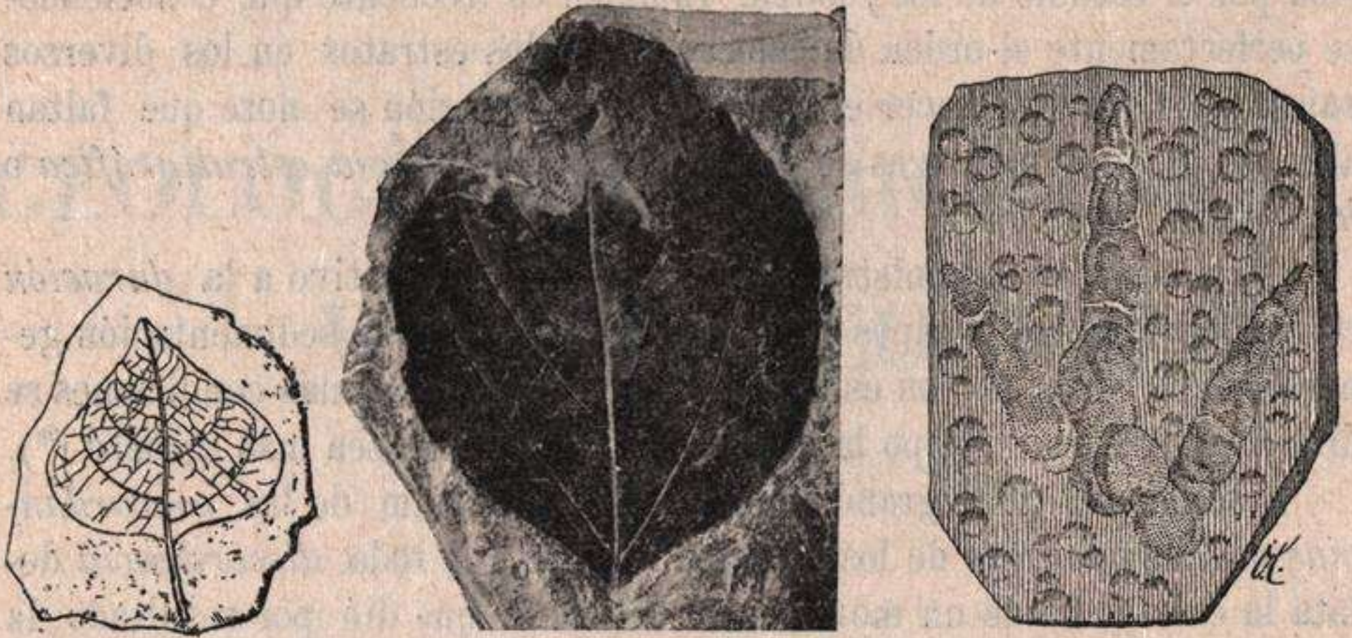
Fig. 466.—Impresión de una hoja de chopo en una caliza: su longitud nueve centímetros.
