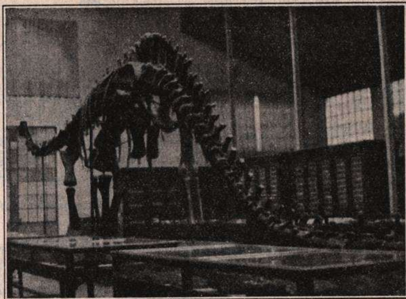
Fig. 520.—Esqueleto de Diplodóccus , Reptil saltador del Jurásico: longitud, 25 metros. Está visto por su parte posterior para que se pueda apreciar el gran desarrollo de la cola y extremidades posteriores. (Ejemplar del Museo Nacional de Ciencias Naturales).—(Fot. O. Cendrero).
