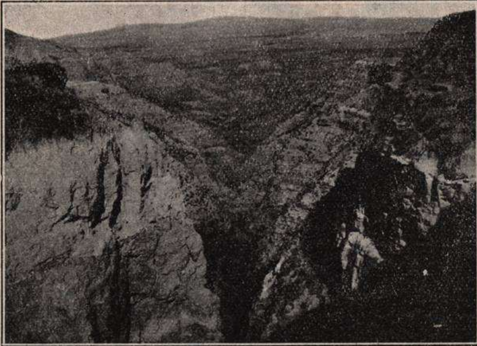
Fig. 299.—El Barranco de los Mártires, en Alcalá de Henares (Madrid). (Fot. O. Cendrero).
