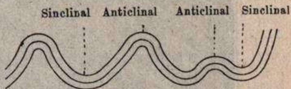
Fig. 373.—Pliegues diclinales.
