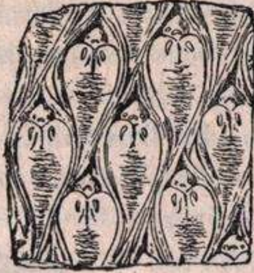
Fig. 494.—Trozo de un tronco de Lepidodendron , Licopodinea del Devónico y Carbonífero
