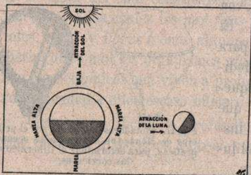
Fig. 45.—Explicación de las mareas: marea muerta.
