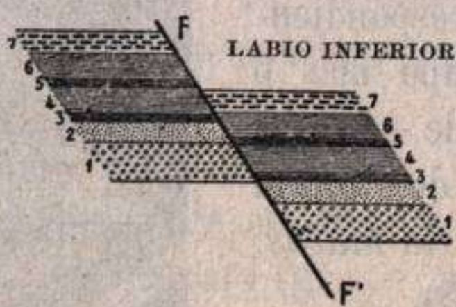
Fig. 386.—Falla normal. FF' plano de falla. (De Haug).
