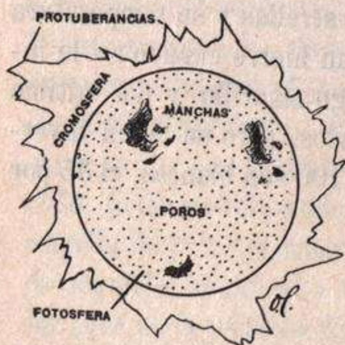
Fig. 12.—Conjunto esquemático del Sol.
