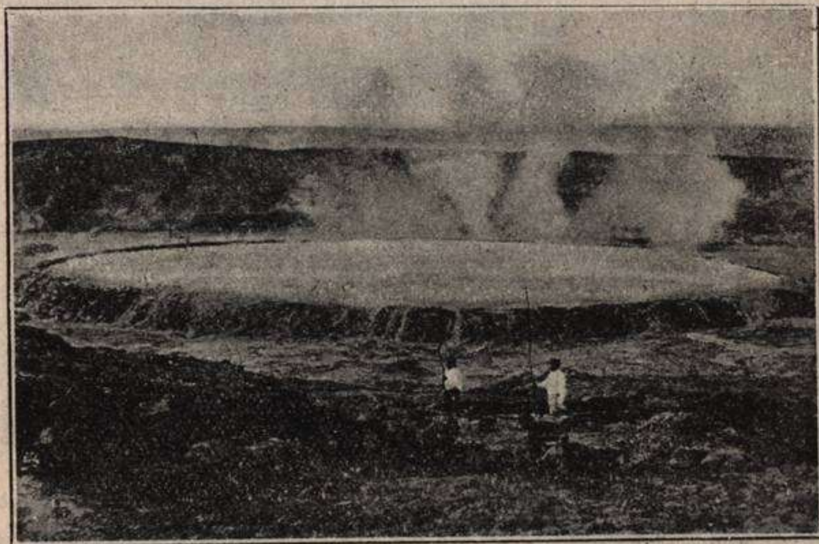
Fig. 401.—Cráter del volcán Kilauea. En realidad, el cráter primitivo del Kilauea es enorme, pues su circunferencia mide unos 12 kilómetros; pero hace ya tiempo que no está todo él en actividad, sino que ésta se limita a una o más regiones o cráteres secundarios, como el que representa esta figura que reproduce el estado del cráter en 1893. Al fondo se ve la pared del cráter primitivo. (Fot. F. G. T. Silva).
