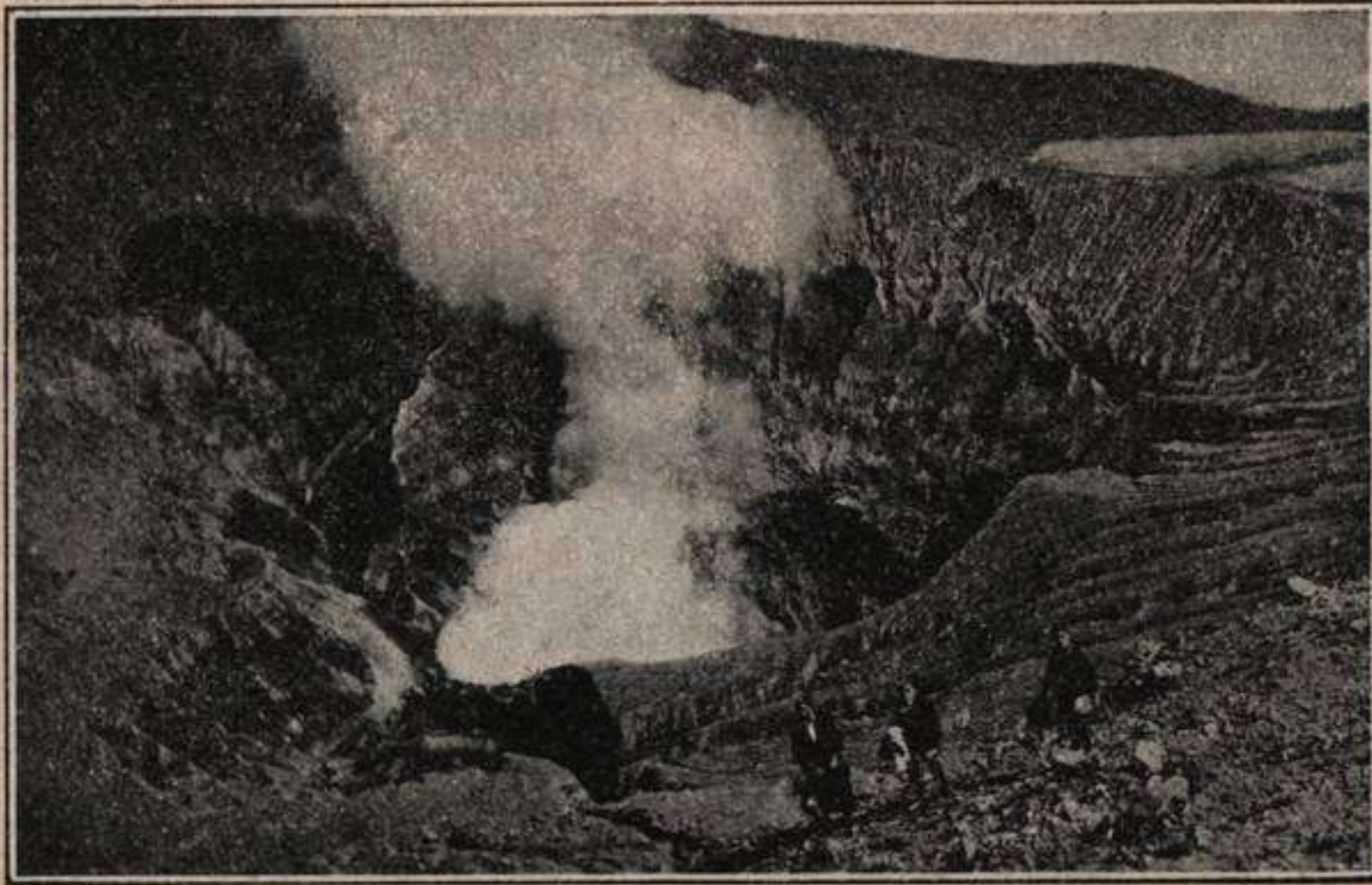
Fig. 414.—Cráter del Volcán Irazú (Costa Rica) en su continua fase de fumarola. (Fot. com. por el prof. costarricense Dr. Manuel Valerio).
