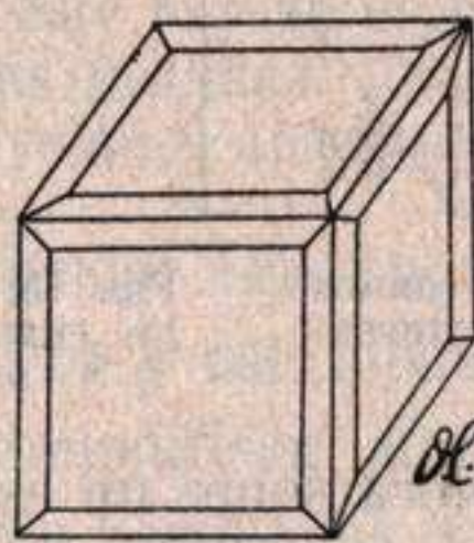
Fig. 80.—Cubo biselado.
