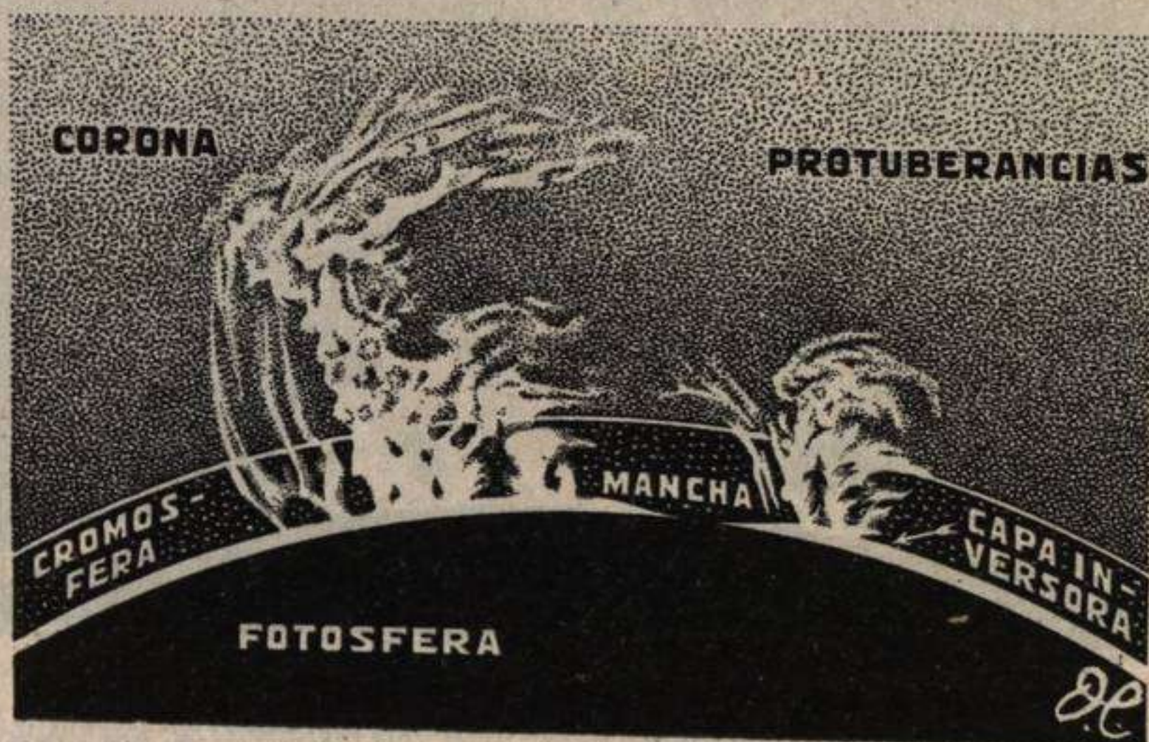
Fig. 14.—Esquema de la estructura del Sol.
