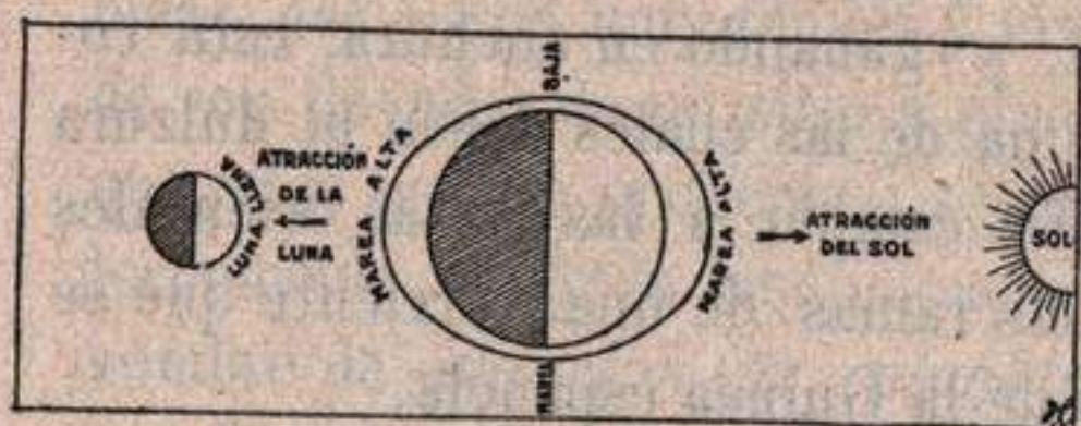
Fig. 43 Explicación de las mareas: marea viva.
