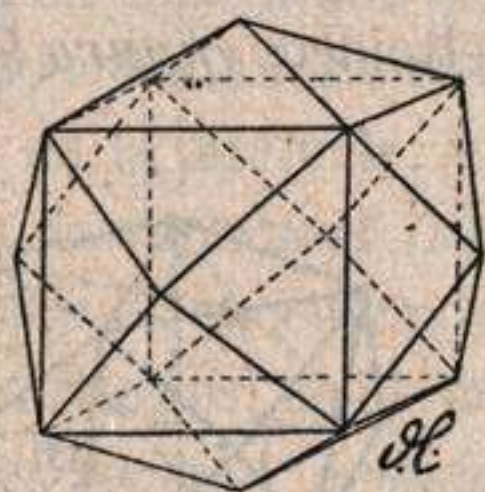
Fig. 93. Tetraquisexaedro.
