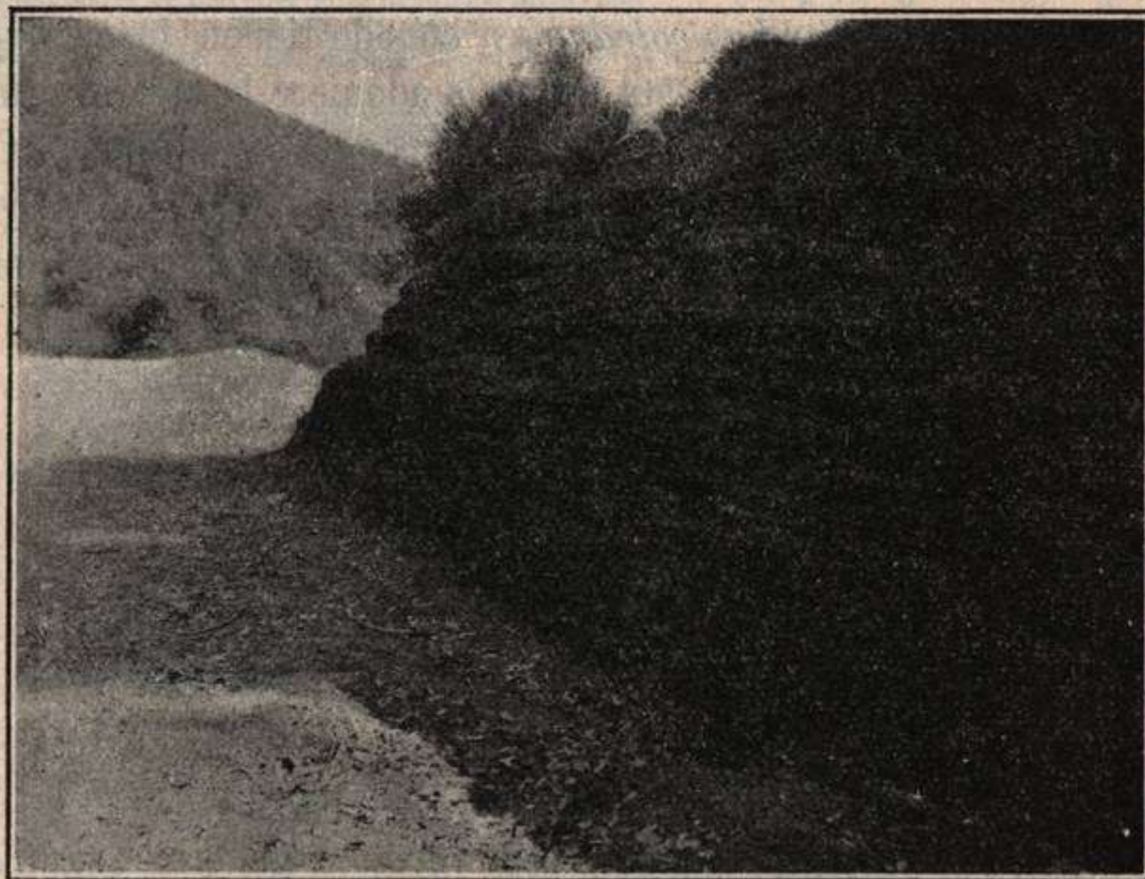
Fig. 438.—Tobas volcánicas del volcán de Santa Margarita (Olot-Gerona) (Fot. com. por el prof. Modesto Bargalló).
