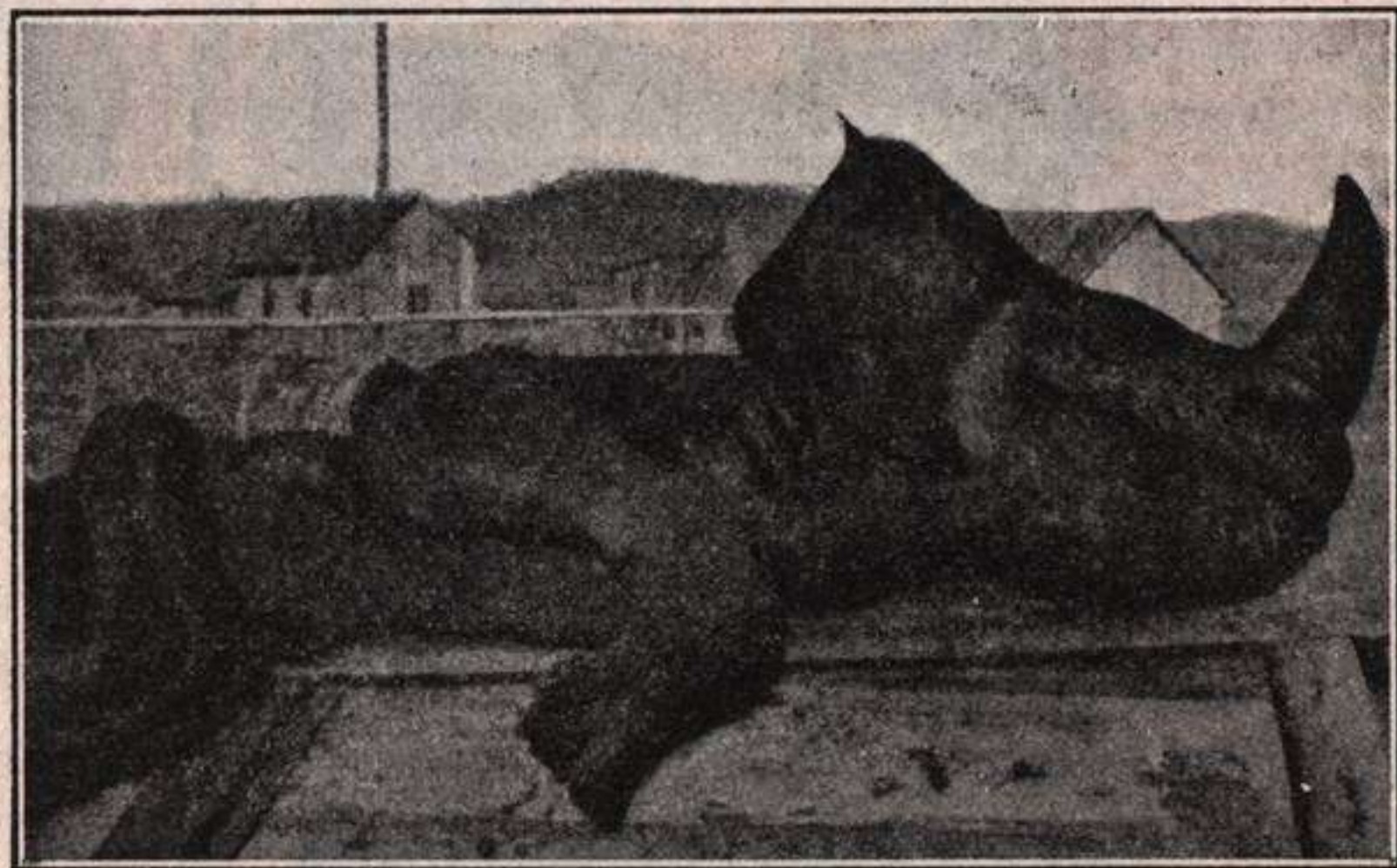
Fig. 473.—Rinoceronte extraído de un yacimiento petrolífero de Starunj (Galitzia-Austria). De la obra del Dr. H. Obermaier, Der Mensch der Vorzeit .
