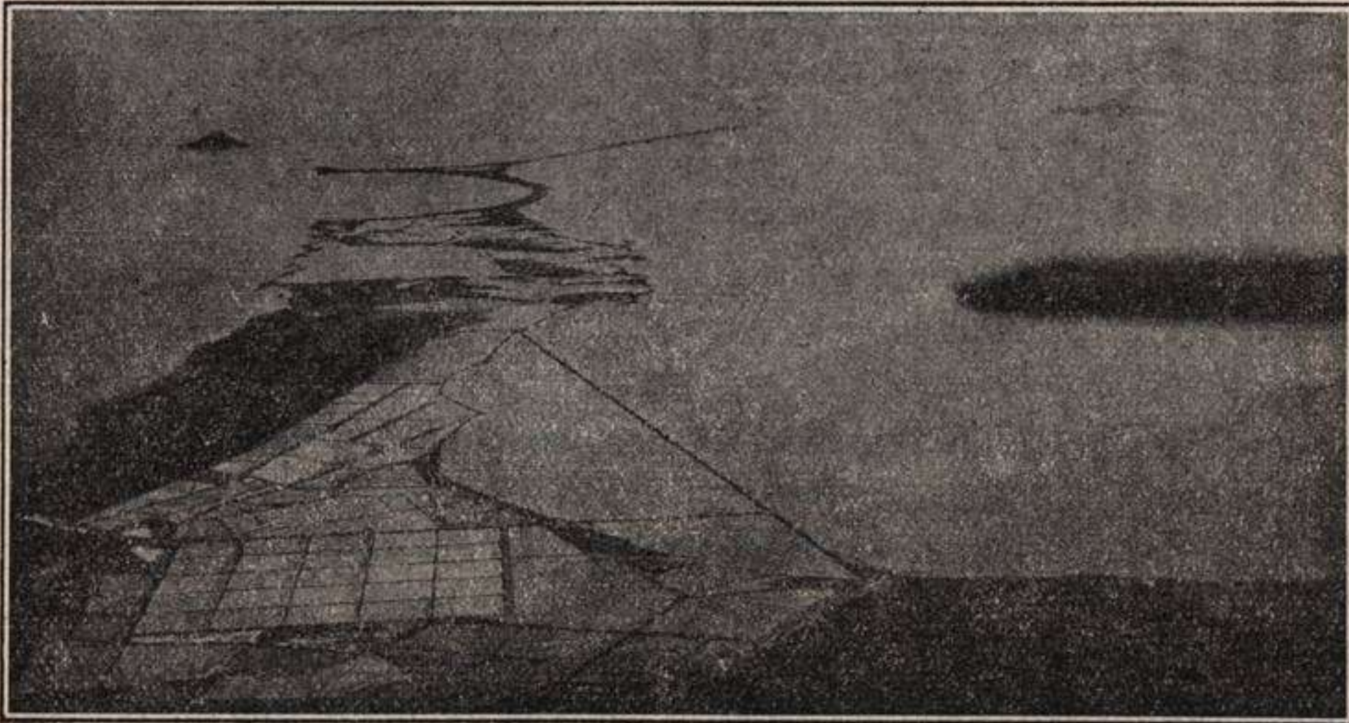
Fig. 327.—Vista general del cordón litoral que separa el Mediterráneo (a la izquierda) y el Mar Menor (Murcia). En primer término izquierda las Salinas de San Pedro de Pinatar. (Fot. Aviación Española, comunicada por el profesor J. Páez Ríos).
