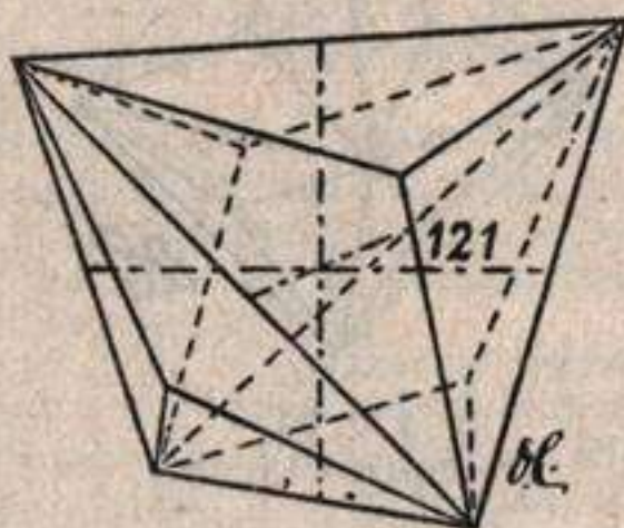
Fig. 99. Triaquistetraedro.
