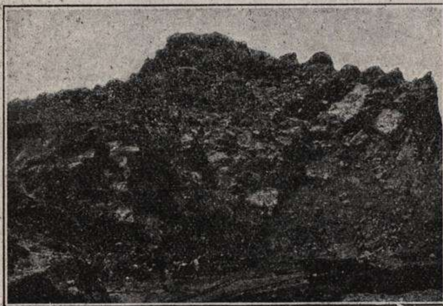
Fig. 241:—Crestones de oligisto y magnetita en el Monte Uisan. (Melilla-Africa).
