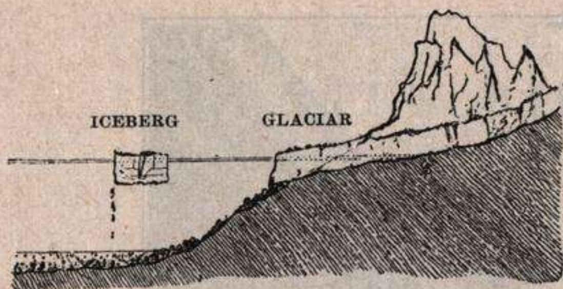
Fig. 349.—Esquema de la formación de los icebergs. (De Geikie).
