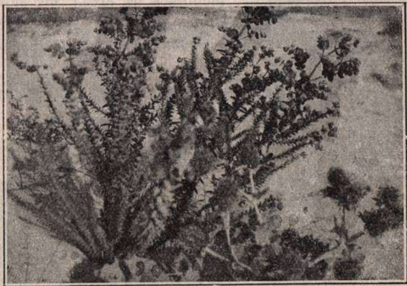
Fig. 283.—Otras plantas ( Eryngium , la menor y Euphorbia , la ª mayor) que contribuyen a la fijación espontánea de las dunas vivas. (Fot. O. Cendrero).
