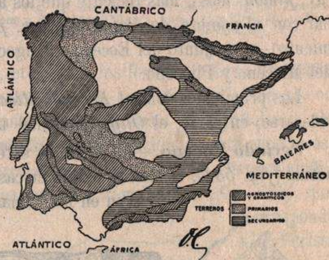
Fig. 530.—Esquema de la distribución de las tierras y de los mares en la Península Ibérica al terminar la Era Secundaria.
