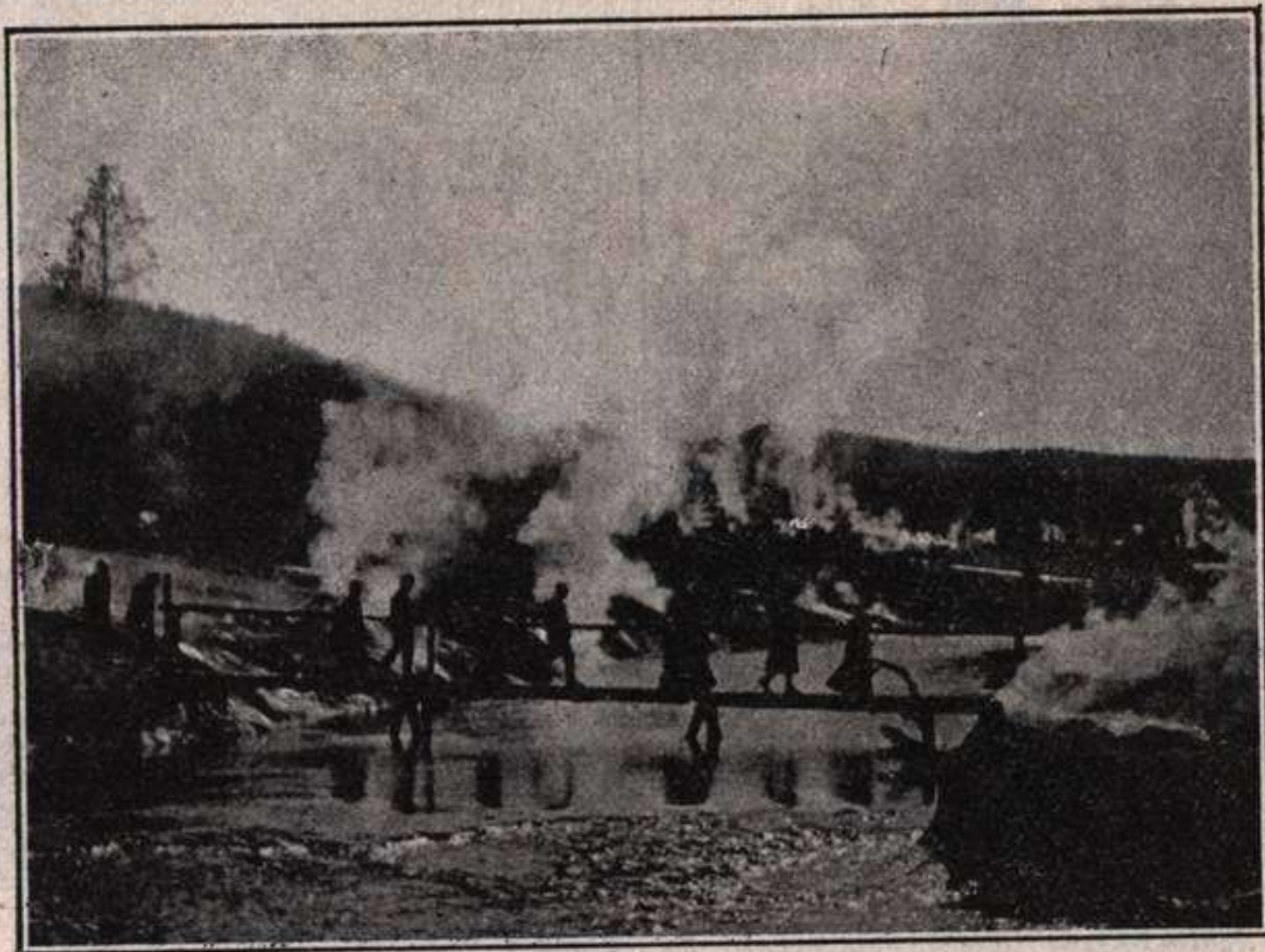
Fig. 421.—Vista parcial del Parque de Yellowstone (EE. UU. de N. América) que sólo da una remota idea de la belleza de esta región donde existen en total unos setecientos orificios de solfataras, fumarolas, fuentes termales, geiseres, etc. (Fot. comunicada por el prof. C. Ordóñez C. M.)
