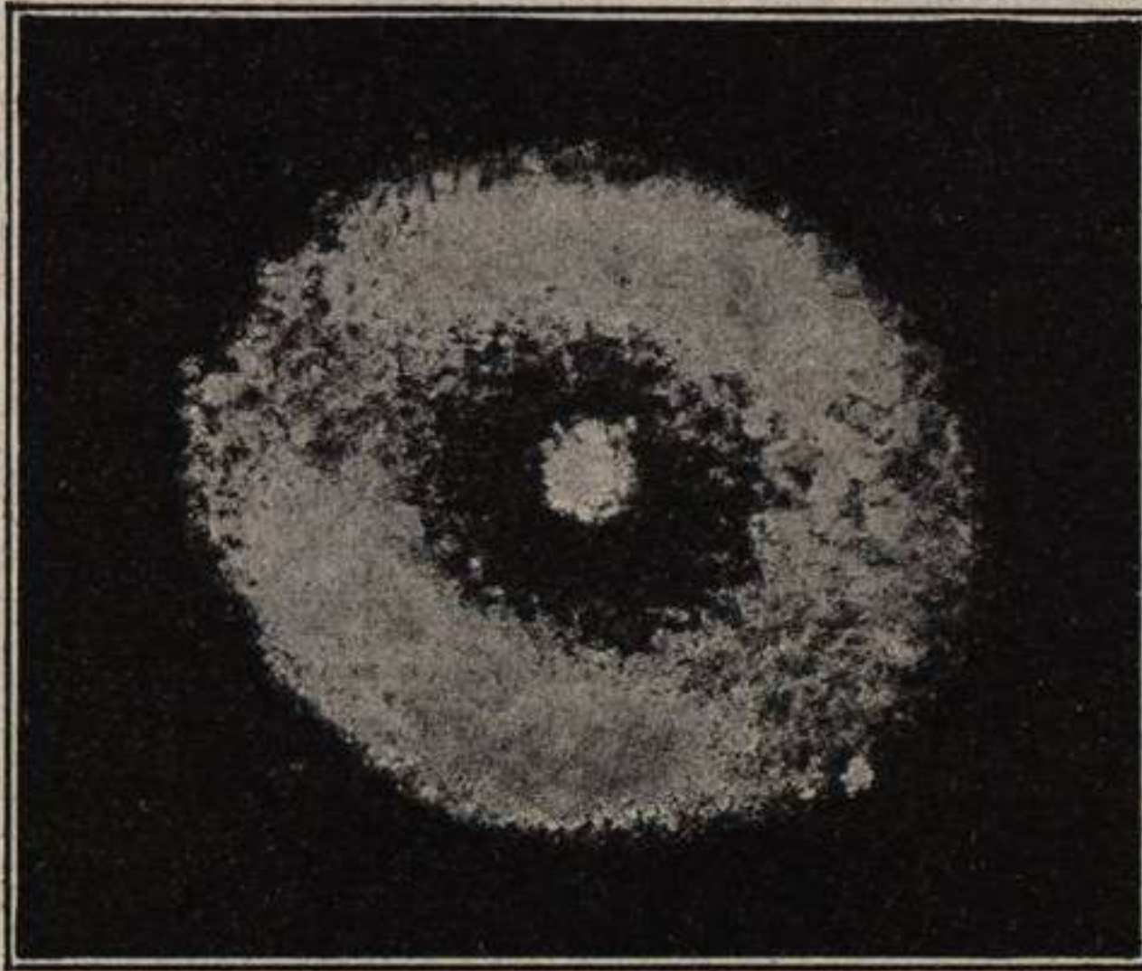
Fig. 7.—Nebulosa anular de Lira. (Fot. Montangerand en el Observatorio de Toulouse, con una exposición de 9 horas).
