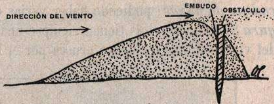
Fig. 272.—Esquema de la formación de una duna.
