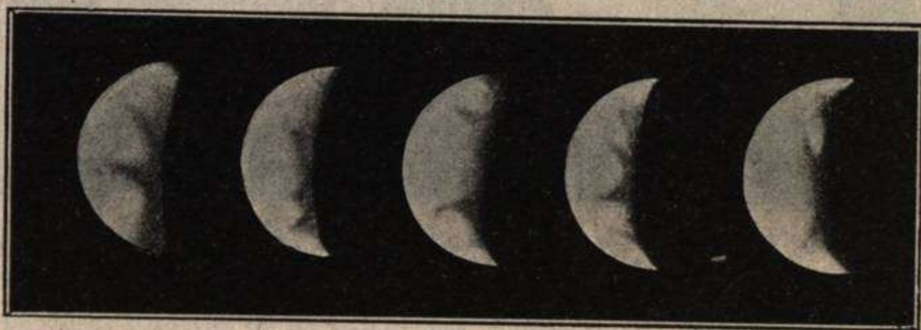
Fig. 18.—Diversos aspectos de Mercurio. (Según G. y V. Fournier).
