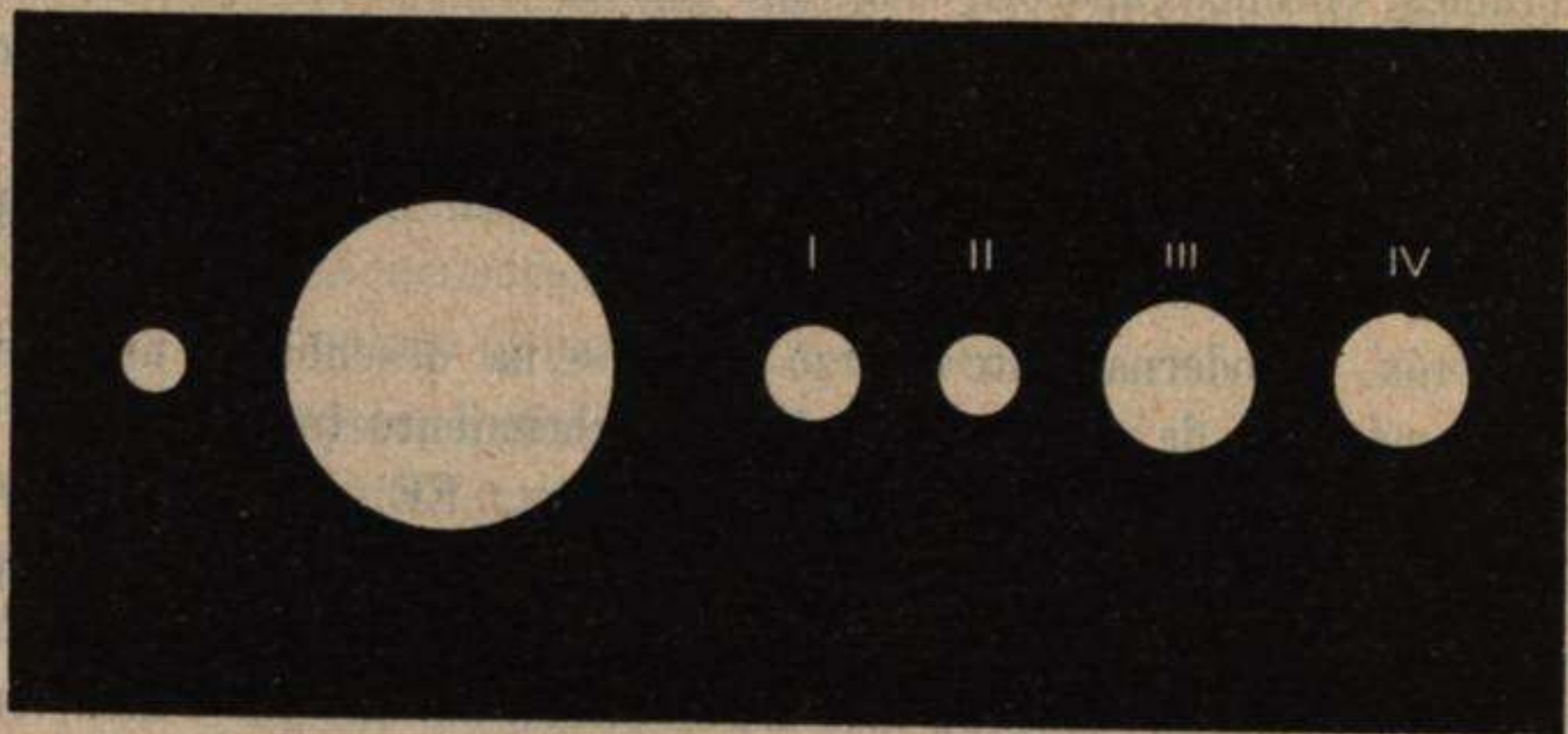
Fig. 27.—A la izquierda la Luna y la Tierra.—De I a IV los cuatro satélites de Júpiter que son mayores que la Luna.
