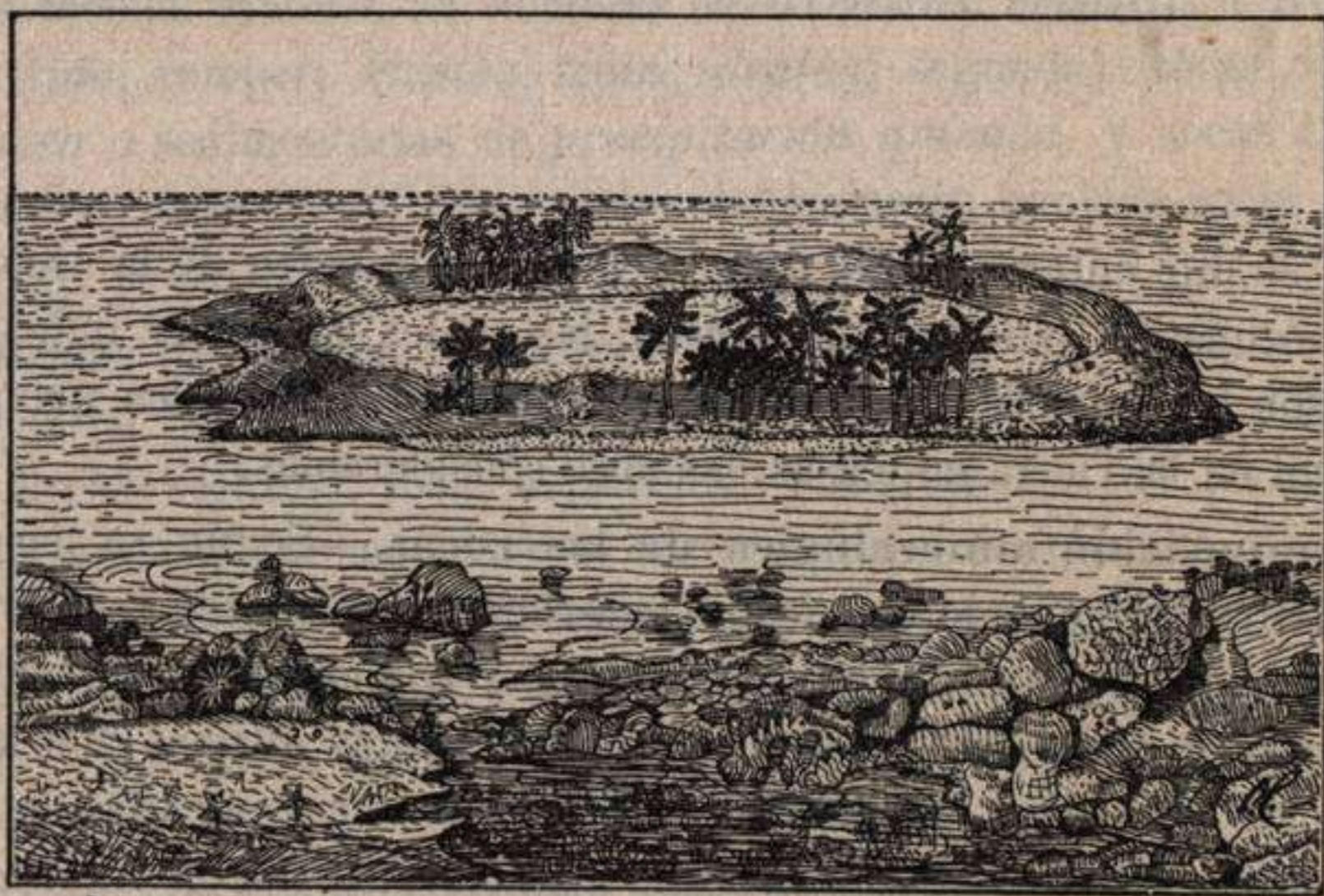
Fig. 364.—Conjunto esquemático de un atoll y de parte de un arrecife de coral.
