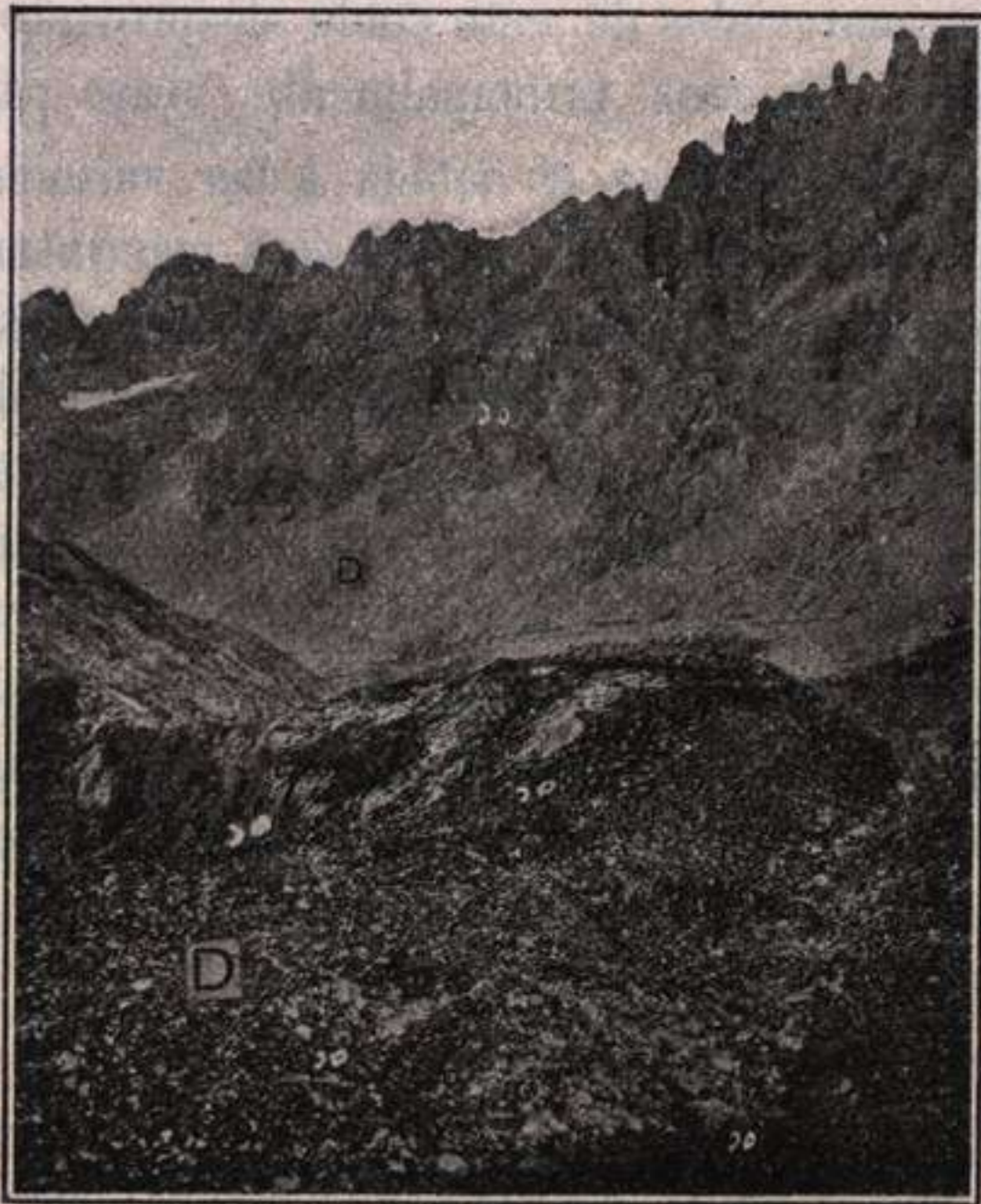
Fig. 257.—Pedrizas o pedregales en Picos o Peñas de Europa (Santander-Asturias). En las vertientes de las montañas elevadas se encuentran muchos detritos de tamaño variable ( D en la figura) debidos a la descomposición atmosférica, o acción destructora de la atmósfera, y a la acción del hielo. (Fot. comunicada por el profesor J. Fresnedo).
