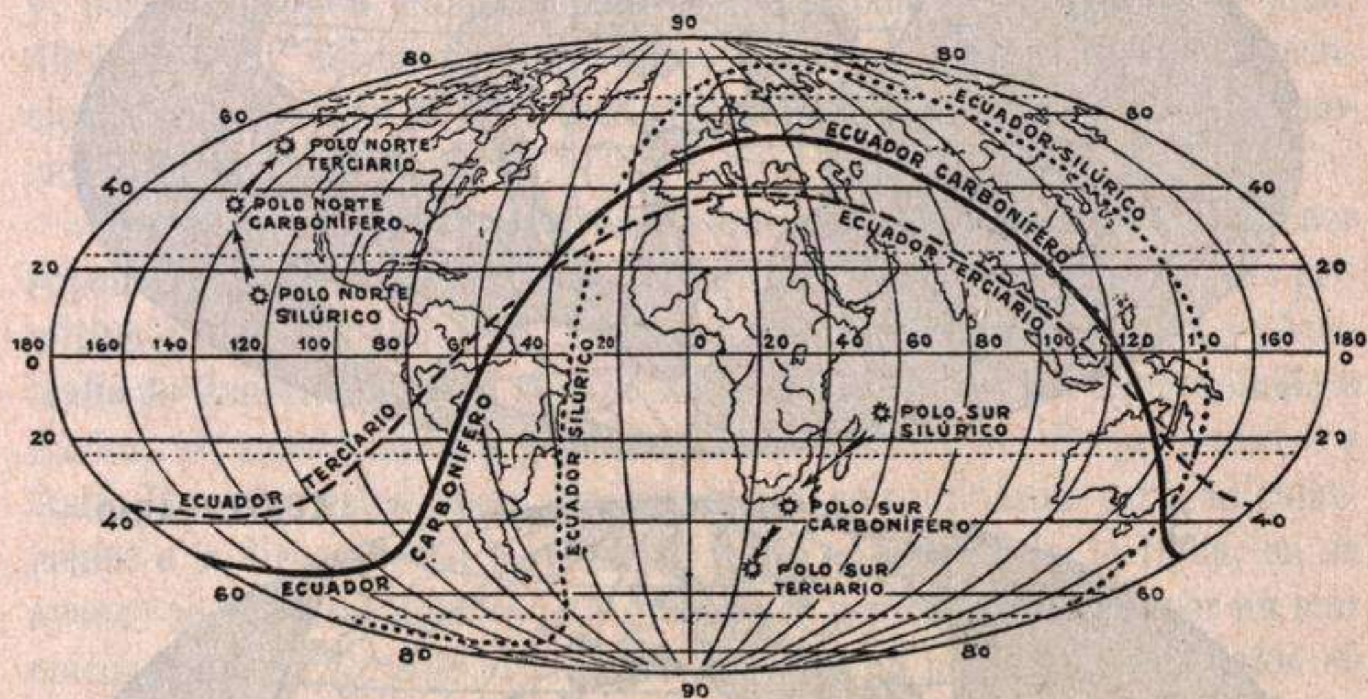
Fig. 447.—Planisferio terrestre con la posición del ecuador y los polos en algunos periodos geológicos. Las flechas indican la dirección del movimiento de los polos del Silúrico al Terciario. (Inspirado en Kreichgauer).
