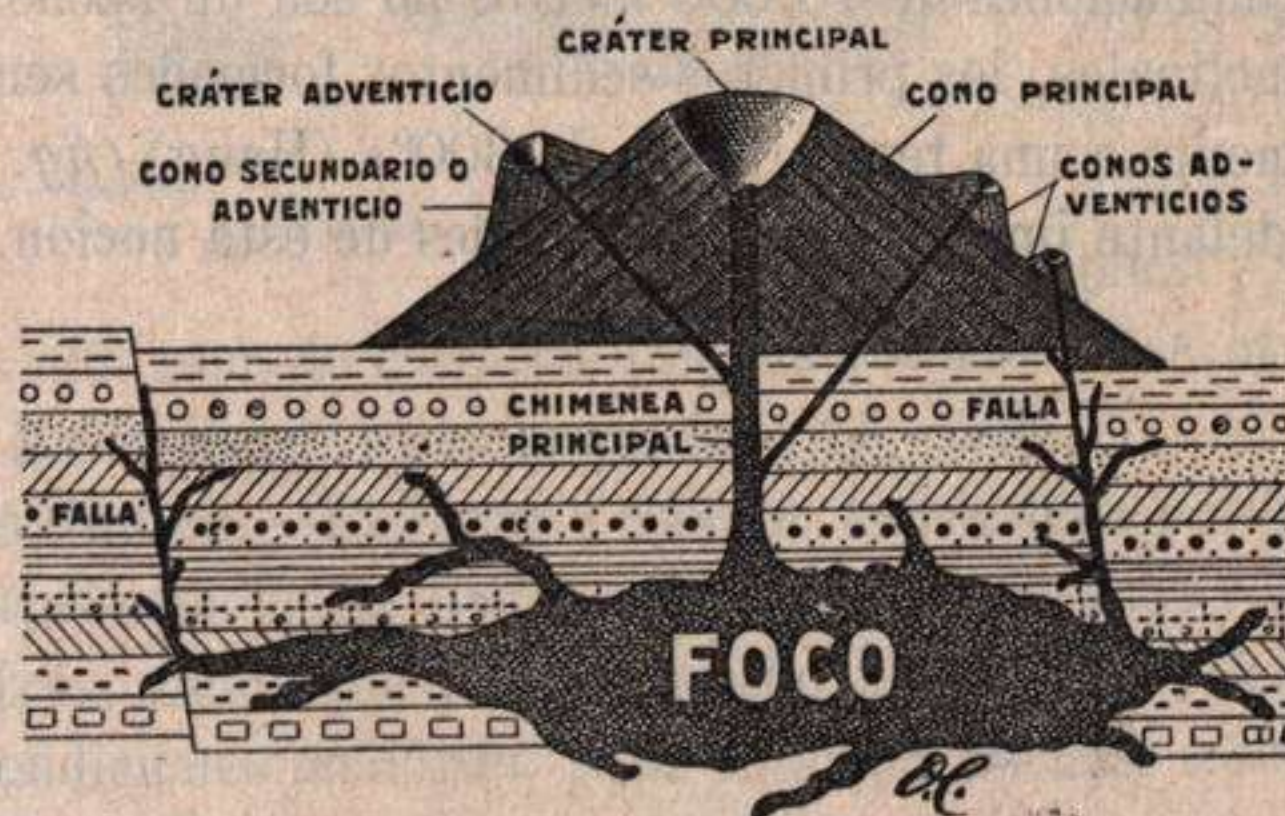
Fig. 395.—Esquema de un volcán.
