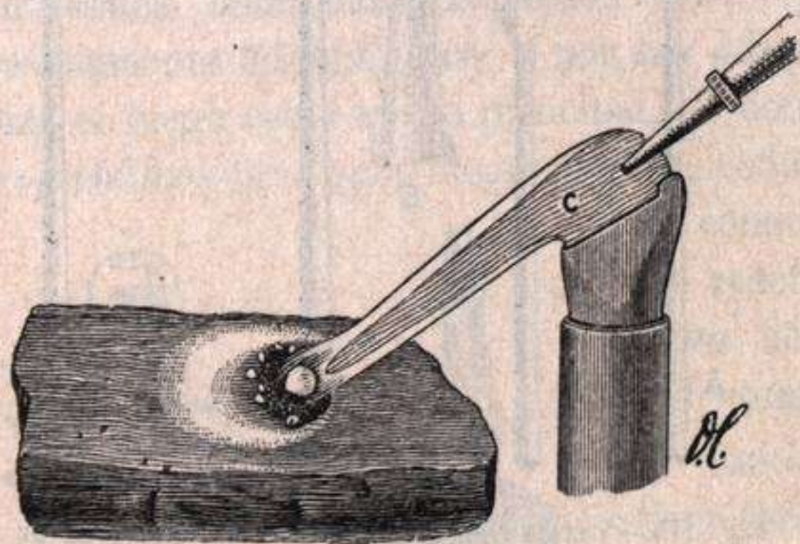
Fig. 178.—Obtención de botones y aureolas en los ensayos al carbón. (De la obra Prácticas de Mineralogía y Geología , por J. Royo y O. Cendrero).
