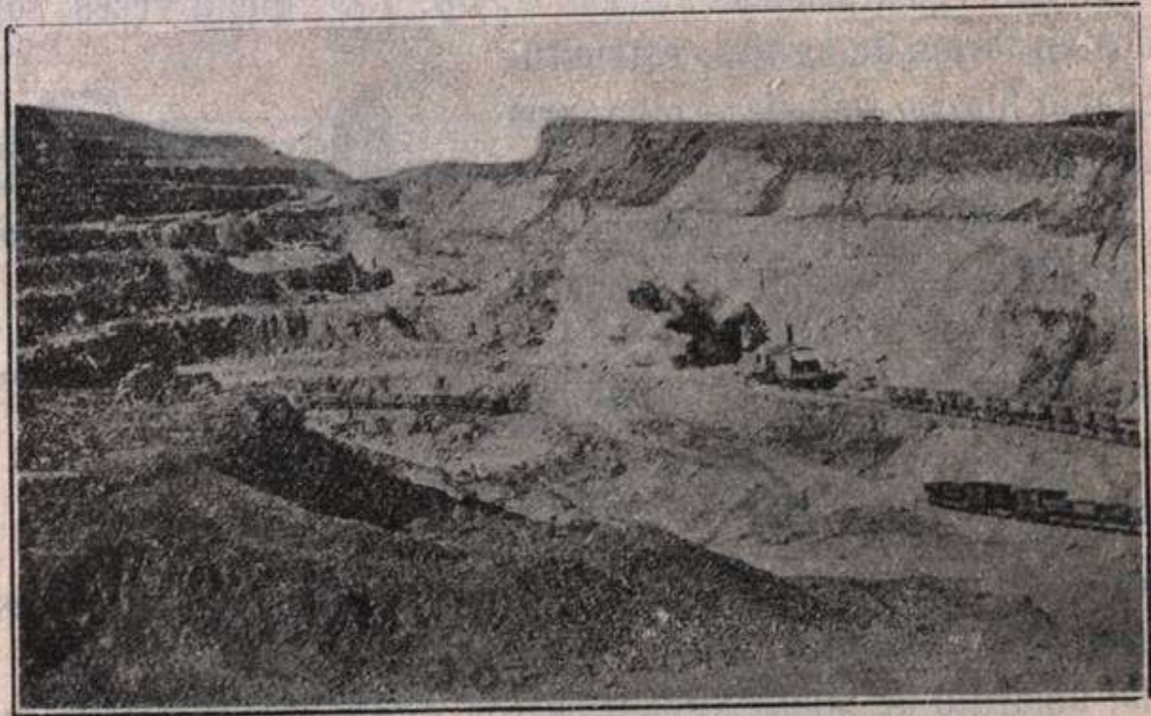
Fig. 200.—Minas de pirita y de calcopirita de Riotinto (Huelva).—Canteras en el mismo mineral en el sitio llamado La Dehesa. (Fot. comunicada por el profesor doctor M. San Miguel).
