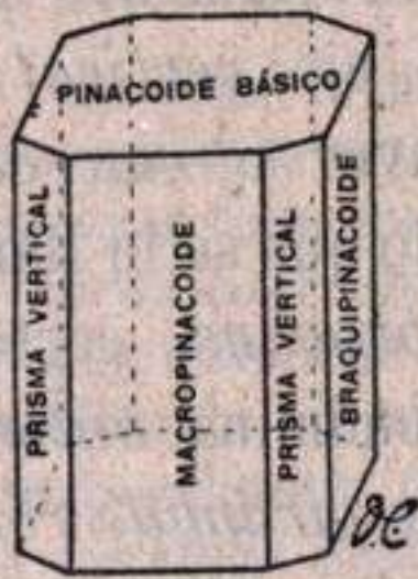
Fig. 112.-Forma compuesta de pinacoides y prisma vertical.
