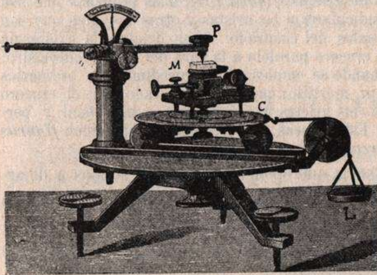
Fig. 152.—Esclerómetro.
