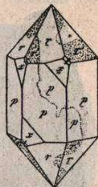
Fig. 131. Dos maclas de intrusión del cuarzo. (Tschermak, Sansoni).
