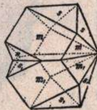
Fig. 127.—Macla de contacto de la casiterita. (Tschermak).
