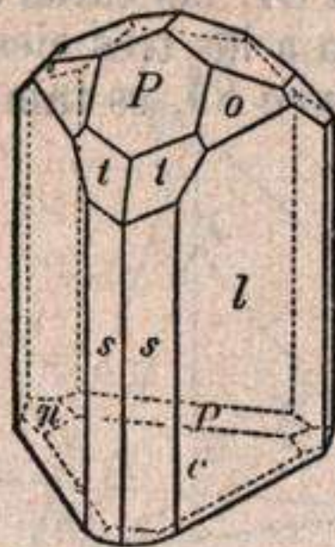
Fig. 82. Dos formas hemimórficas. (De Tschermak).
