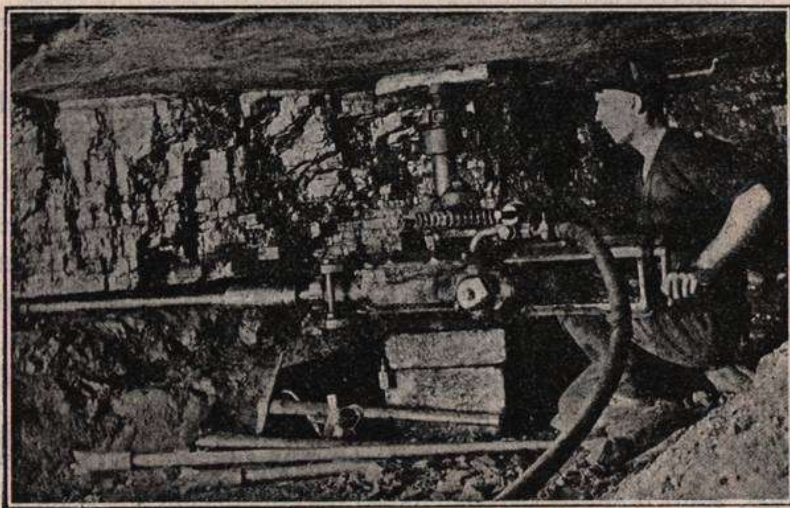
Fig. 254.—Interior de una mina de hulla: rompiendo las capas del carbón por medio de una percusora eléctrica. (Fot. comunicada por M. de Pintés).
