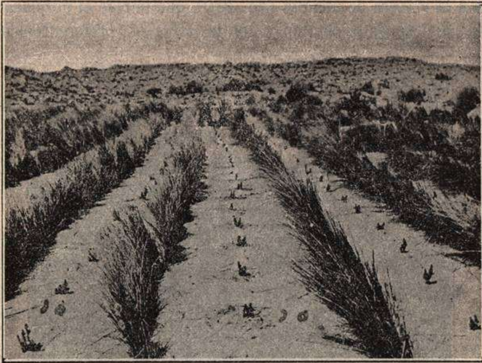
Fig. 279.—Fijación de la duna litoral de Guardamar (Alicante) con plantaciones de barrón ( Psamma ): entre ellas, pinos de un año. (Fot. ing. F. Mira, comunicada por el profesor P. M. Vigo, S. J.)
