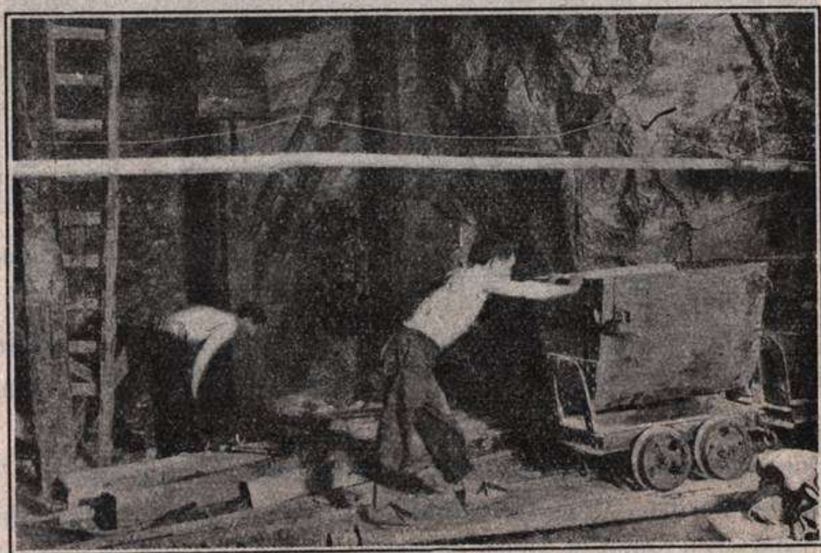
Fig. 204.—Interior de una mina de Pirargirita en Hiendelaencina (Guadalajara).
