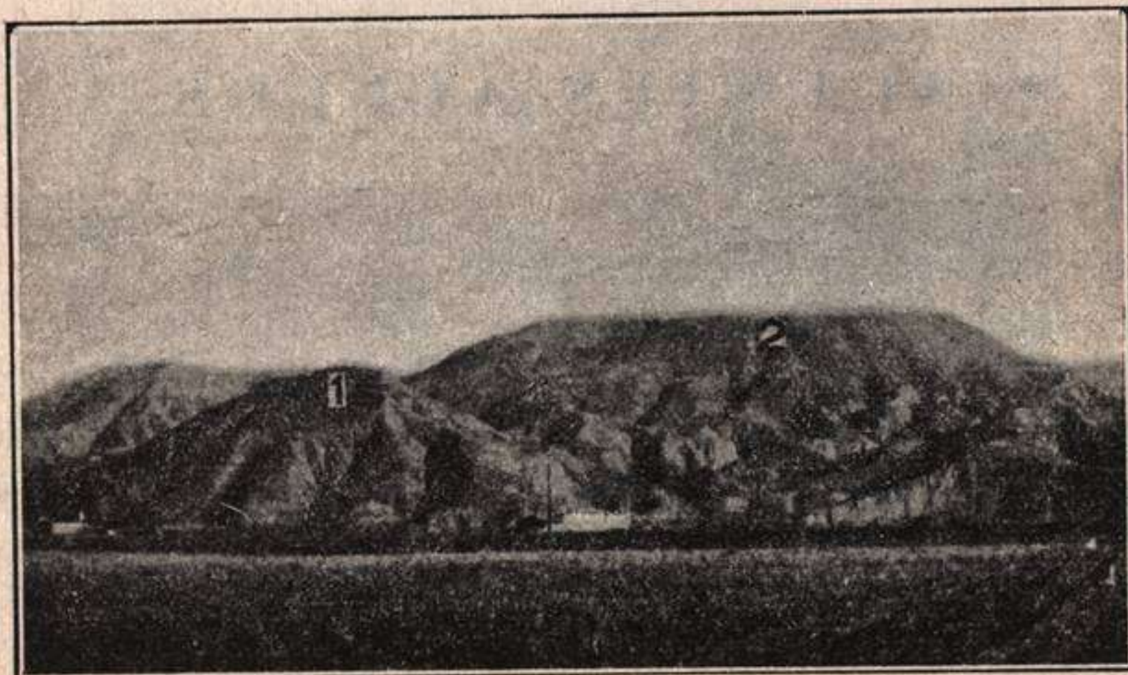
Fig. 284.—Barrancos o zanjas formados por efecto de la erosión y denudación de las aguas salvajes en los terrenos blandos del Cerro del Conde (1) y del Écce-Homo (2) en Alcalá de Henares (Madrid). (Fot. O. Cendrero).
