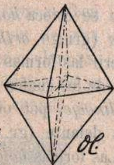
Fig. 109.—Pirámide rómbica.
