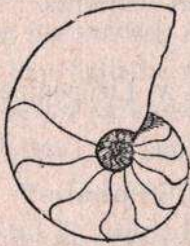
Fig. 496.— Clymènia , Ammonitido propio del Devónico.
