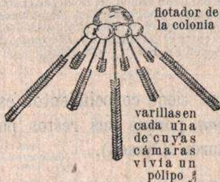
Eig. 486.— Graptolites restaurado.
