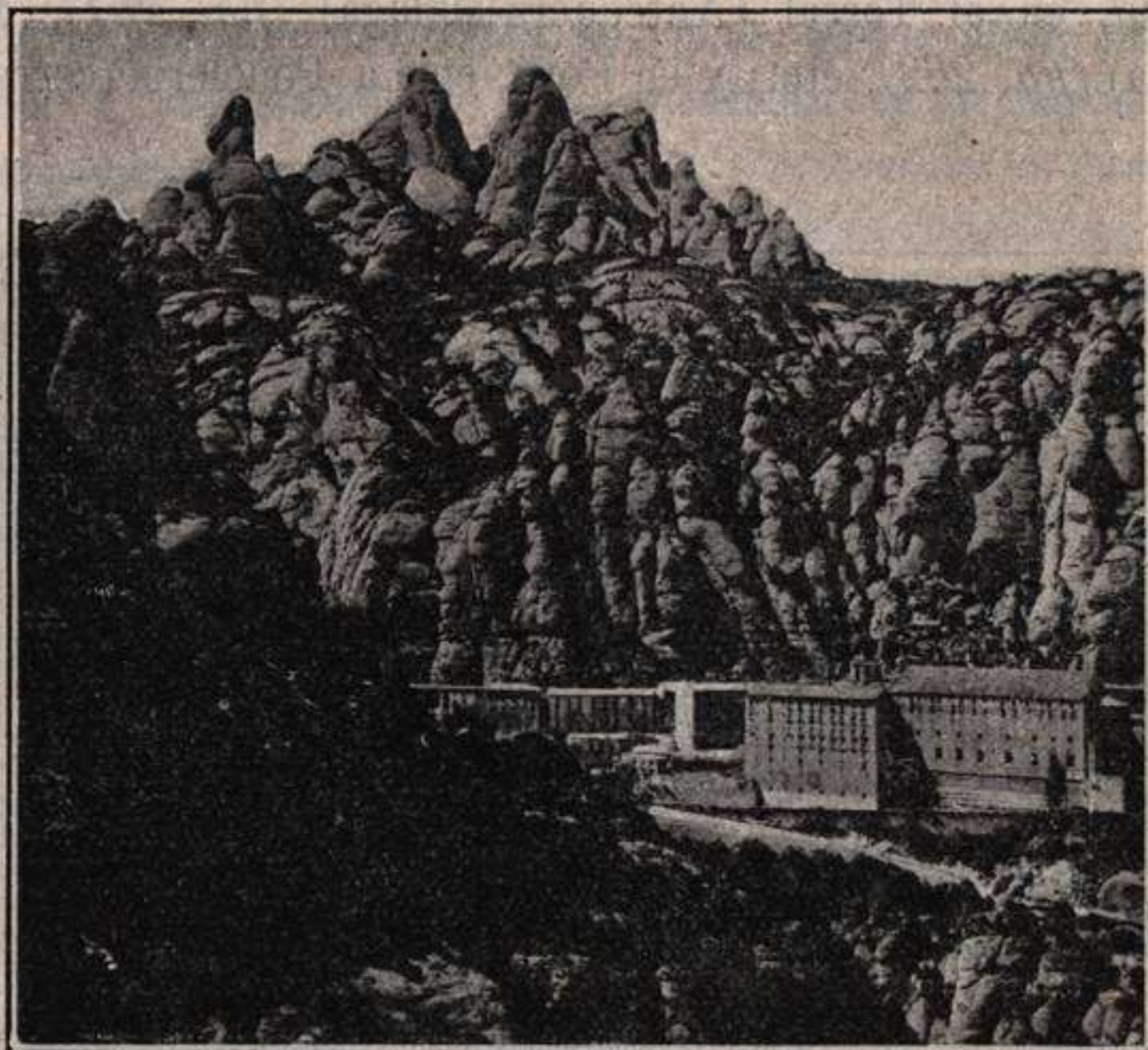
Fig. 262.—Topografía ruiforme-monserratina. (Fot. comunicada por el profesor Dr. M. San Miguel de la Cámara).
