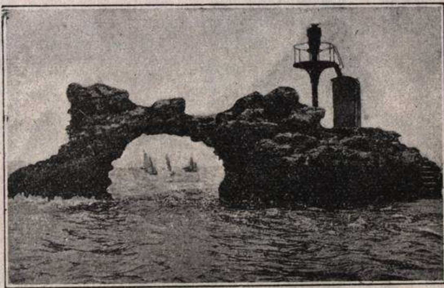
Fig. 322.—«Peña Horadada», a la entrada de la bahía de Santander, como ejemplo de arco natural debido a la acción erosiva del mar. (Fot. O. Cendrero).
