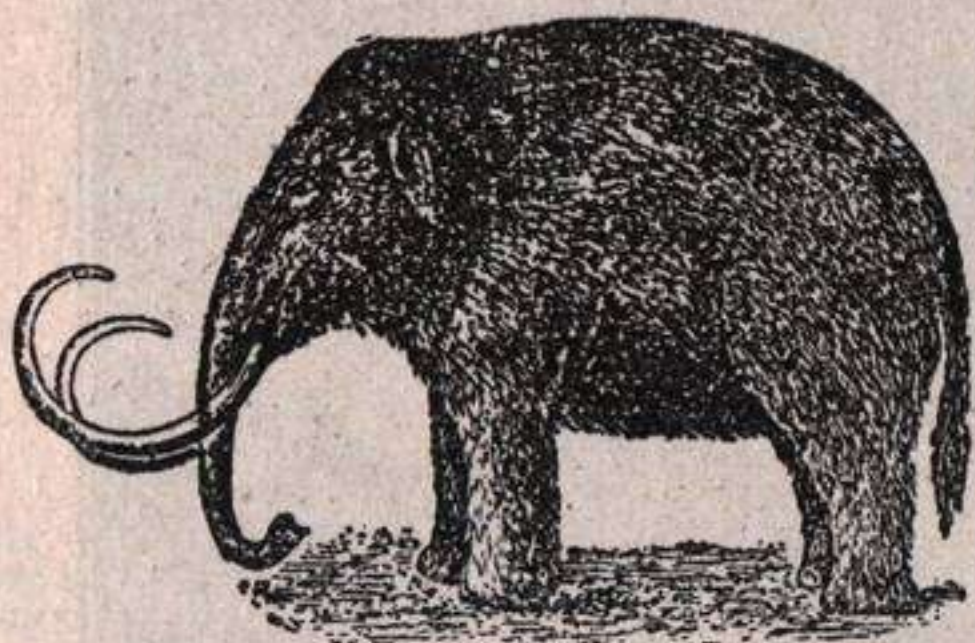
Fig. 472.—Mamut o elefante lanudo ( Élephas primigenius ): su altura 4 a 5 metros.
