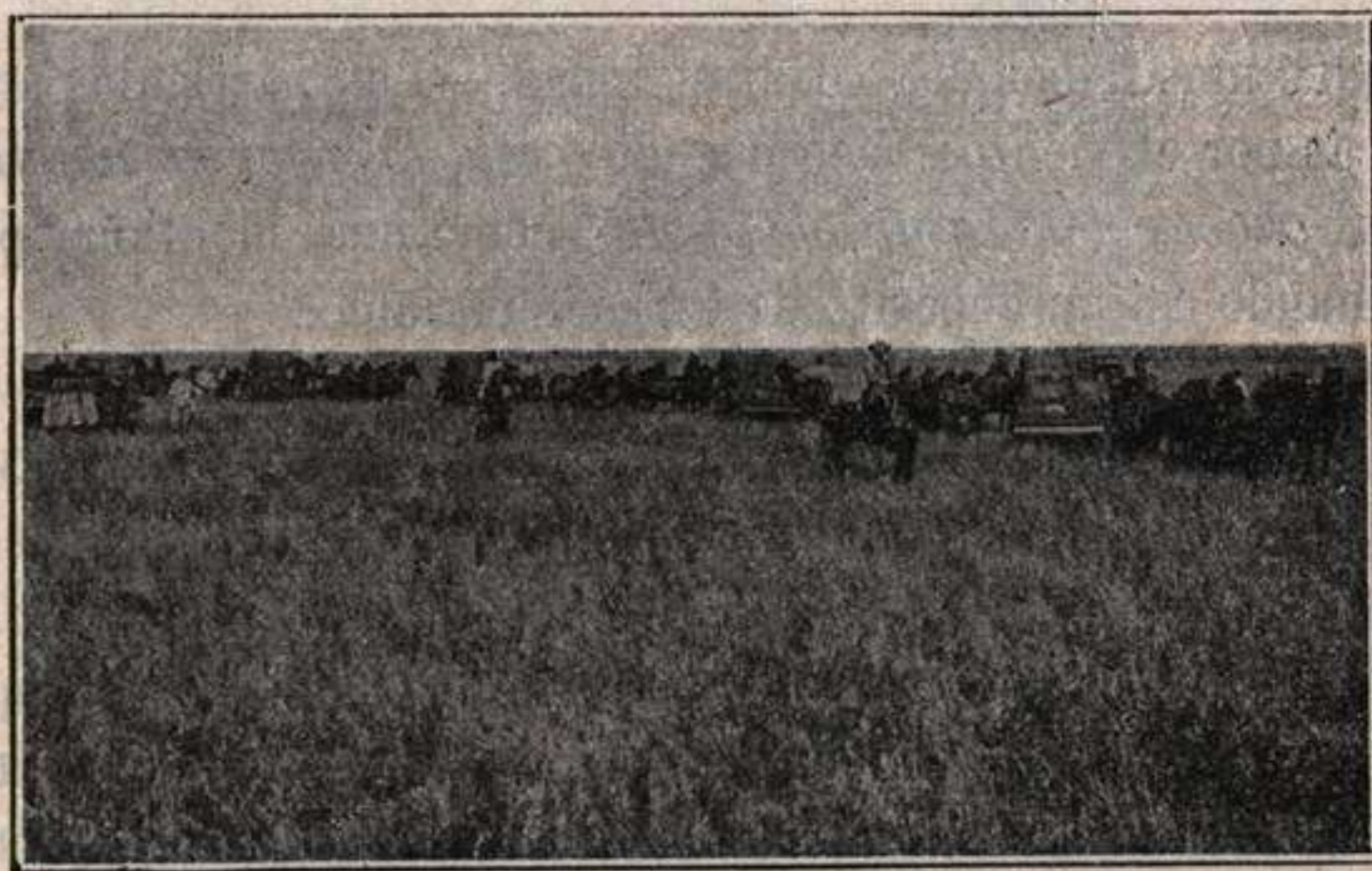
Fig. 271.—La pampa Argentina, así como otras varias pampas americanas, están formadas por loes. (Fot. com. por el prof. argentino Dr. Victor E. Miguez).
