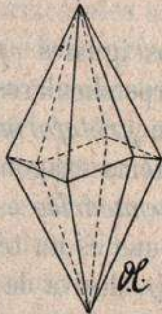
Fig. 103.—Escalenoedro.
