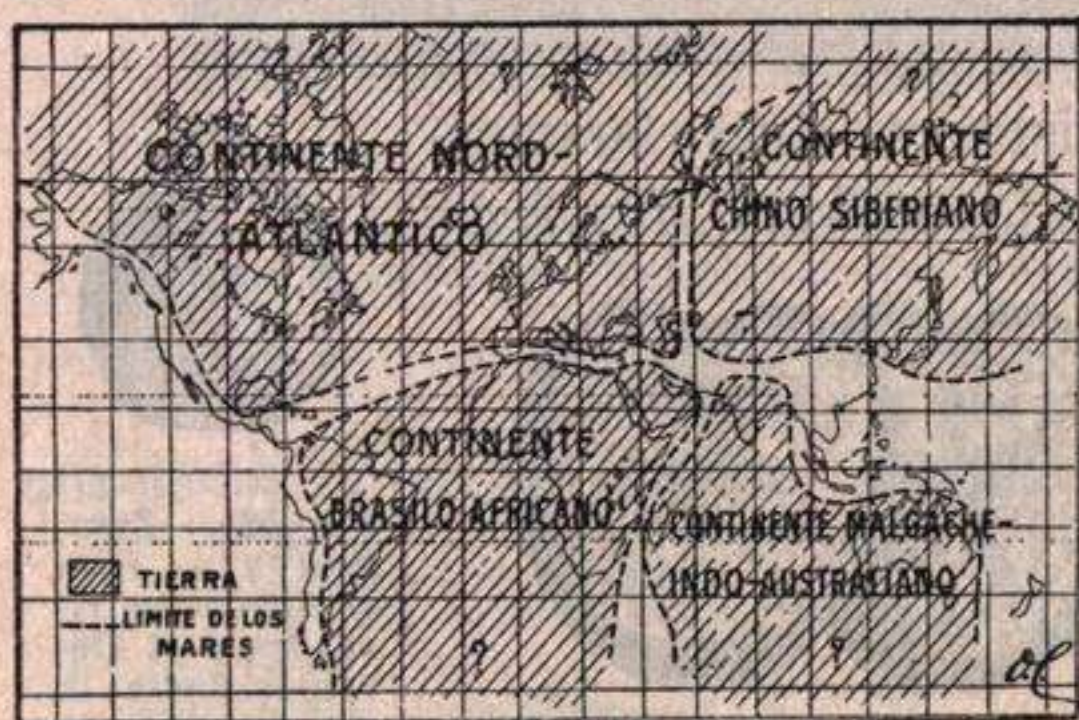
Fig. 529.—Esquema de la distribución de los continentes y de los mares al final de la Era Secundaria.
