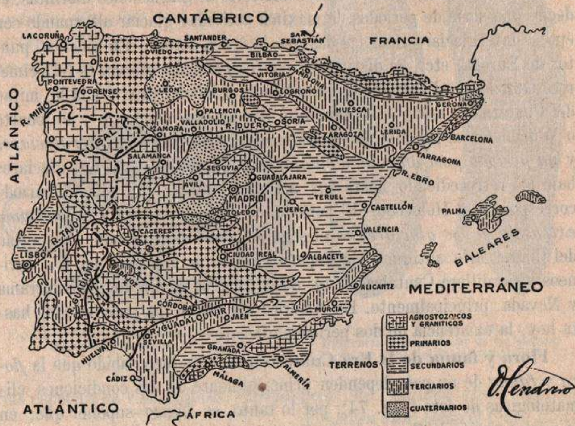
Fig. 546.—Esquema de la distribución en la Península Ibérica de los terrenos geológicos de las distintas Eras.
