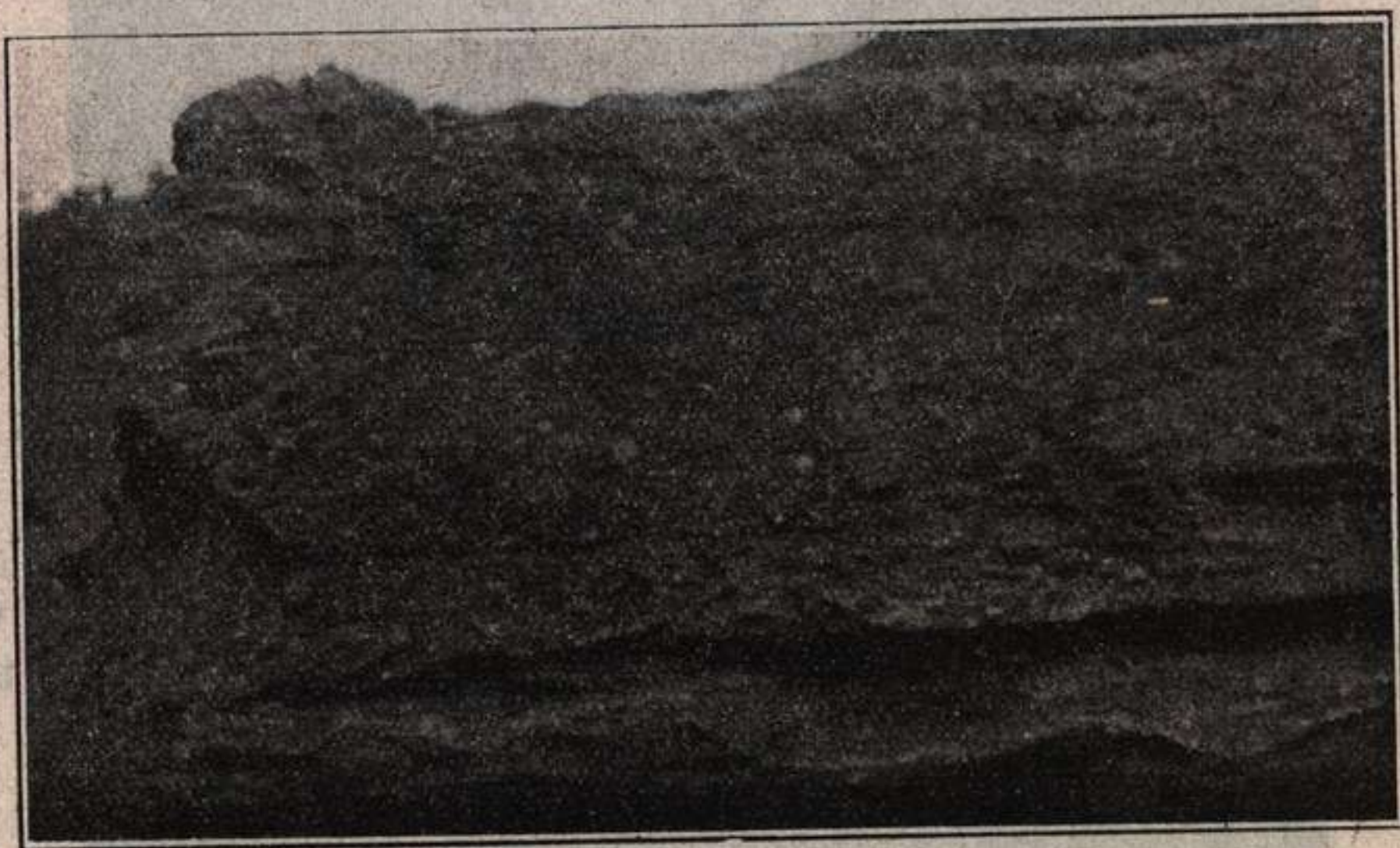
Fig. 372.—Estratificación cruzada en unos conglomerados de la provincia de Toledo. (Fotografía O. Cendrero).
