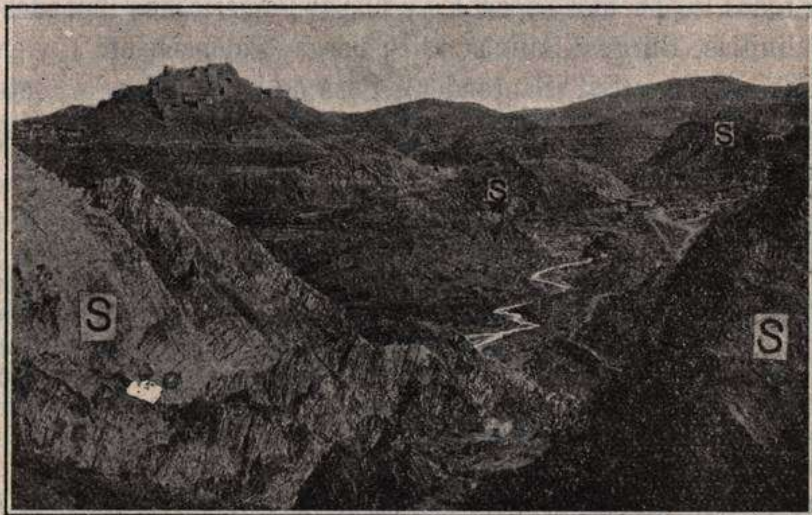
Fig. 218.—Vista general de los cerros de sal (S) de Cardona (Barcelona). En las proximidades y debajo de este yacimiento, existe otro importante de sales potásicas. (Pot. com. por el prof. Dr. M. San Miguel de la Cámara).
