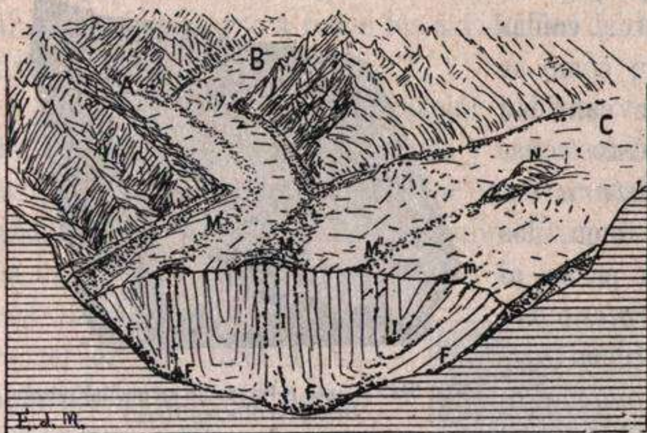
Fig. 346.—Esquema de un glaciar formado por la reunión de las lenguas de los tres glaciares A , B y C .— M , M' , morrenas superficiales centrales resultantes de la reunión de las laterales.— F , morrena profunda.— N , origen de la morrena M' . (Según E. de Martonne).
