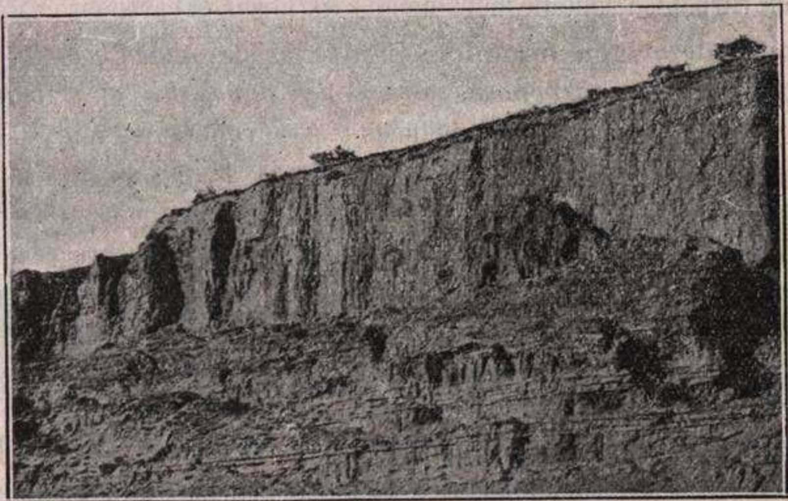
Fig. 371.—Estratos casi horizontales. (Cerro de Cantabria-Logroño). (Fot. comunicada por el ingeniero R. Sánchez Lozano).
