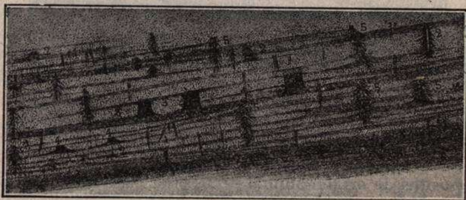
Fig. 357.—Corte de una capa de hulla (según Grand'Eury).
