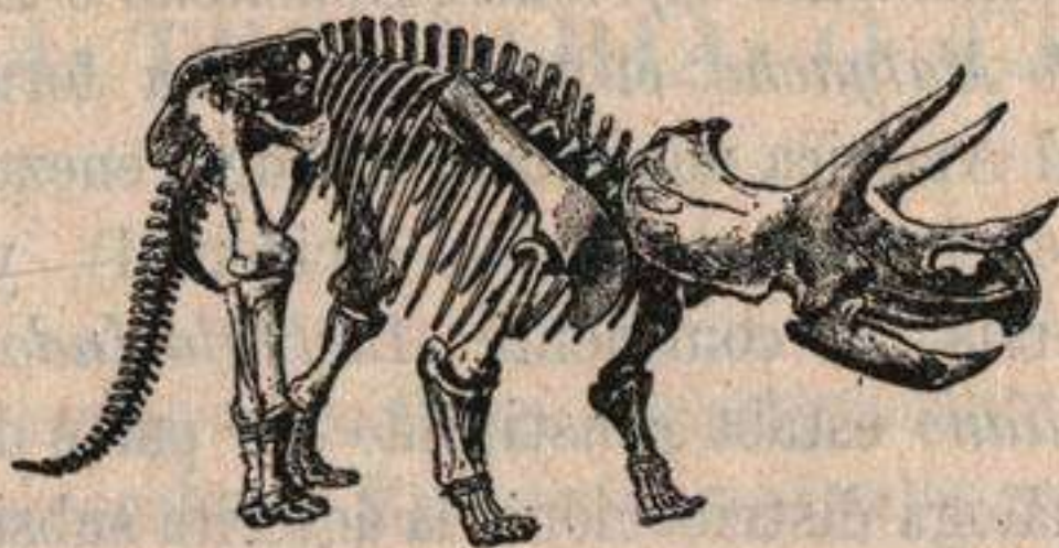
Fig. 527.— Triceratops , Reptil del Cretácico: longitud, siete metros.
