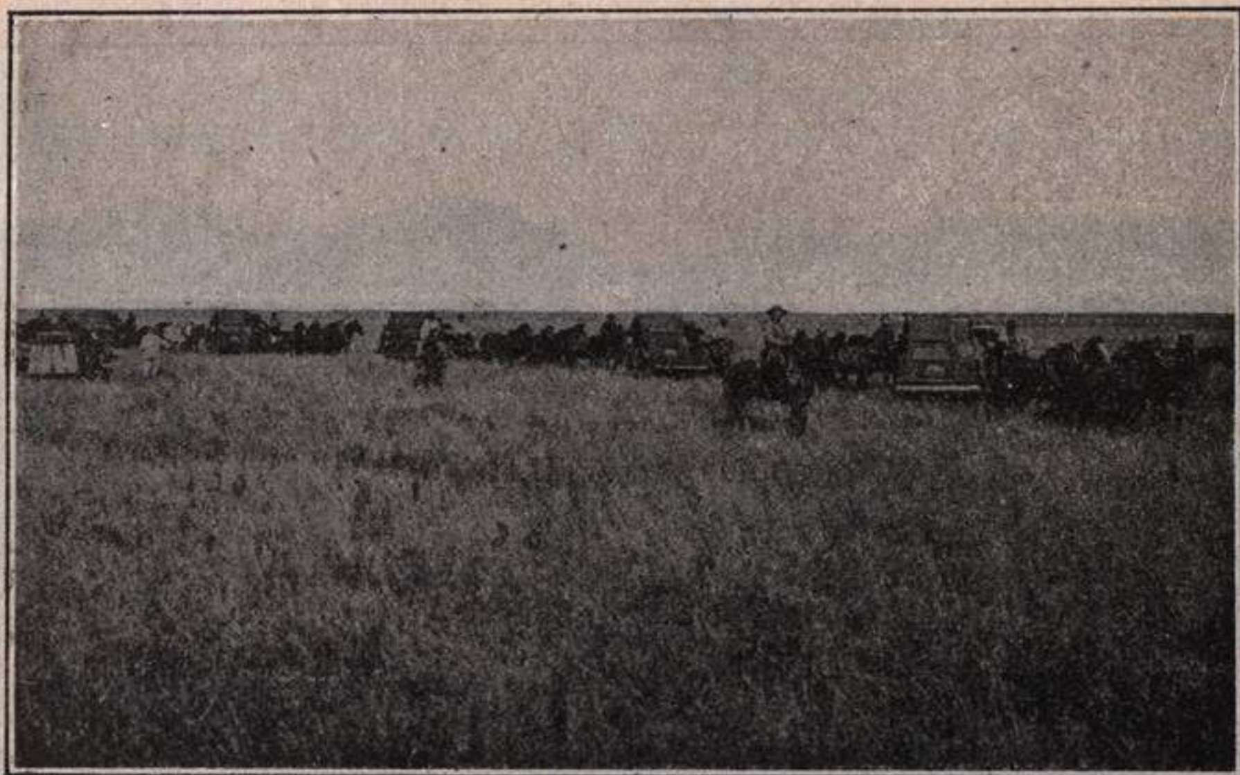
Fig. 59.—La pampa argentina como ejemplo de llanura. (Fot. comunicada por el profesor argentino Dr. Victor E. Miguez).
