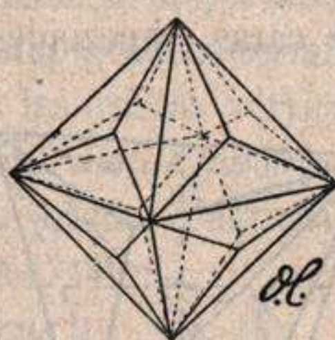
Fig. 94: Triaquisoctaedro.
