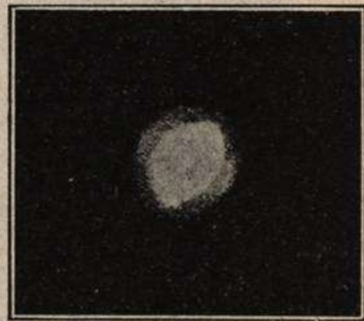
Fig. 8.—Nebulosa planetiforme de la Constelación de la Hidra. (Fot. del Observatorio de Lick).
