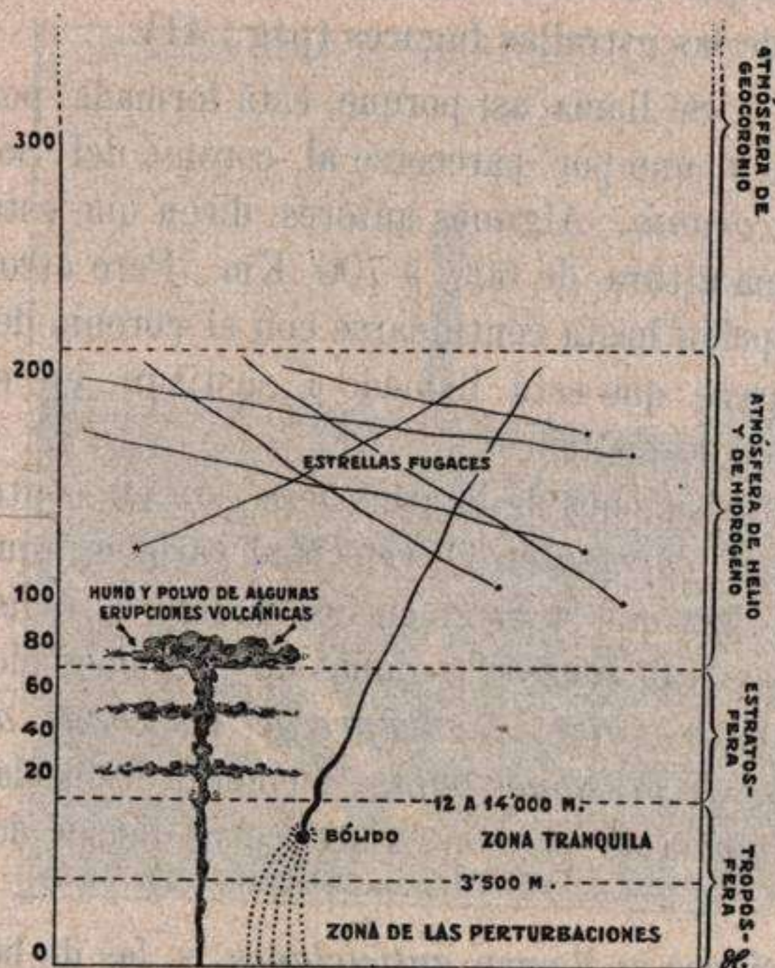
Fig. 36.—Esquema de la estructura de la atmósfera. La troposfera se representa desproporcionada con relación a las restantes partes.
