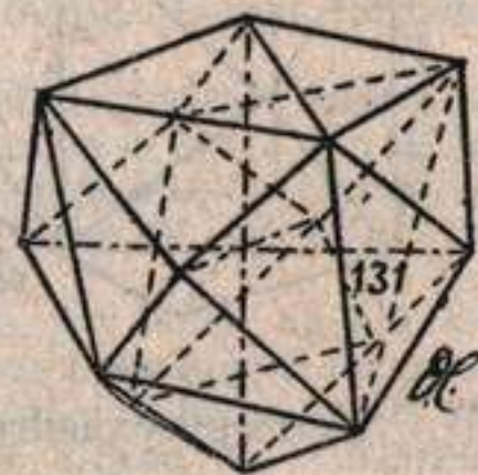
Fig. 100. Exaquistetraedro.
