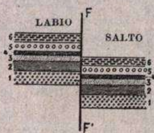
Fig. 385.—Falla vertical.
