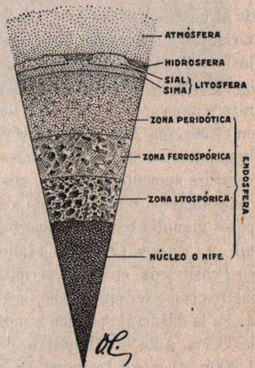
Fig. 65.--Esquema que resume las ideas actuales sobre la constitución de la Tierra en general y de la endosfera en particular. (Imit. E. Rioja).
