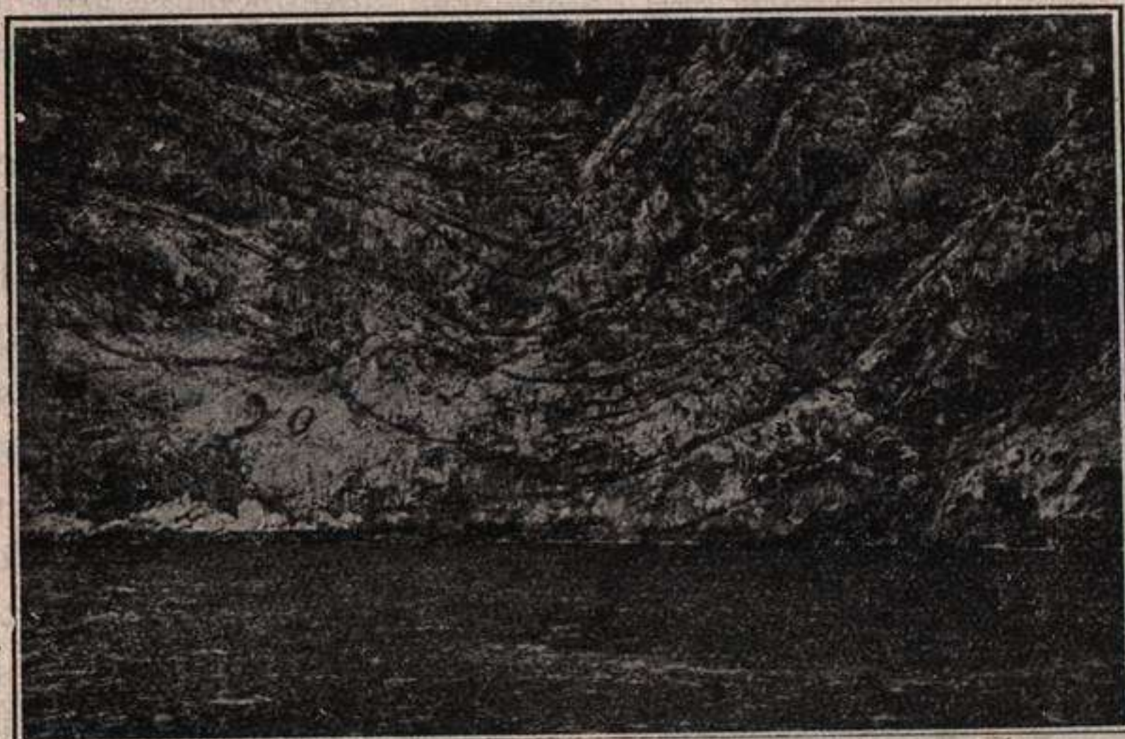
Fig. 376.—Sinclinal en la Punta del Fabioler (Andraitx-Mallorca). (Fot. por el prof. B. Darder de la col. del Museo Nacional de Ciencias Naturales com. por el prof. Dr. L. Fernández Navarro).
