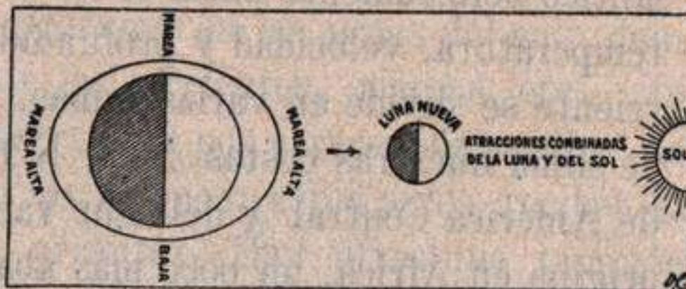
Fig. 44.—Explicación de las mareas: marea viva.
