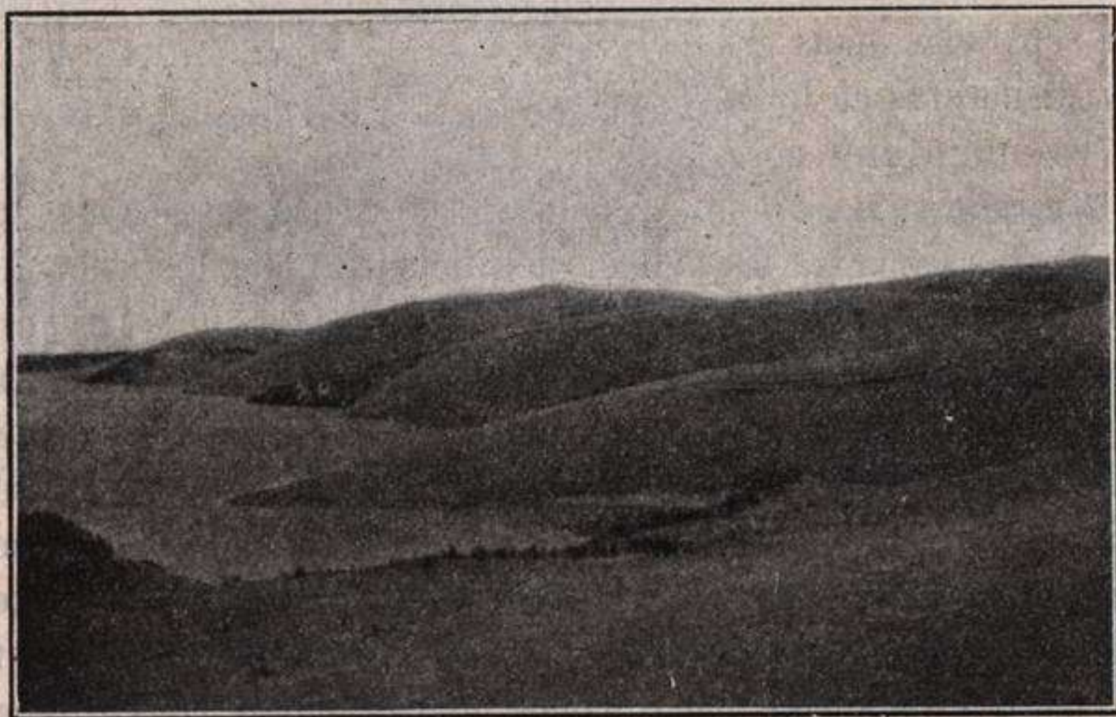
Fig. 274.—Cadena de dunas de Liencres, mal llamadas de Mogro (Santander). (Fotografía O. Cendrero).
