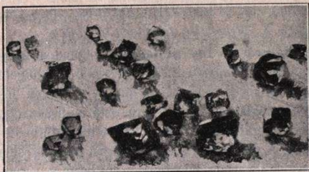
Fig. 186.—Diamantes cristalizados en octaedros, etc., tal como se sacan de la mina, que era la forma en que se usaron hasta el siglo xv. (Fot. comunicada por el Dr. Heismaus, de Transvaal).
