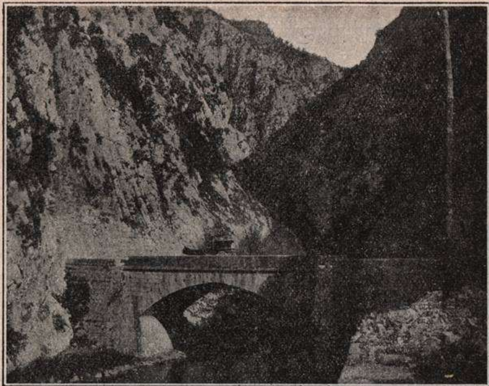
Fig. 302.—Una hoz del Río Deva (Santander-Asturias). Las rocas claras, son las de la orilla derecha del río, y las oscuras, las de la izquierda. (Fotografía comunicada por el profesor Dr. J. Rioja).
