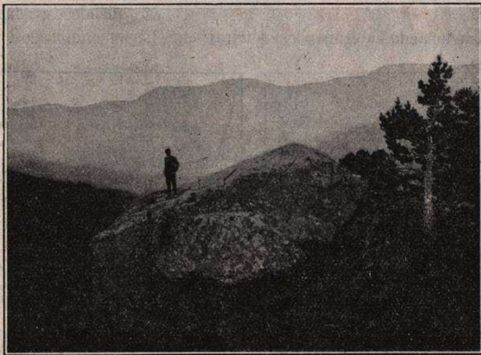
Fig. 345.—Bloque errático en la Sierra de Guadarrama. (Del trabajo Los glaciares cuaternarios de la Sierra de Guadarrama , por los profs. Dr. H. Obermaier y Dr. J. Carandell).
