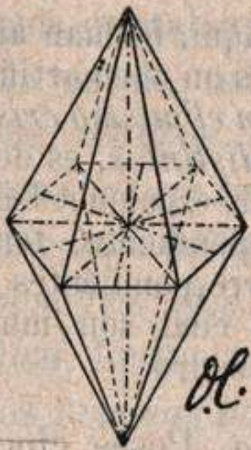
Fig. 101.—Pirámide exagonal.
