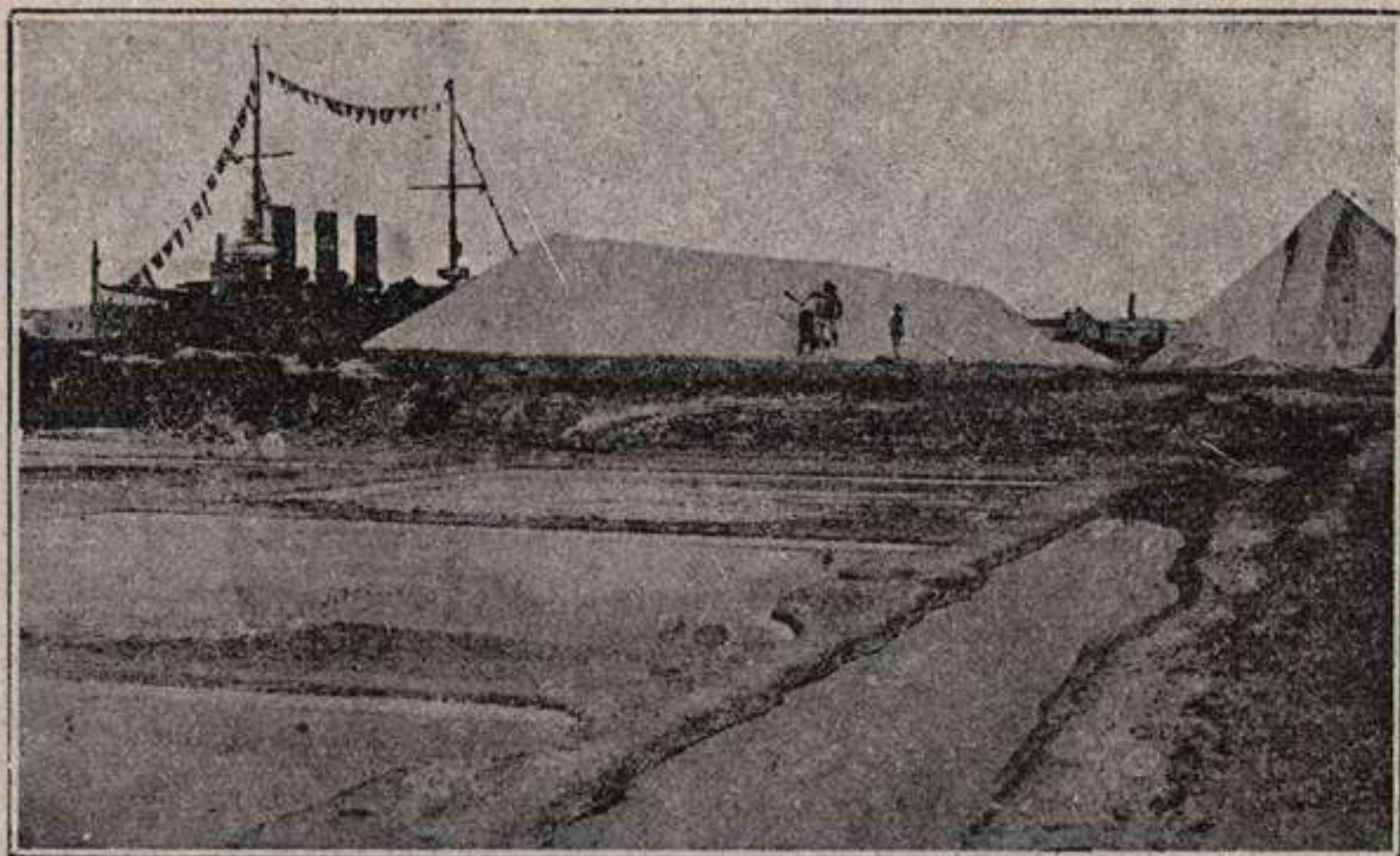
Fig. 217.—Vista parcial de las salinas de San Fernando (Cádiz); en segundo término, los montones o parvas de sal. (Fotografía comunicada por el profesor doctor V. Martínez Gámez).
