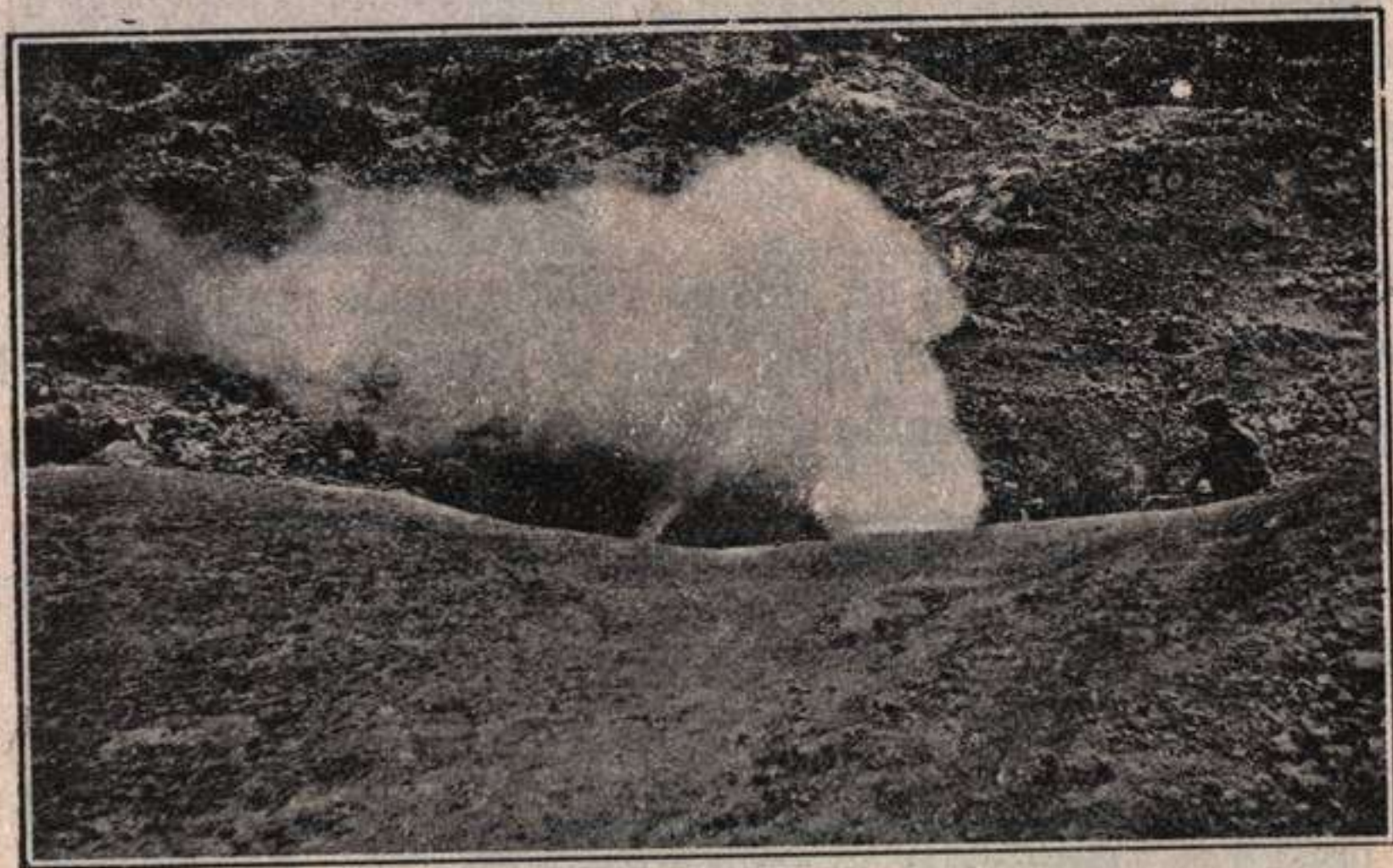
Fig. 413.—Solfataras de Puzzuoli, cerca del Vesubio; es una de las mejor estudiadas. (Fotografía Perret).
