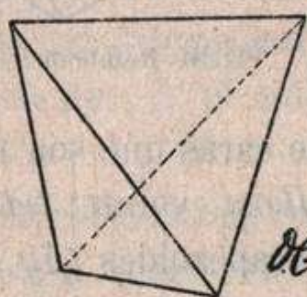
Fig. 96. Tetraedro.
