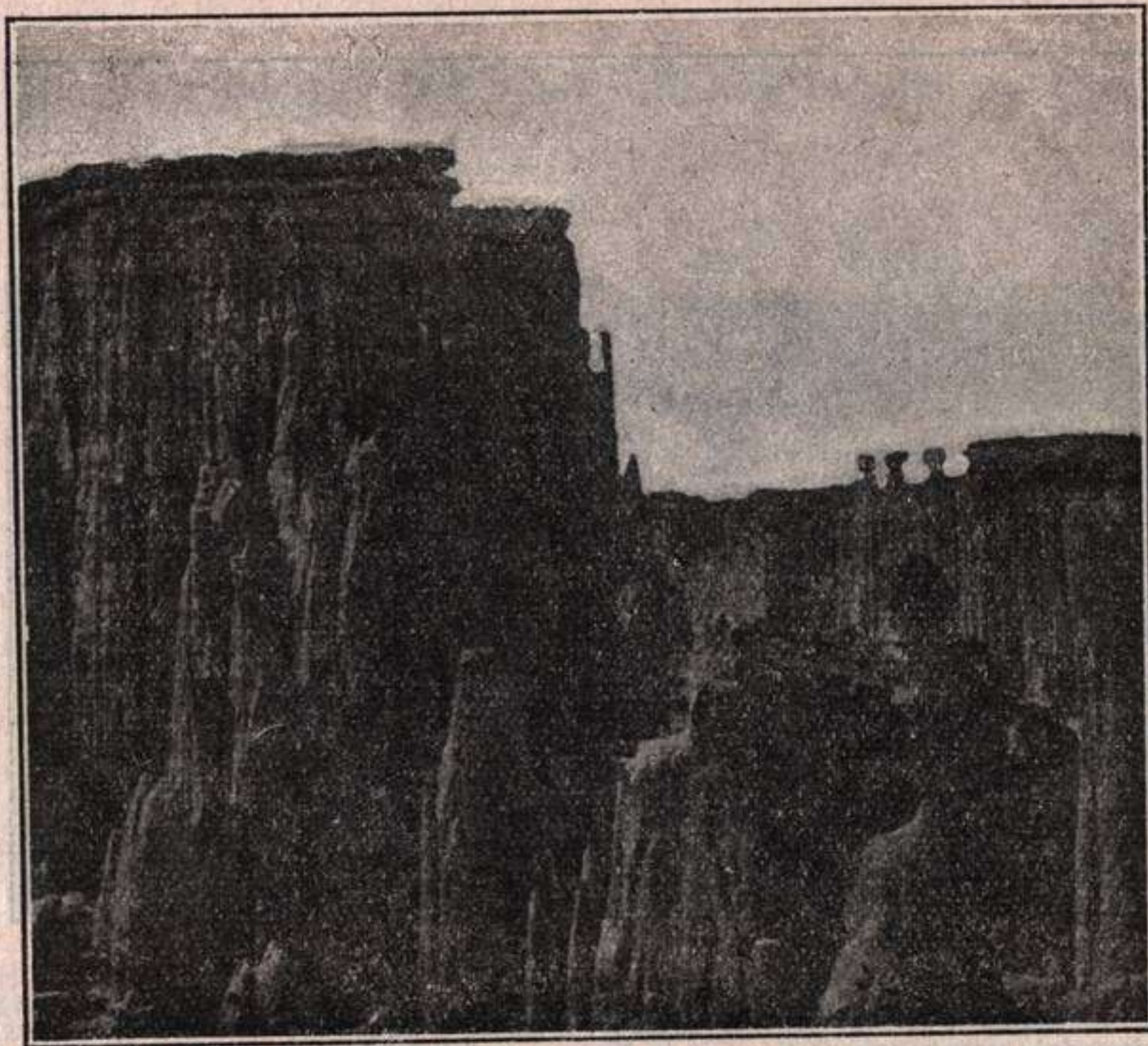
Fig. 288.—En cambio, si la roca es blanda, como la que representa la figura, que está formada por una arenisca (o arenas cementadas) poco coherente, el agua de lluvia, en lugar de separar bloques, arrastra la arena y origina esta topografía característica. (Fot. de Bogotá (Colombia) comunicada por la profesora colombiana Ana Torres Plata).
