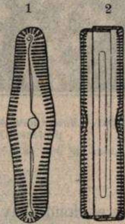
Fig. 360.—Diatomea vista de frente, 1, y de perfil, 2.
