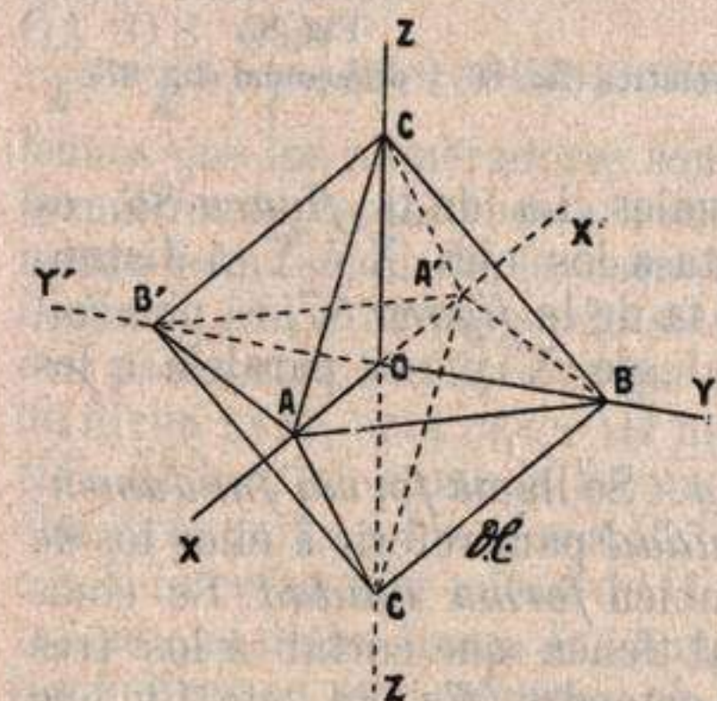
Fig. 84.—Ejes cristalográficos.
