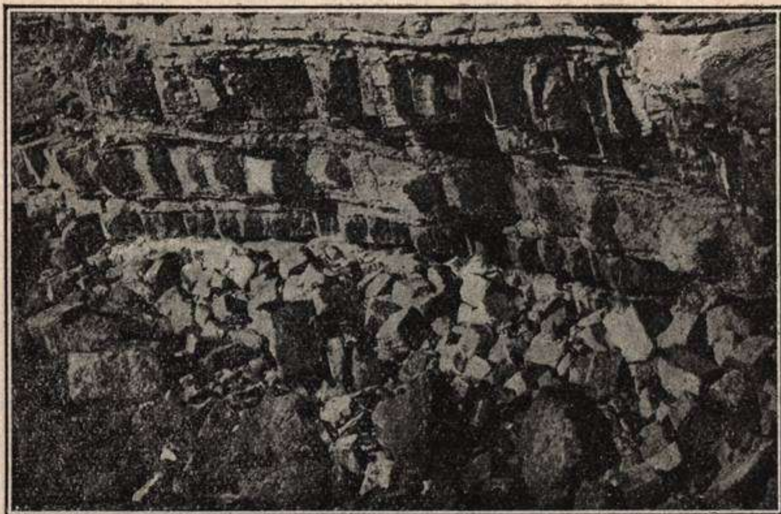
Fig. 287.—El agua de lluvia que penetra por las fisuras de los estratos o capas de la roca dura de la parte superior, unida a la acción mecánica y química de la atmósfera, ha determinado su rotura en los bloques paralelepípedicos de la parte inferior de la figura. Y éstos, a su vez, pasan a cantos rodados al continuar la acción de los agentes citados. (Fotografía O. Cendrero).
