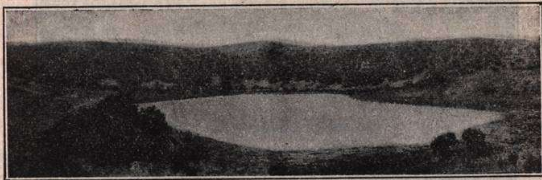
Fig. 398.—La Laguna de la Posadilla (Valverde de Calatrava-Ciudad Real), como ejemplo de cráter de volcán apagado, actualmente lleno de agua. (Fot. com. por el Pbro. J. M. a de la Fuente).
