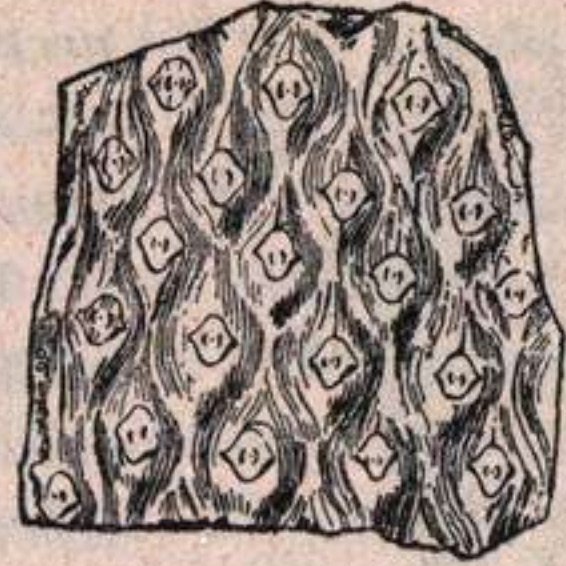
Fig. 495.—Trozo de corteza de Sigillaria , Licopodinea del Devónico y Carbonífero
