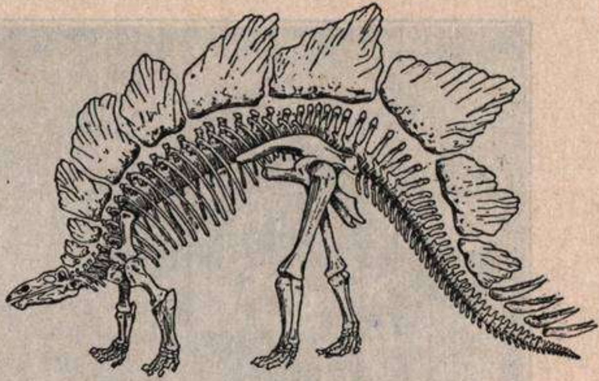
Fig. 518.—Esqueleto de Stegosaurus , Reptil andador del Jurásico: longitud, 10 metros.
