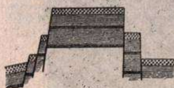
Fig. 391.—Horst.
