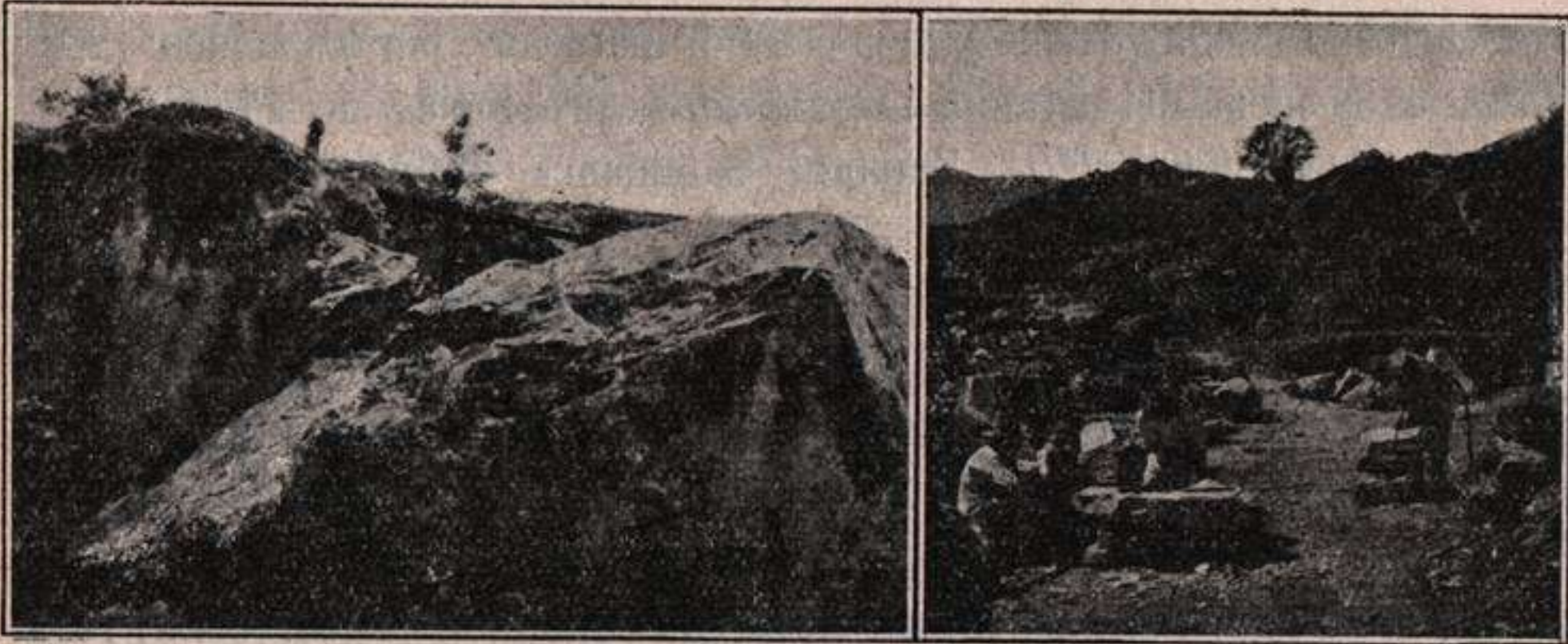
Fig. 208.—Cantera de Ónice «La Peña» en Etna (Oaxaca-Méjico).
