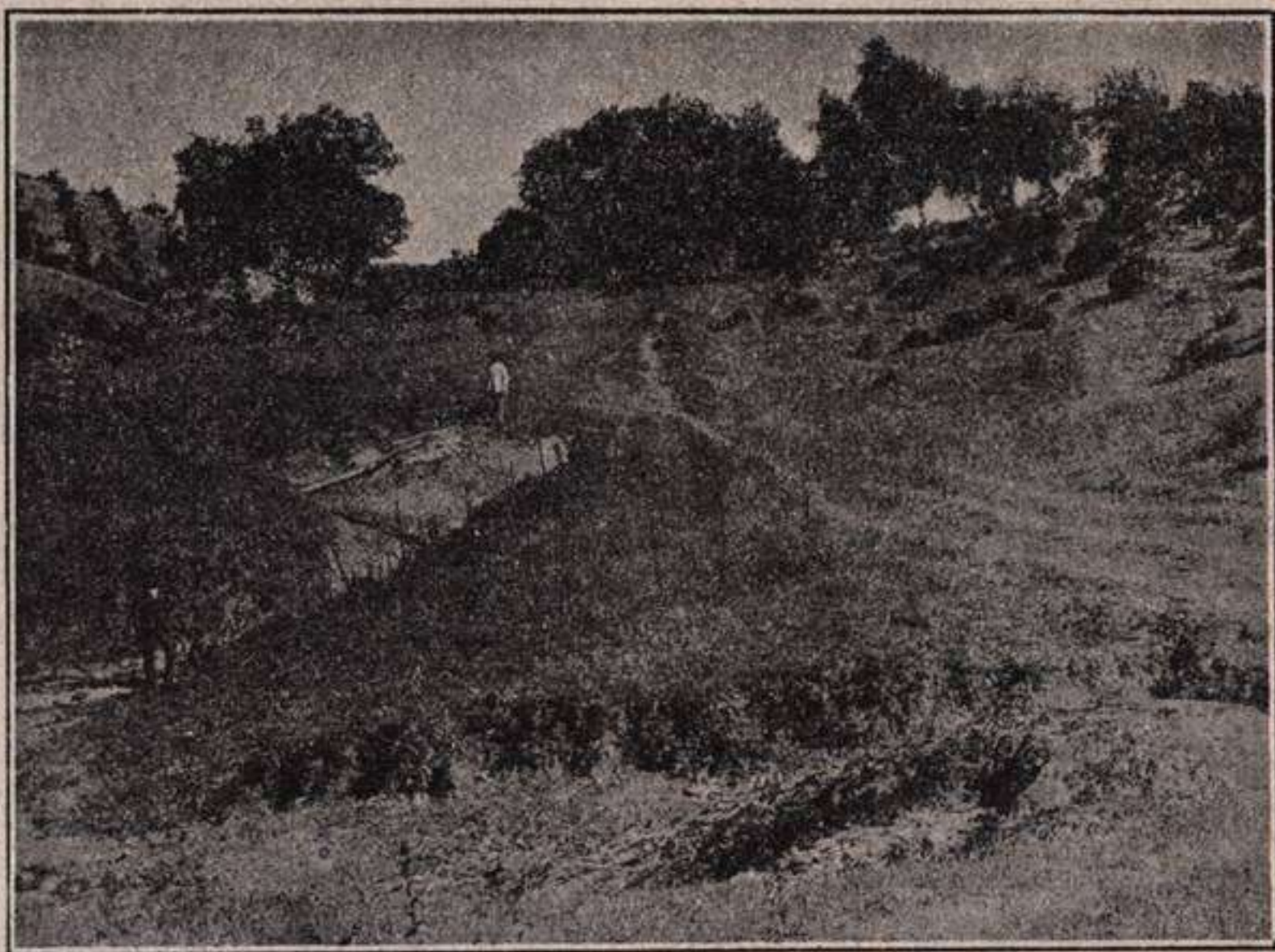
Fig. 416.—Una macaluba de Morón (Sevilla). (Fot. J. Plata Nieto, com. por el prof. E. Albórs).
