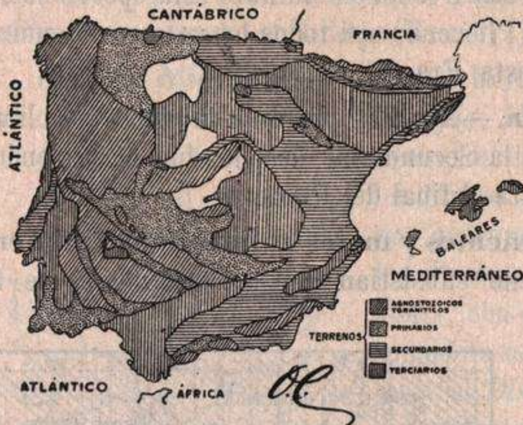
Fig. 545.—Esquema de la distribución en la Península Ibérica de los Terrenos Primarios, Secundarios y Terciarios.
