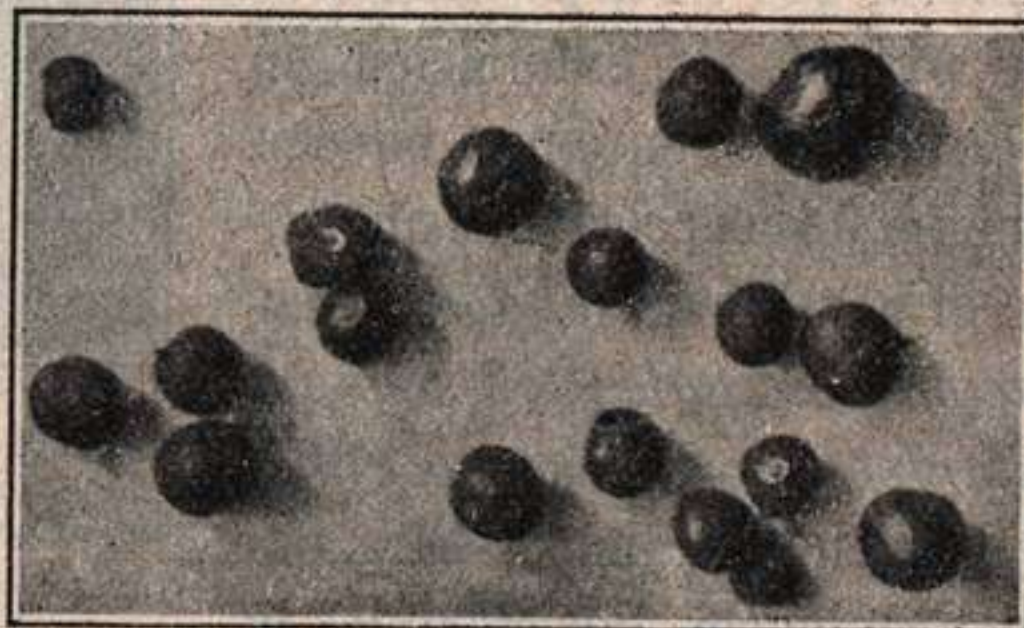
Fig. 146.—Pisolitas aisladas. (Fot. O. Cendrero).
