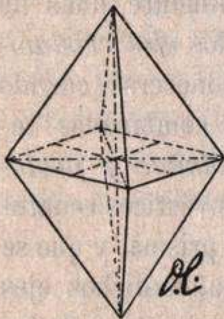
Fig. 105. — Pirámide tetragonal.
