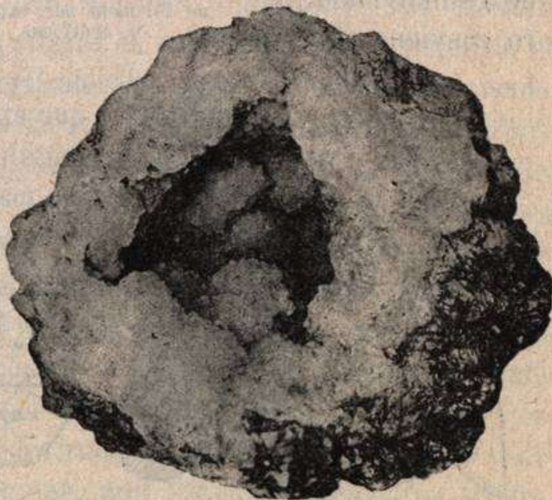
Fig. 119.—Geoda de cuarzo. (Fot. O. Cendrero).
