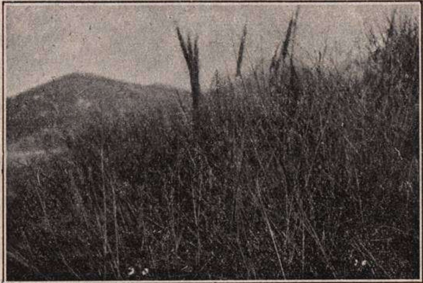
Fig. 282.—Gramináceas (principalmente Psamma arenaria ) que fijan espontáneamente las dunas vivas. (Fot. O. Cendrero).
