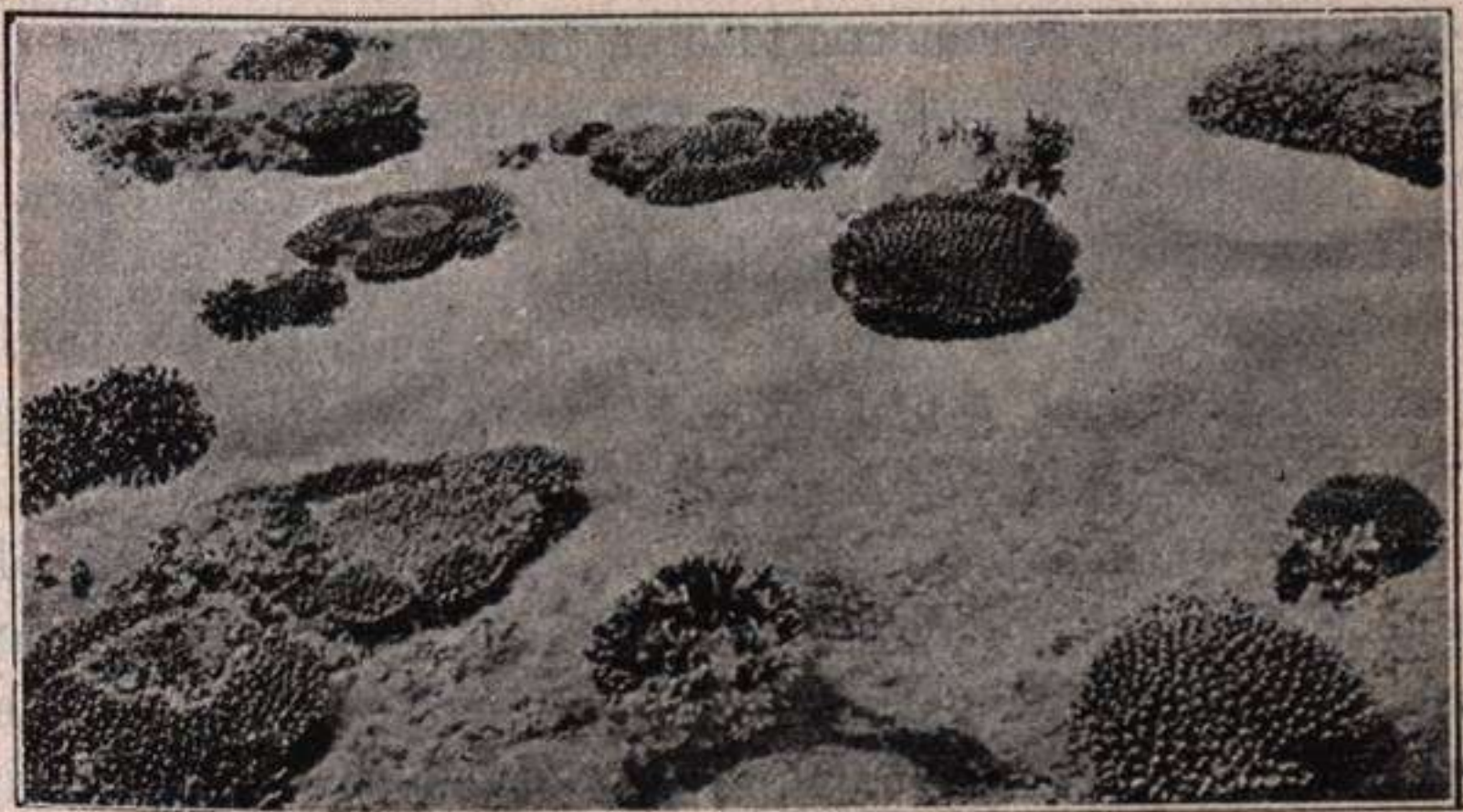
Fig. 363.—Vista parcial de un arrecife de coral en la marea baja.
