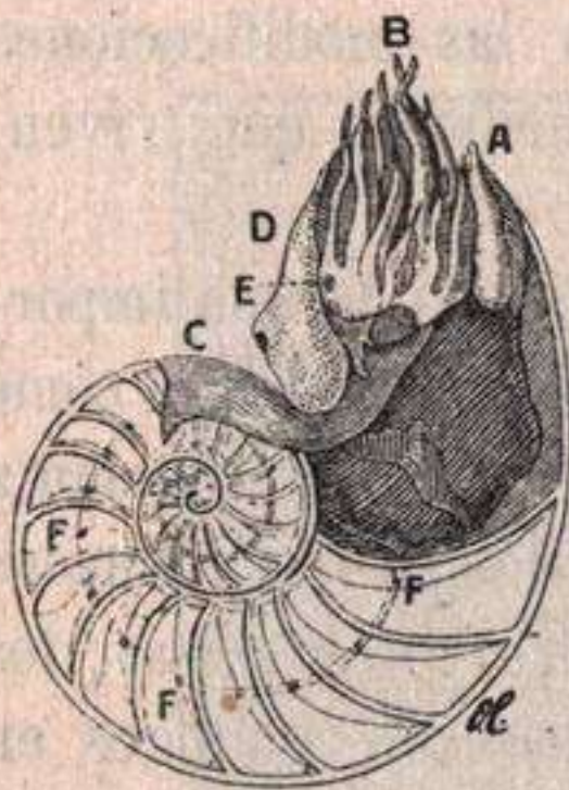
Fig. 481.— Nautilus .—A, B, C, D, E, animal contenido en la última cámara de la concha; F, sifón que pone en comunicación las diversas cámaras de ésta.
