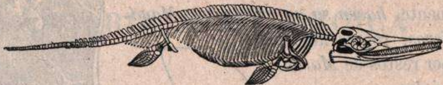
Fig. 514.—Esqueleto de Ichtyosáurnus , Reptil nadador del Jurásico: longitud: 10 metros
