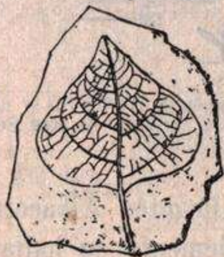
Fig. 531.—Impresión de una hoja de chopo ( Populus modesta ) del Eoceno: longitud, nueve centímetros.
