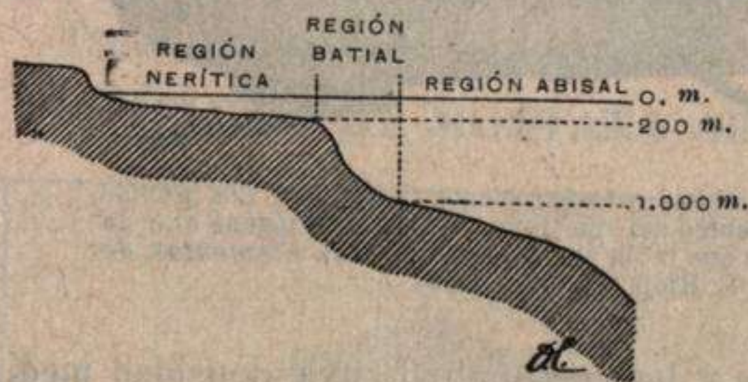
Fig. 48.—Esquema de las regiones marinas. (Imit. Haug).
