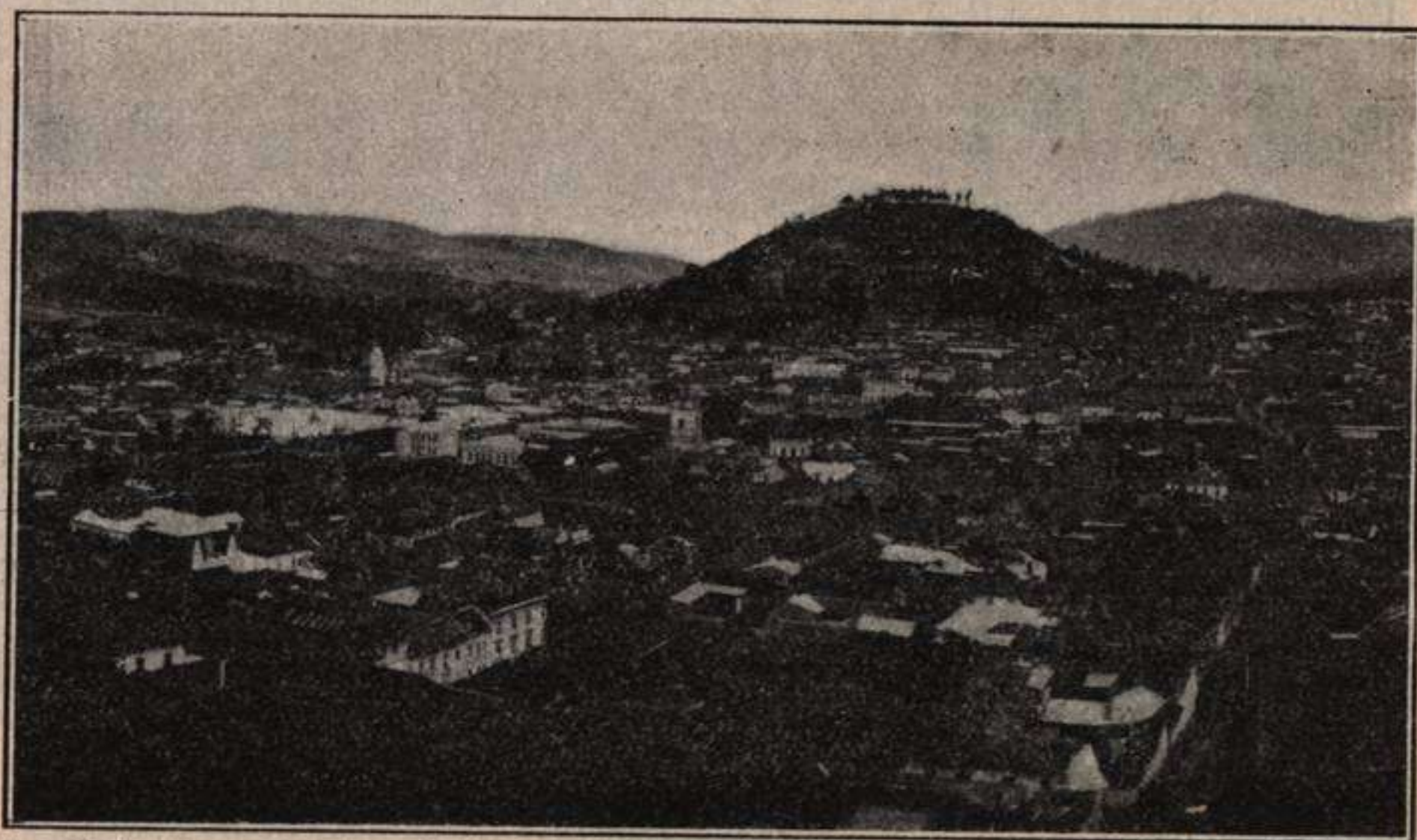
Fig. 57.—Vista parcial de la ciudad de Quito (Ecuador), que está edificada en la altiplanicie de su nombre, a los 2.850 m. de altura. (Fot. I. Pazmiño, comunicada por la profesora ecuatoriana Bl. Andrade).
