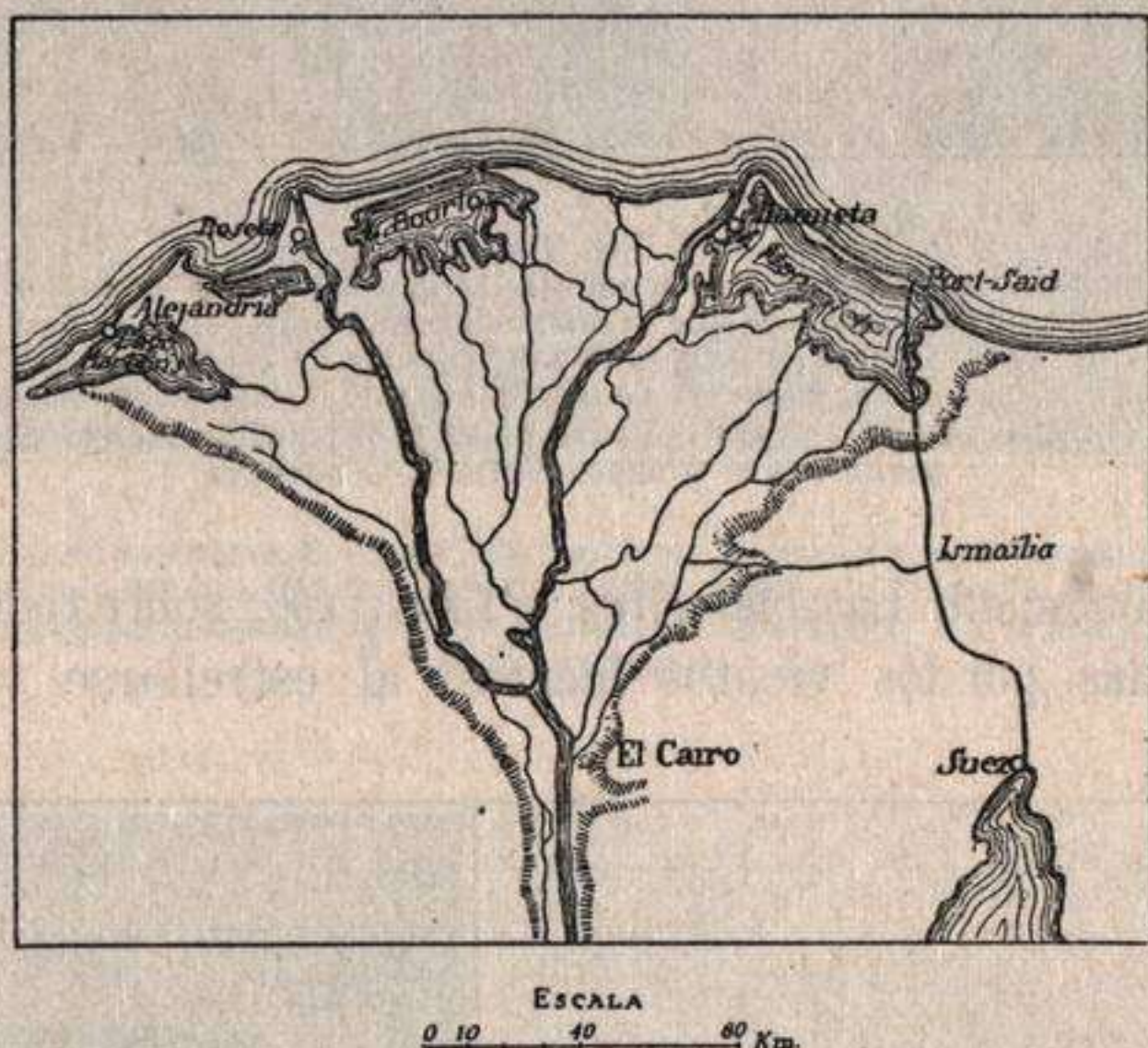
Fig. 313.—Delta del Nilo (según Petermann). (De la obra Elementos de Geología , por L. F. Navarro y O. Cendrero).
