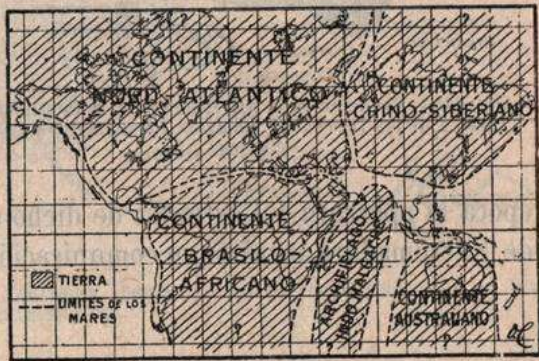
Fig. 543.—Esquema de la distribución de los continentes y de los mares al final del Paleógeno.
