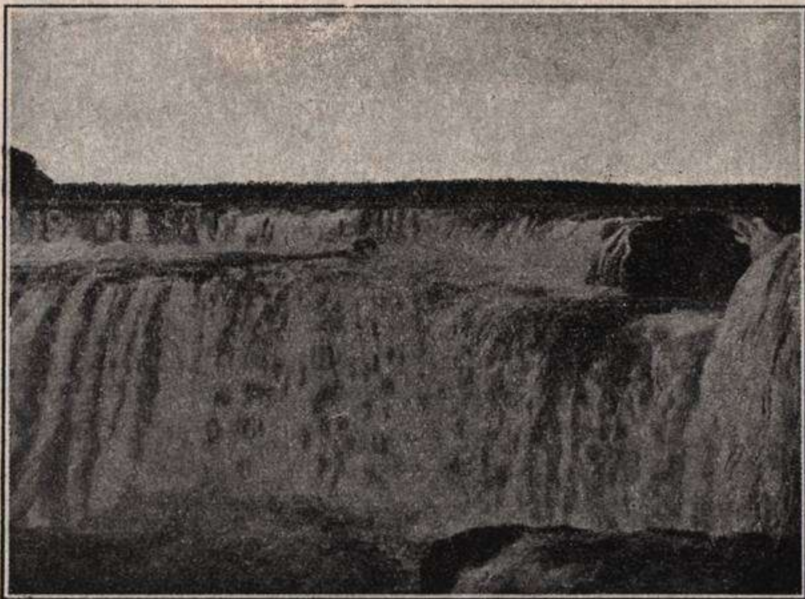
Fig. 304.—Generalmente son poco conocidas las grandiosas cataratas del río Iguazu (Brasil-Argentina), cuya magnificencia iguala, si no excede, a la de otras más renombradas. La de la fotografía representa una de las dos consecutivas que presenta el río, cada una de las cuales tiene 32 metros de altura. (Fot. com. por el prof. argentino Dr. César Acardi).
