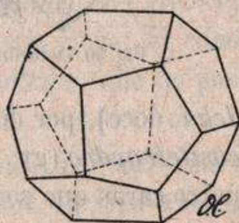
Fig. 97. Pentadodecaedro.
