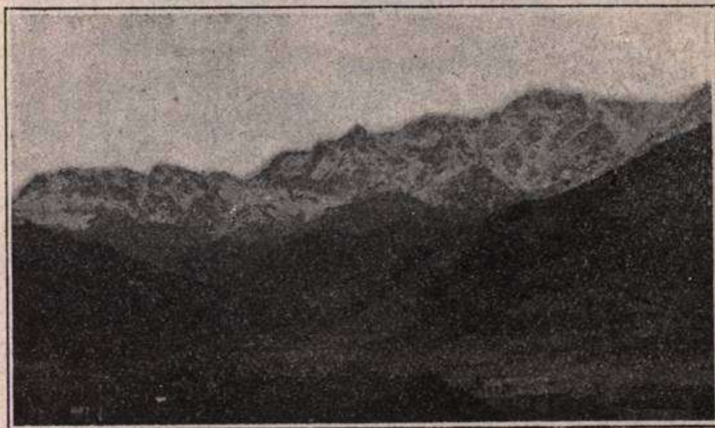
Fig. 56.—La cordillera cantábrica (en la región llamada Peñas o Picos de Europa), vista desde Potes (Santander). (Fot. O. Cendrero).
