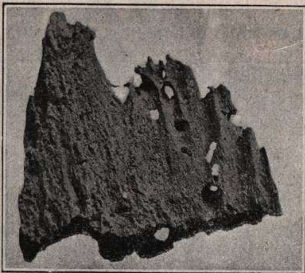
Fig. 258.—Canto calizo estriado por corrosión. (De Elementos de Geología , por L. Fernández Navarro y O. Cendrero).
