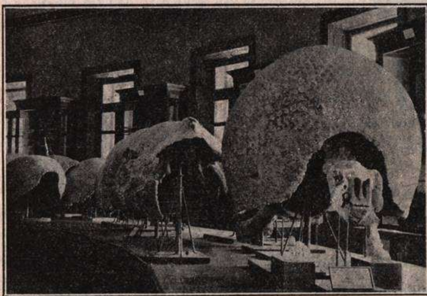
Fig. 554.—Grupo de corazas de Glyptodon , del Museo de Historia Natural de la Plata (Argentina). (Fot. com. por el prof. Doctor A. Bosca).
