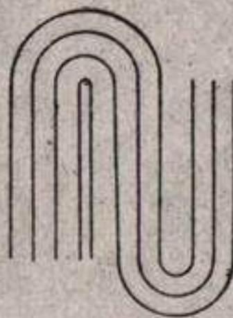
Fig. 379.—Pliegues isoclinales.
