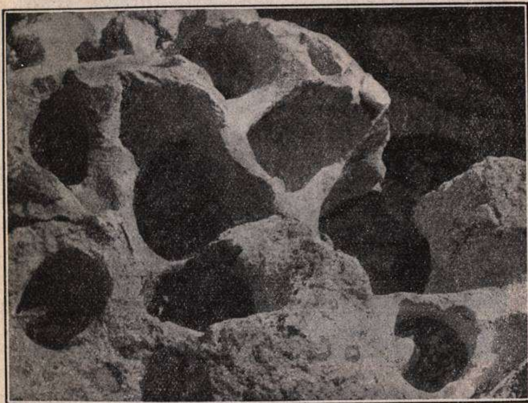
Fig. 309.—Pilas u ollas en el río Torio (Hoces de Vegacervera-León). (Fot. com. por el profesor Dr. J. Gómez de Llarena).
