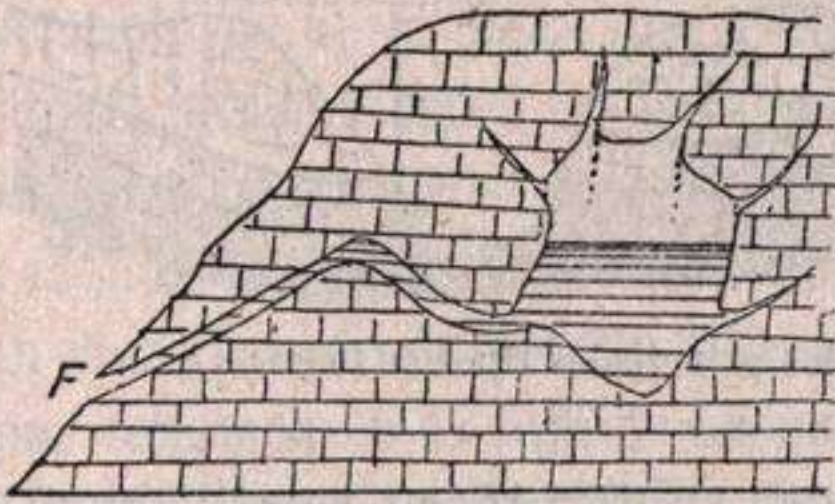
Fig. 330.—Teoría de la fuente intermitente sencilla, F .
