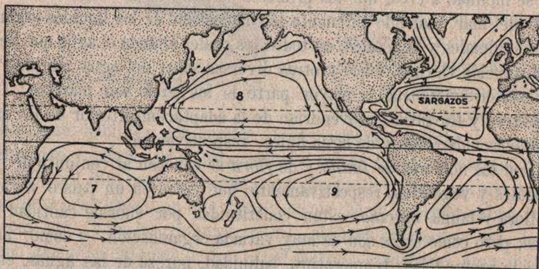
Fig. 46.—Mapa esquematizado de las corrientes oceánicas: la tierra firme se representa punteada. (De la obra Elementos de Geología , por L. Fernández Navarro y O. Cendrero).
