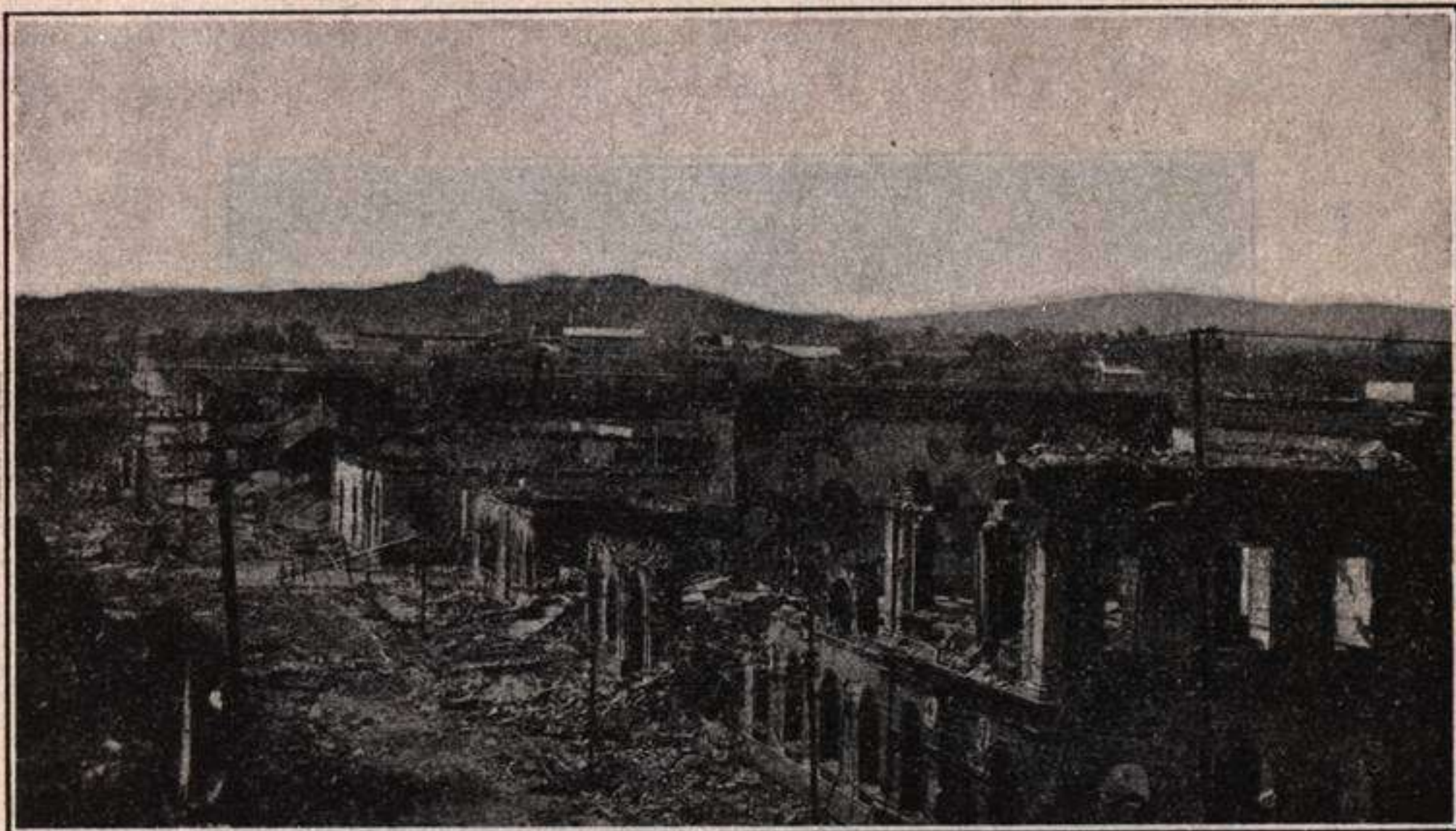
Fig. 452 bis.—Vista parcial de la ciudad de Managua (Nicaragua), (más de 60.000 habitantes), totalmente destruida por el terremoto de 31 de marzo de 1931. (Fot. com. por el prof. nicaragüense Alejandro Marengo h.)
