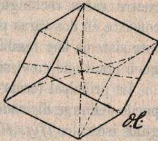
Fig. 104.—Romboedro.
