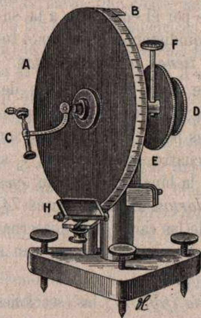
Fig. 73.—Goniómetro de reflexión de Wollaston y esquema explicativo. (De la obra Prácticas de Mineralogía y Geología , por J. Royo y O. Cendrero).
