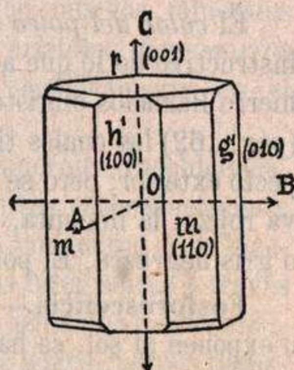
Fig. 168.—Cristal de Cordierita, como ejemplo de mineral con policroísmo.
