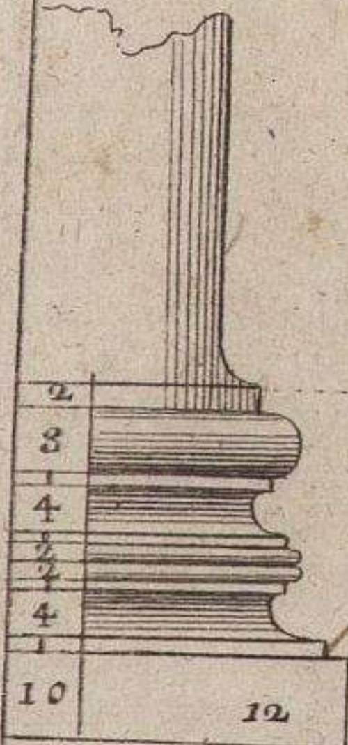
Capitello, e Base Ionica
