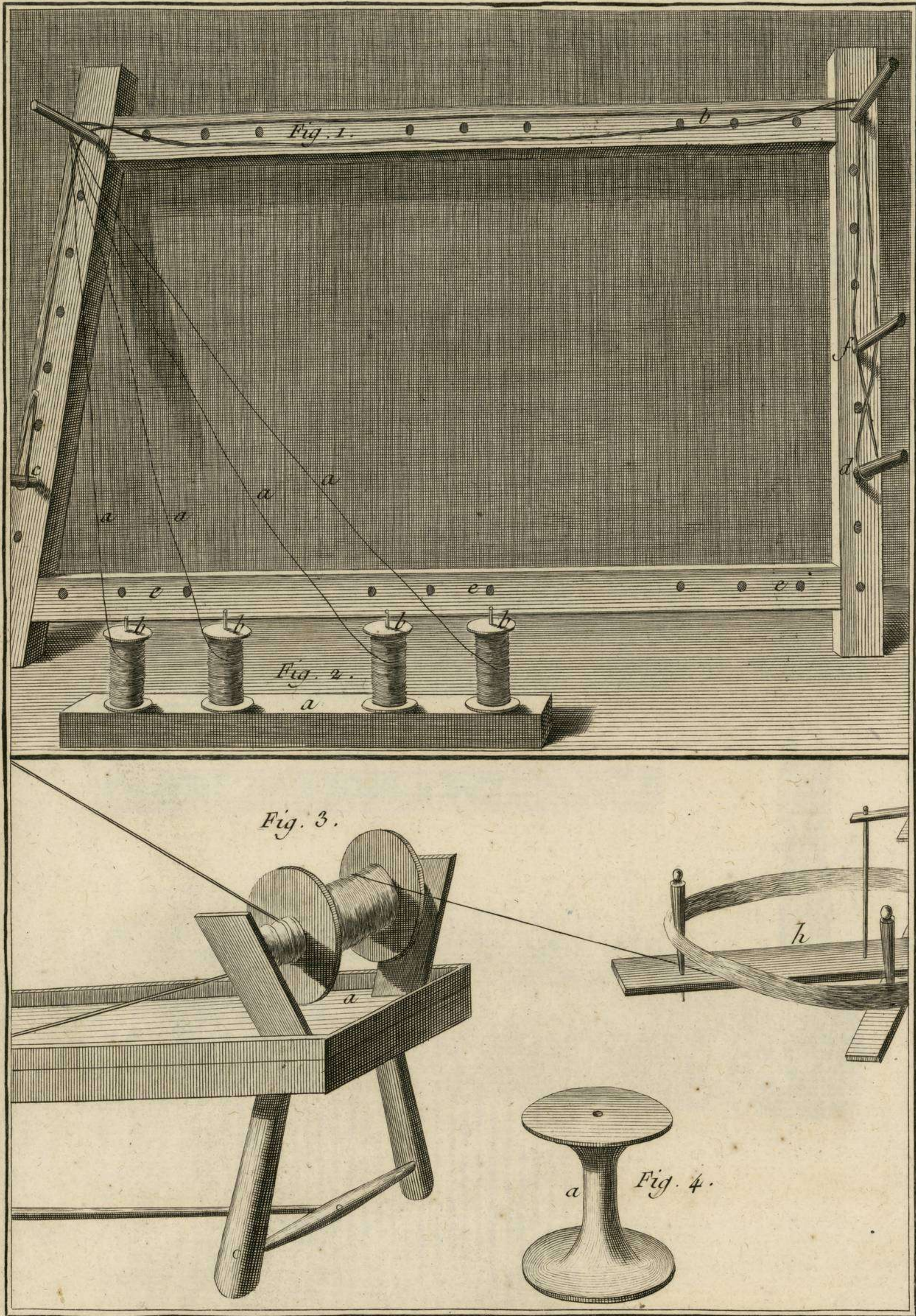
Benard direxit Tapisserie de Haute Lisse des Gobelins, Service de l'Ourdissoir.
