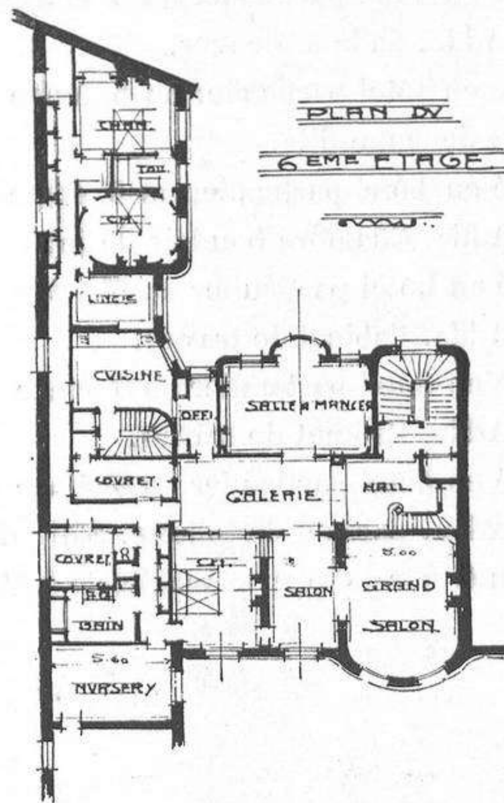
Plan de l'appartement disposé en hôtel particulier, rue Ampère, à Paris. — Architecte : M. ADDA.
