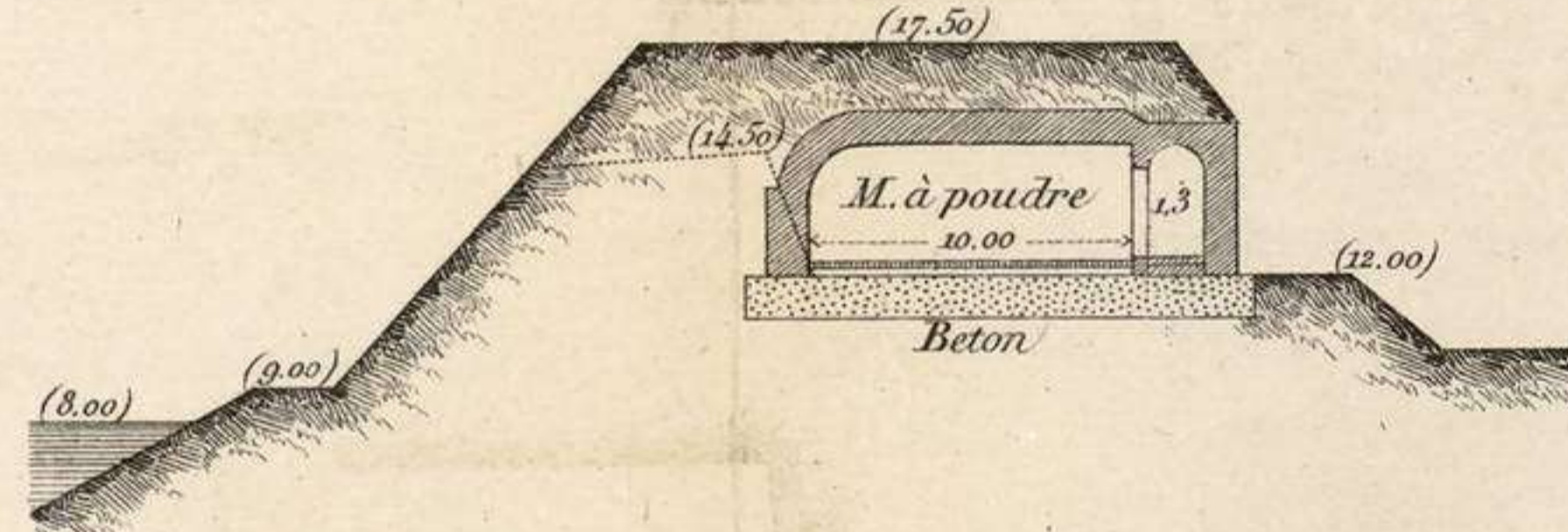
Coupe sur EF.
