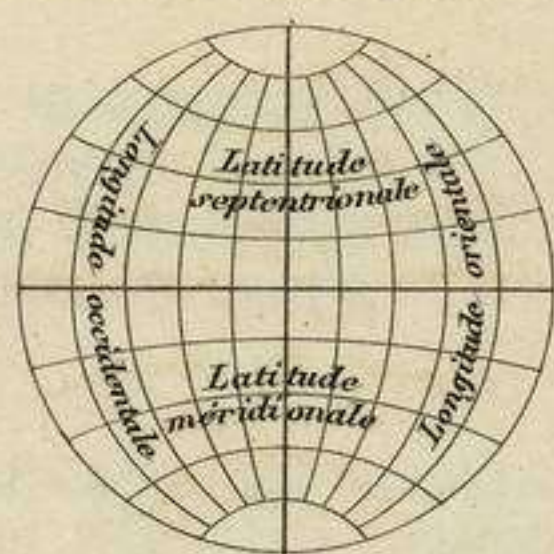
LATITUDE, LONGITUDE.
