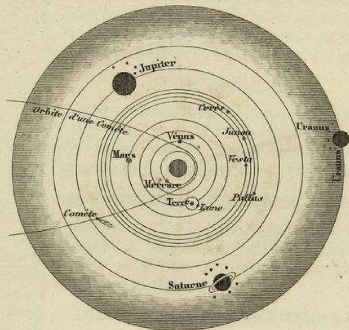
SYSTÈME PLANÉTAIRE.
