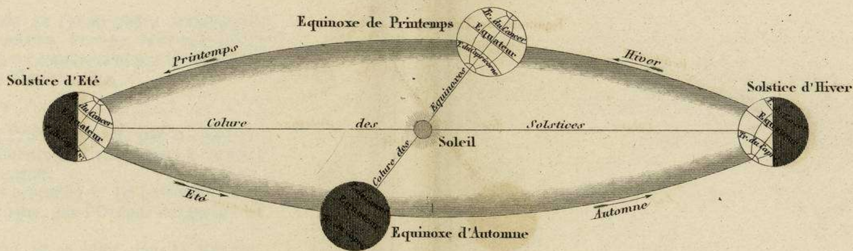
RÉVOLUTION ANNUELLE DE LA TERRE AUTOUR DU SOLEIL.
