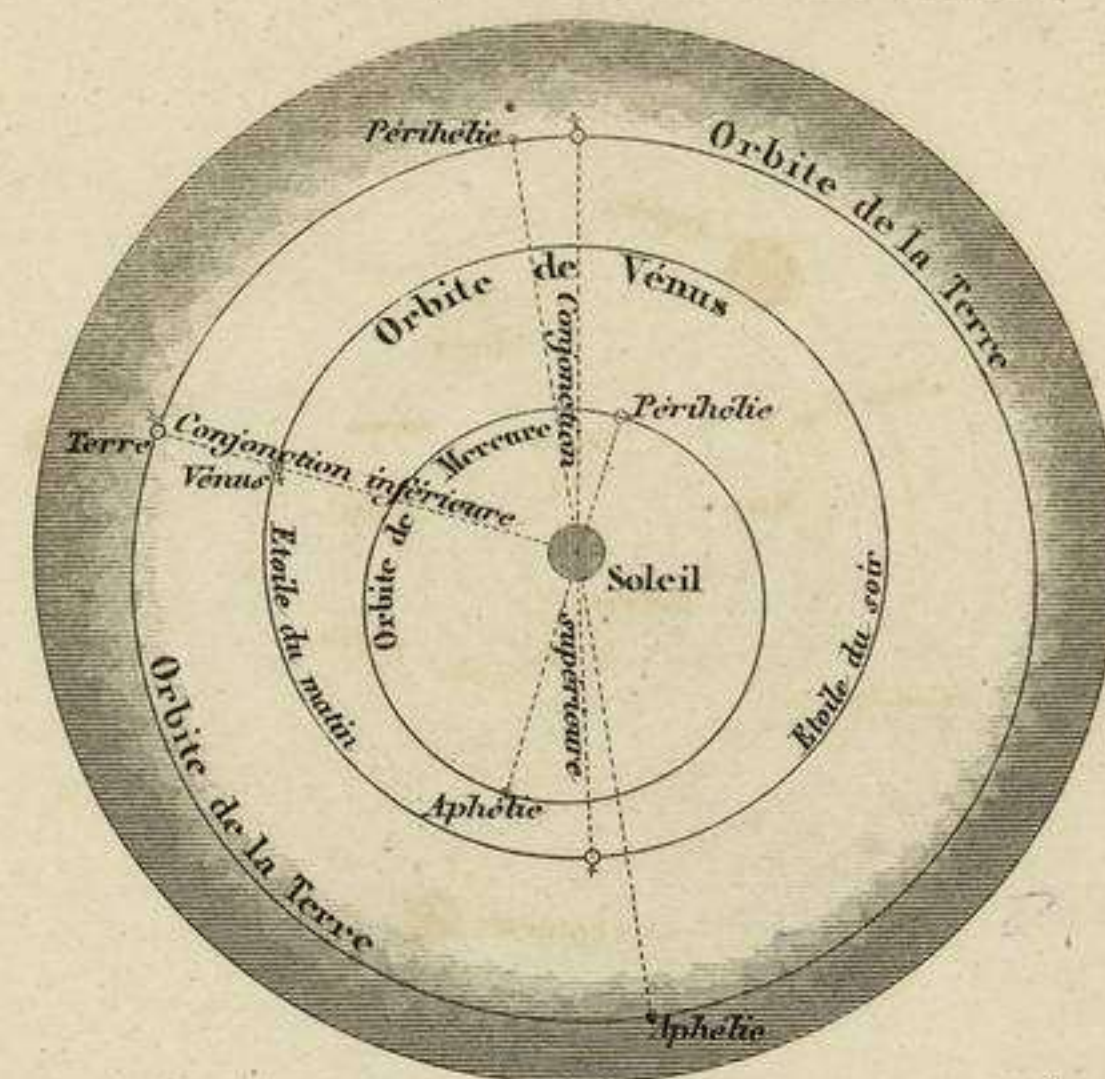
LA TERRE, VÉNUS ET MERCURE.
