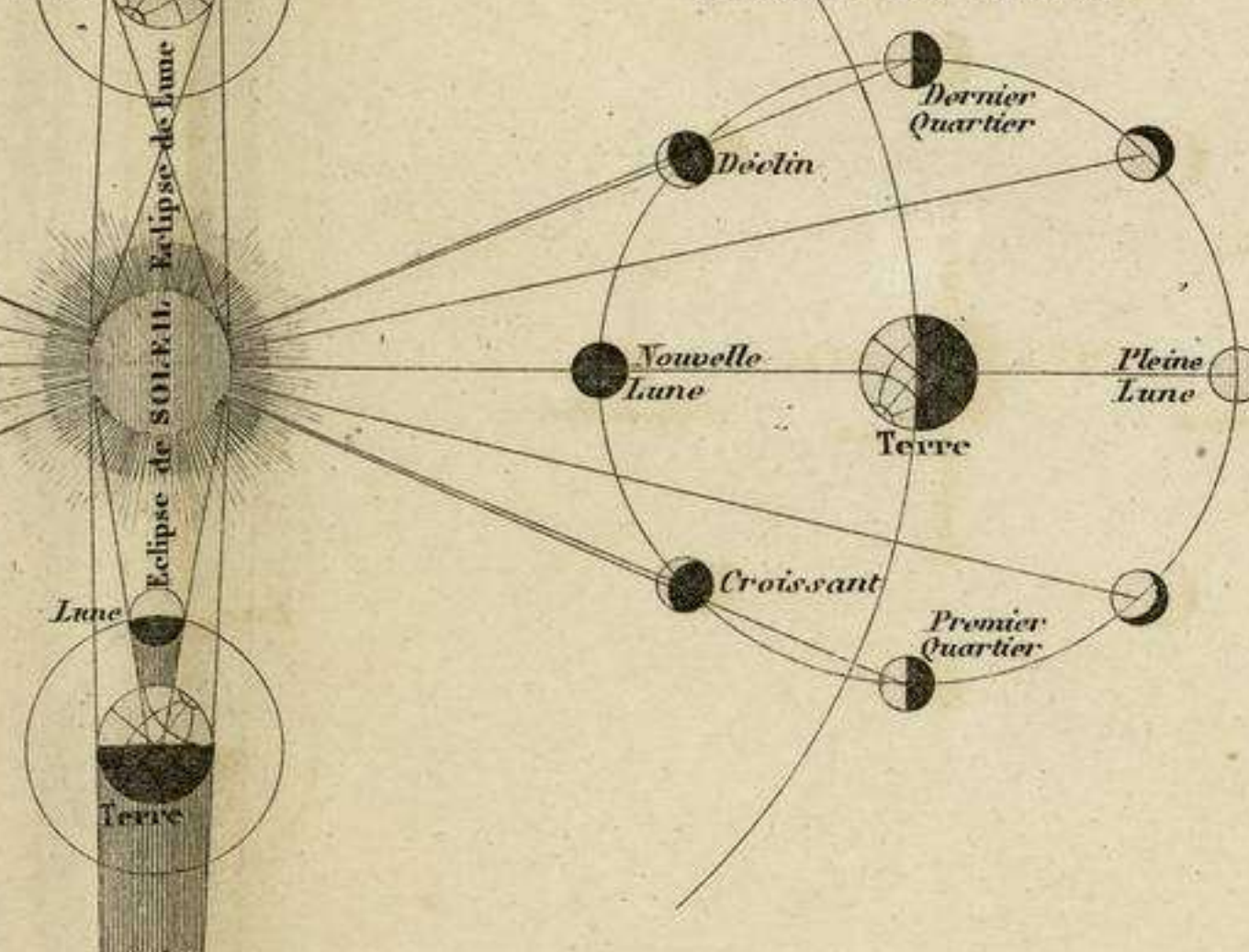
LE SOLEIL, LA TERRE ET LA LUNE.
