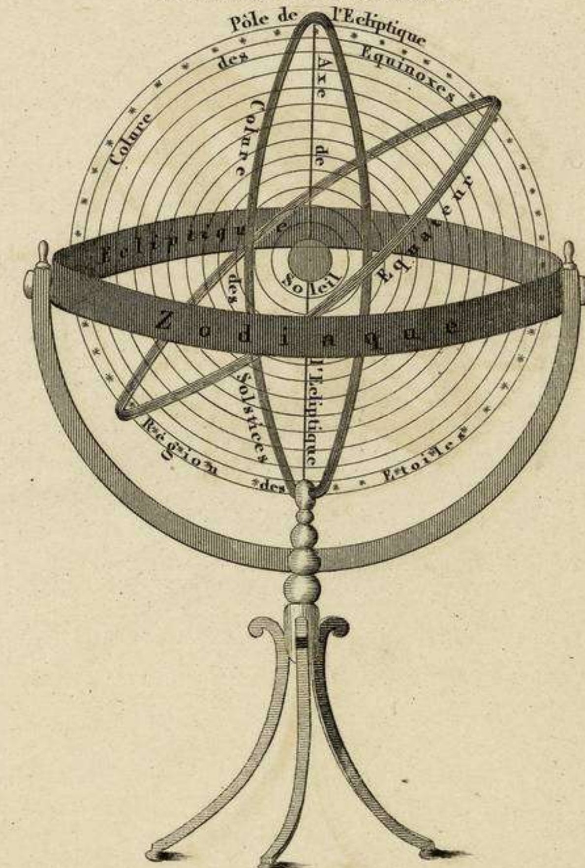
SYSTÈME DE COPERNIC.
