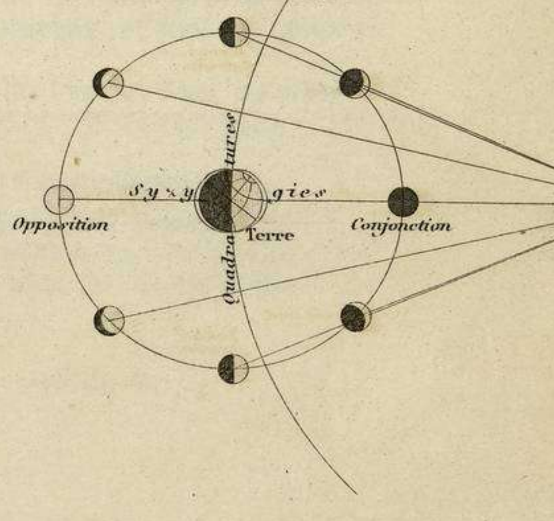
LE SOLEIL, LA TERRE ET LA LUNE.
