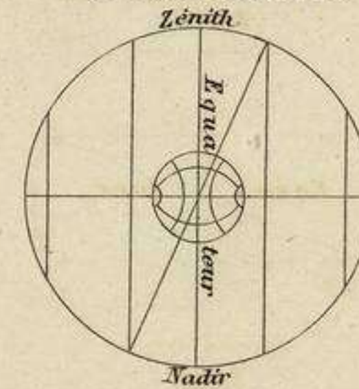
SPHÈRE DROITE.
