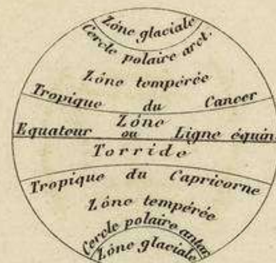
ZONES, CERCLES.
