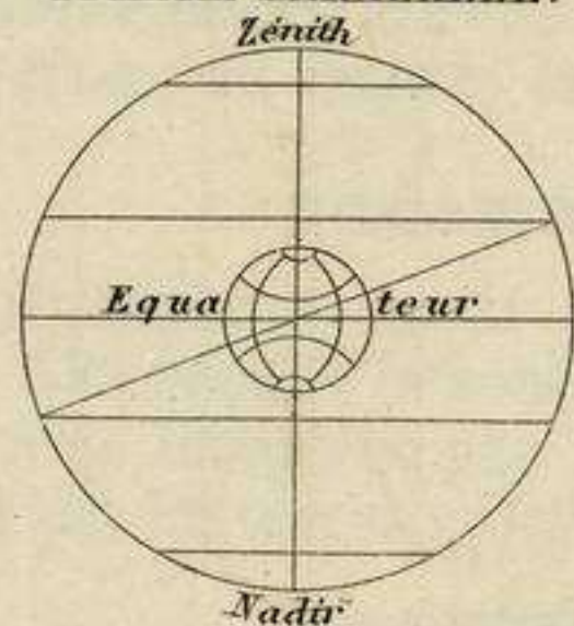
SPHÈRE ARMILLAIRE.
