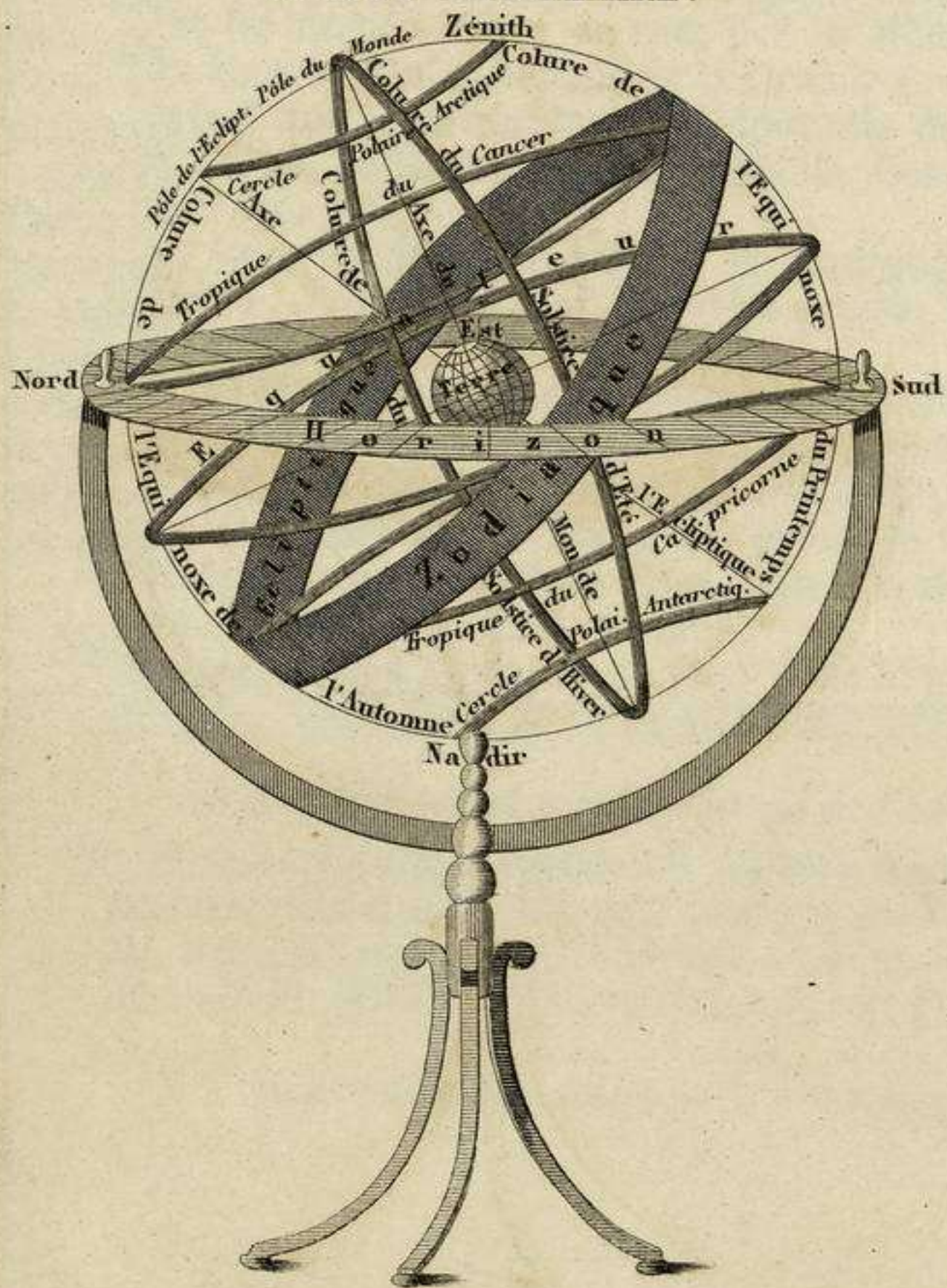
SPHÈRE ARMILLAIRE.
