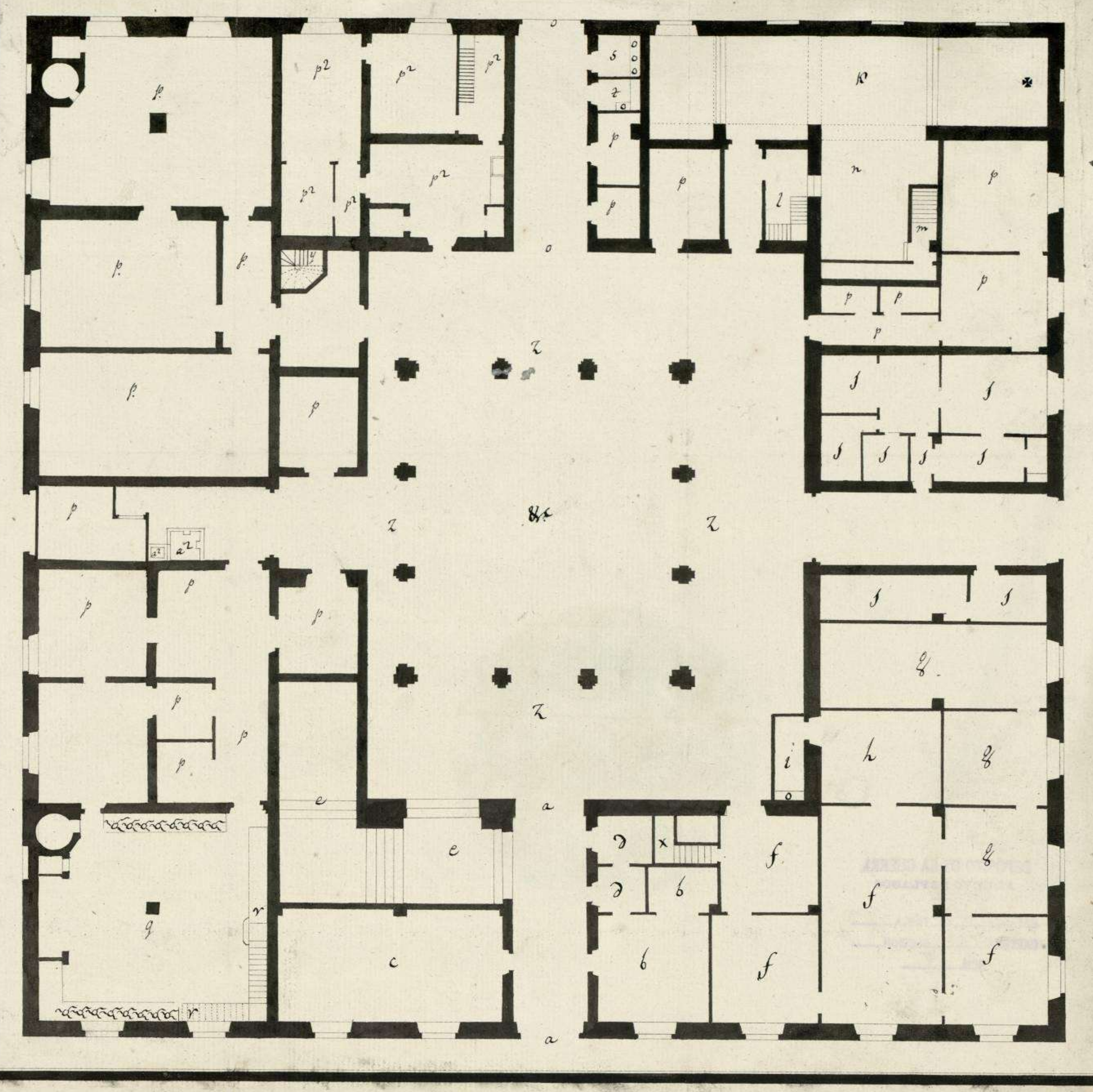
Plano del Piso Principal del R. Palacio de Barcelona
