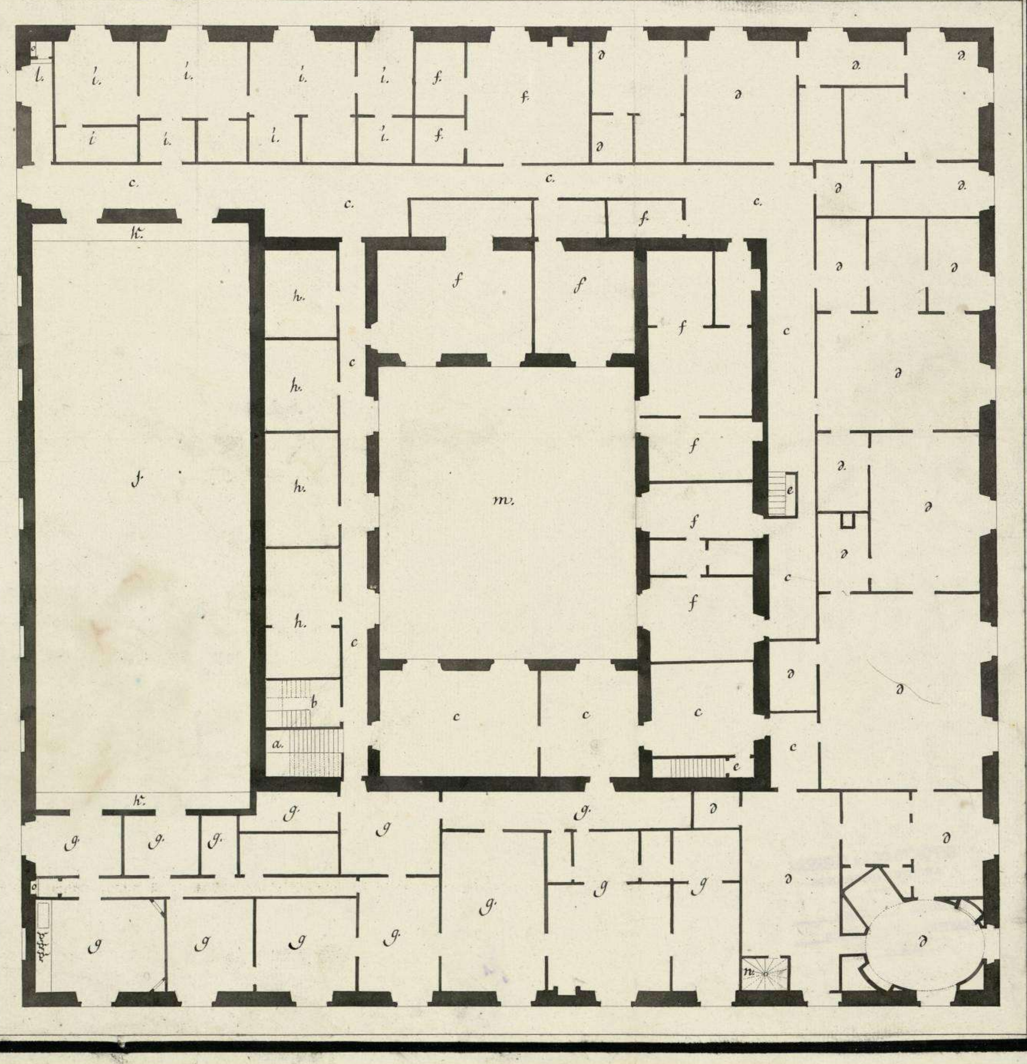
Plano del piso segundo del R. Palacio de esta Plaza en que se manifiesta la distribución interior que se ha dado después de la salida de S. M. N. para volverlo a habitar los Capitanes Generales y demas individuos segun costumbre con arreglo a lo prevenido en la R. O. de 24 de Noviembre de 1802.
