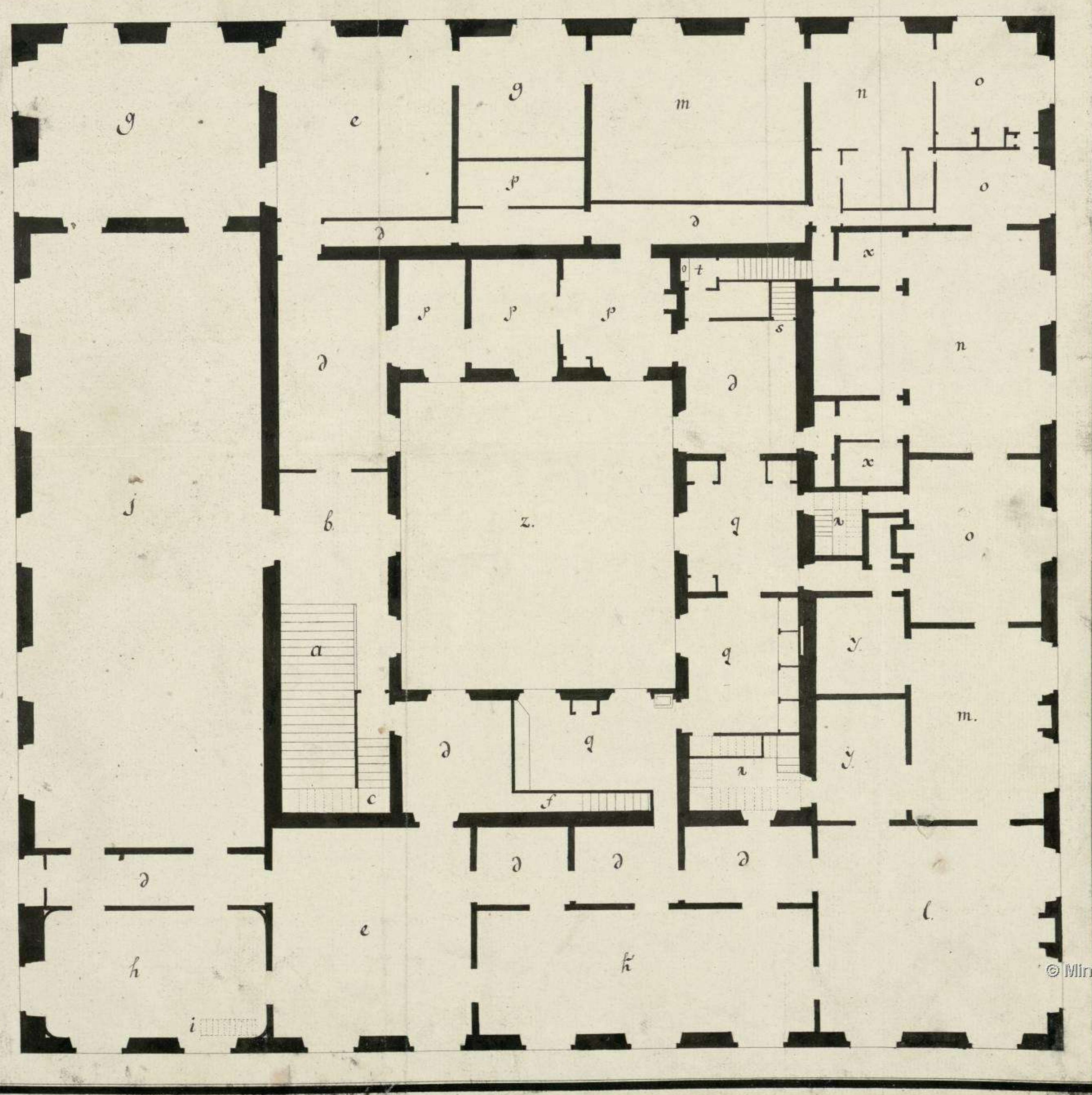
Plano del piso principal del R. Palacio de esta Plaza en que se manifiesta la distribución interior que se ha dado después de la salida de S. M. N. para volverlo a habitar los Capitanes Generales y demas individuos segun costumbre con arreglo a lo prevenido en la R. O. de 24 de Noviembre de 1802.
