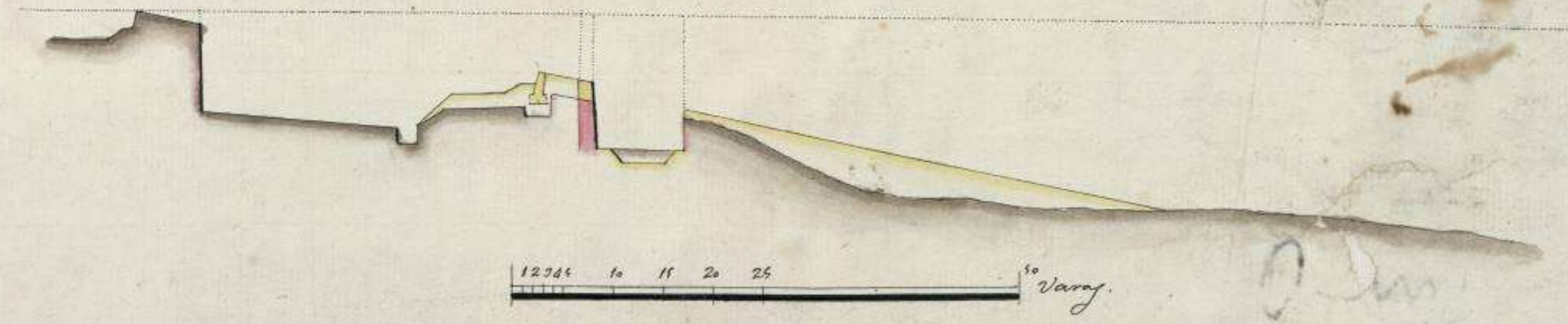
Perfil n.º 6 por la línea 30, 31, del Papel volante n.º 1.º
