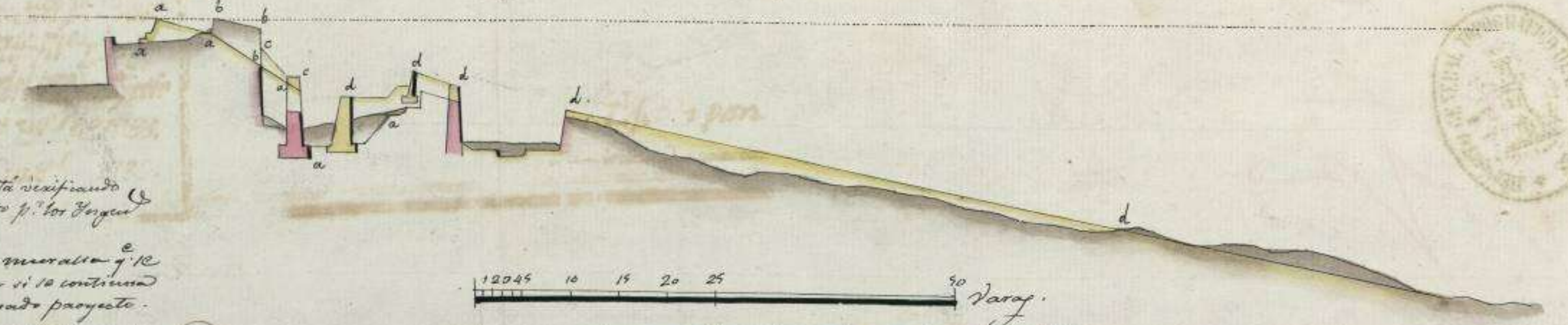
Perfil n.º 7 por la línea 34, 35, del papel volante n.º 1.º
