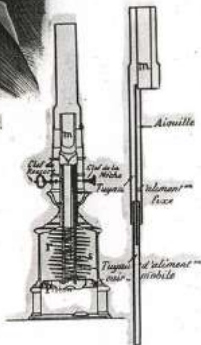
LAMPE MODÉRATEUR
