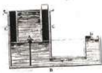
— Mécanisme de la lampe à niveau constant.
