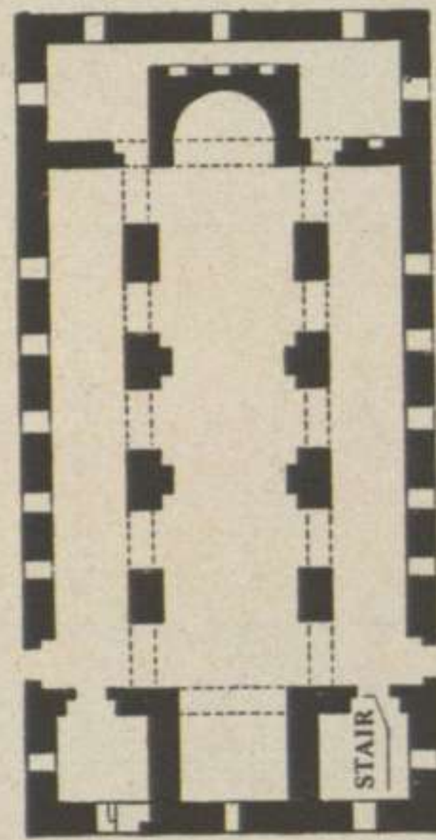
Fig. 23. — Wadi Ghazali (Somers Clarke) Escala 1:400
