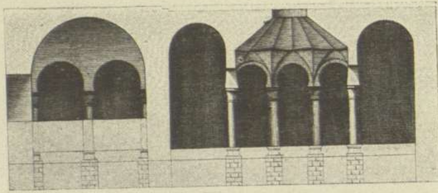
Esc. 1:400 Fig. 10. — Banys de Barcelona (Laborde)
