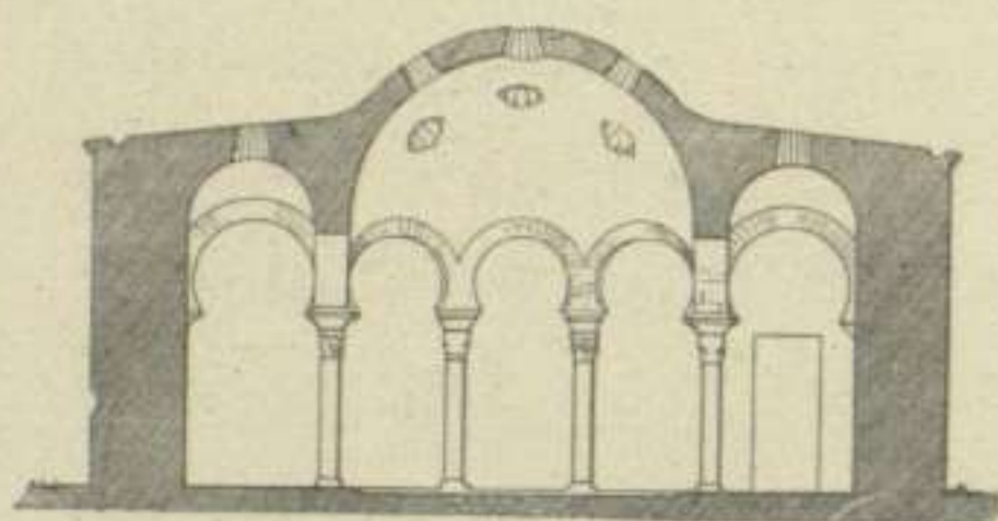
Fig. 5. — Banys de Palma. Secció
