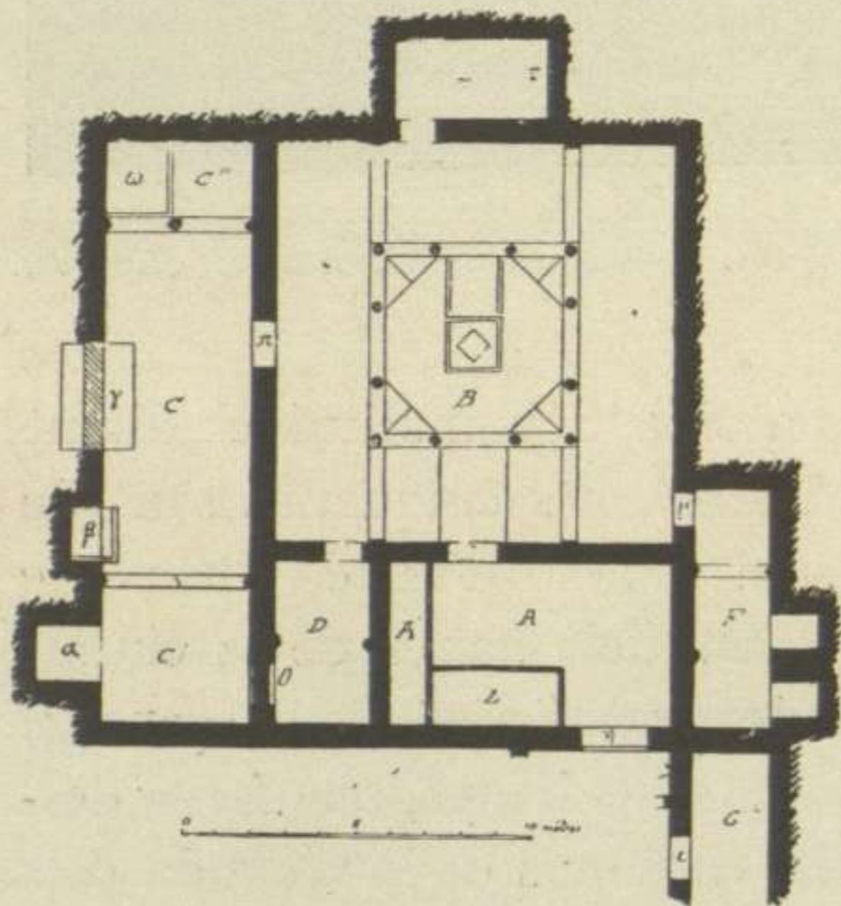
Fig. 14. — Banys dels tintorers de Tlemcen
