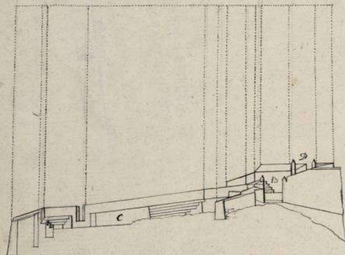
Perfil cortado p a la línea 3.4
