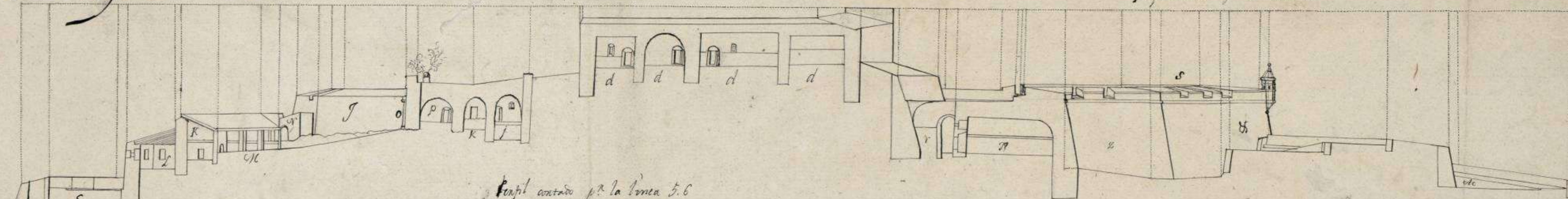
Perfil cortado p a la línea 1.2
