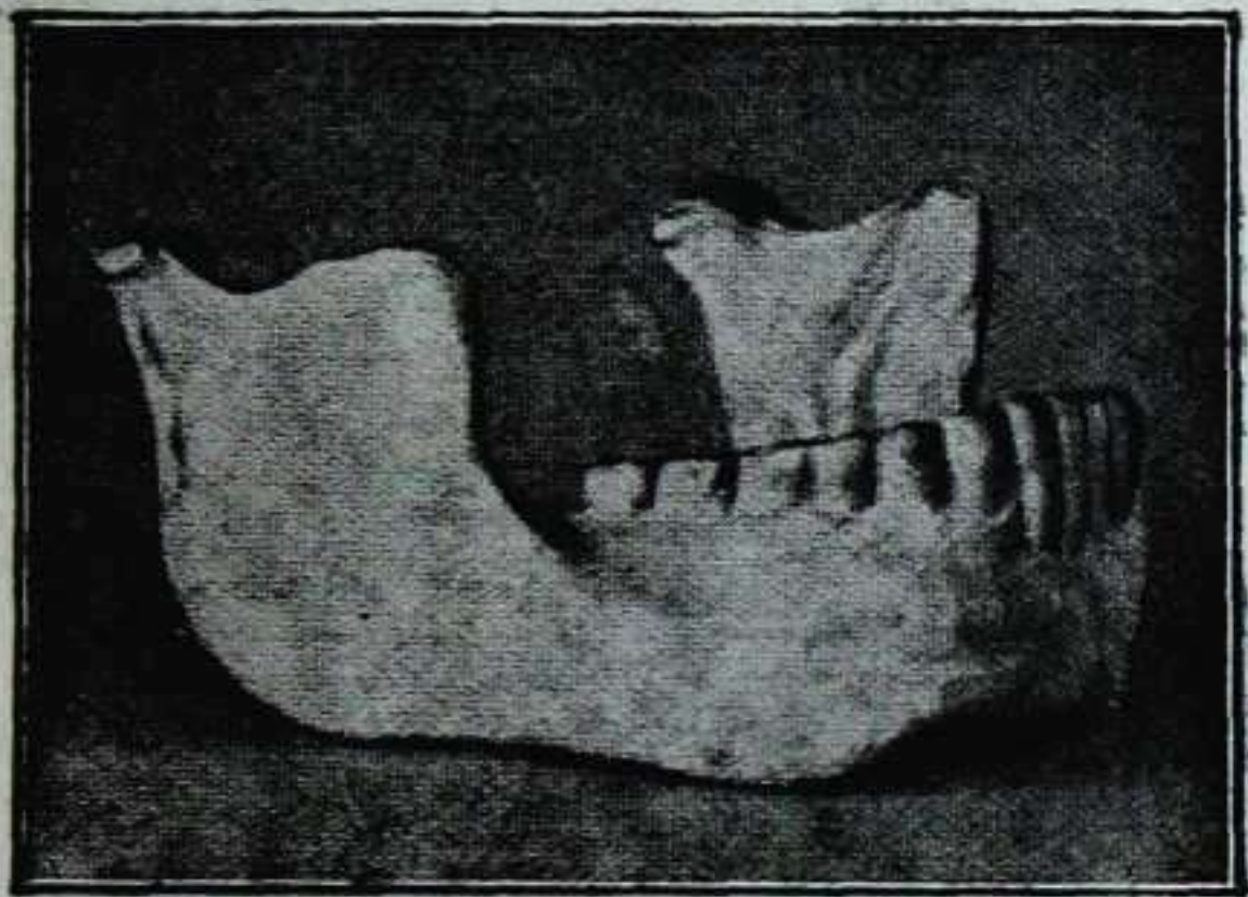
10 irudia.-Mauer'en arkitutako matrail- ezuía (Homo Heidelbergensis)
