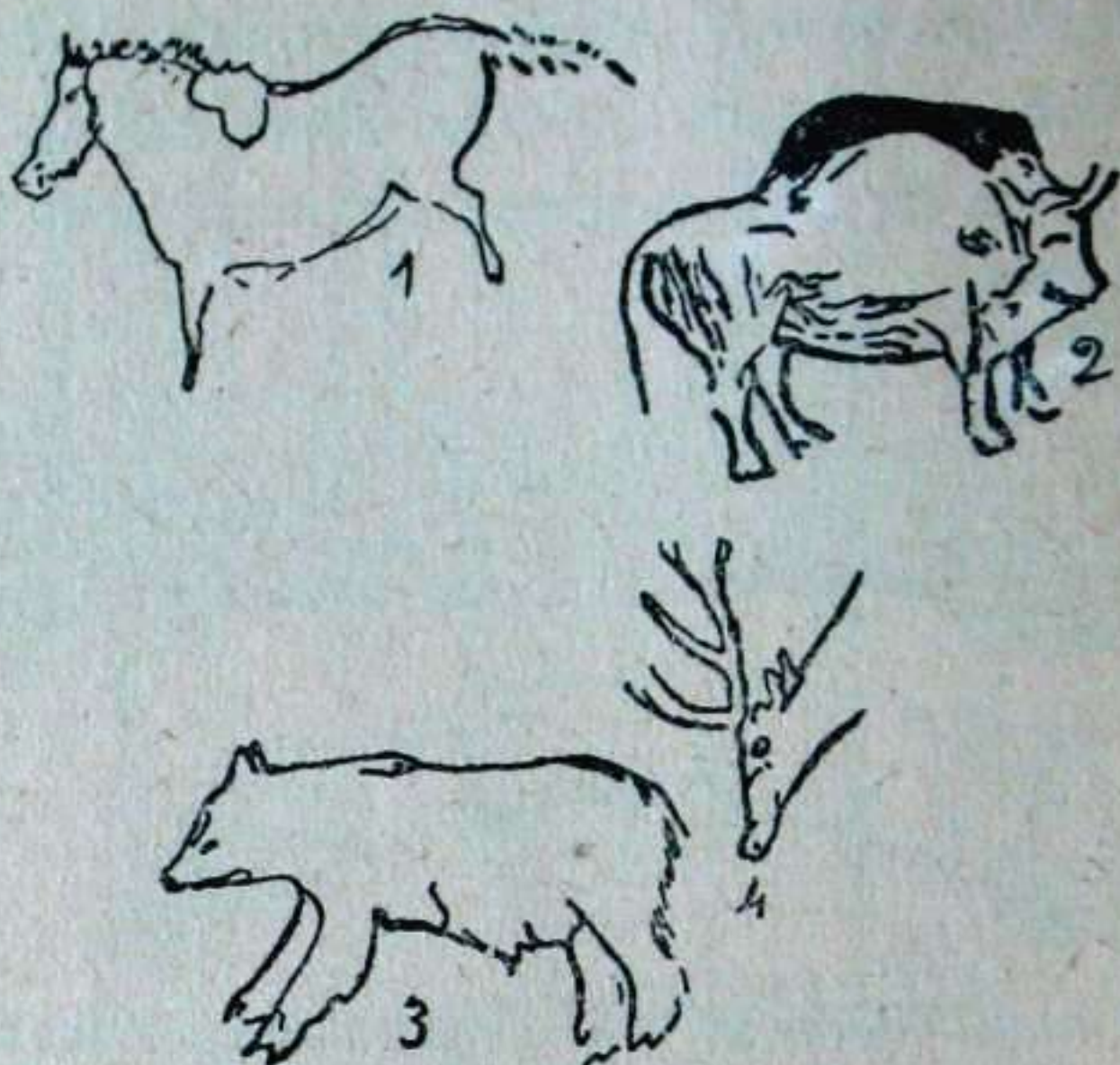
26 irudia.-Santimamiñe'ko madeleineta orma- mañazkintzak. 1, beoña; 2, bisona; 3, artza; 4, orein-burua.
