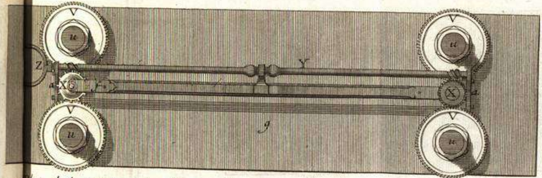
Plan de la Table et des pieces qui servent à serrer le Cylindre d'en haut.
