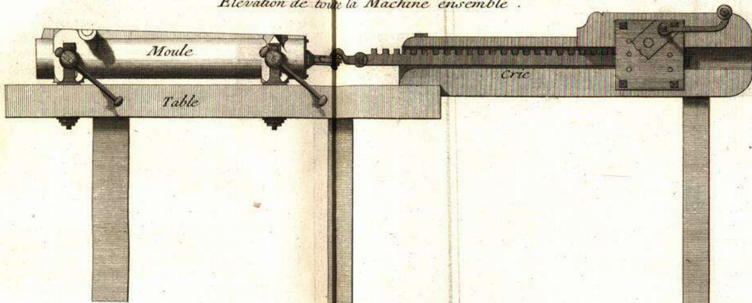
Elevation de toute la Machine ensemble.
