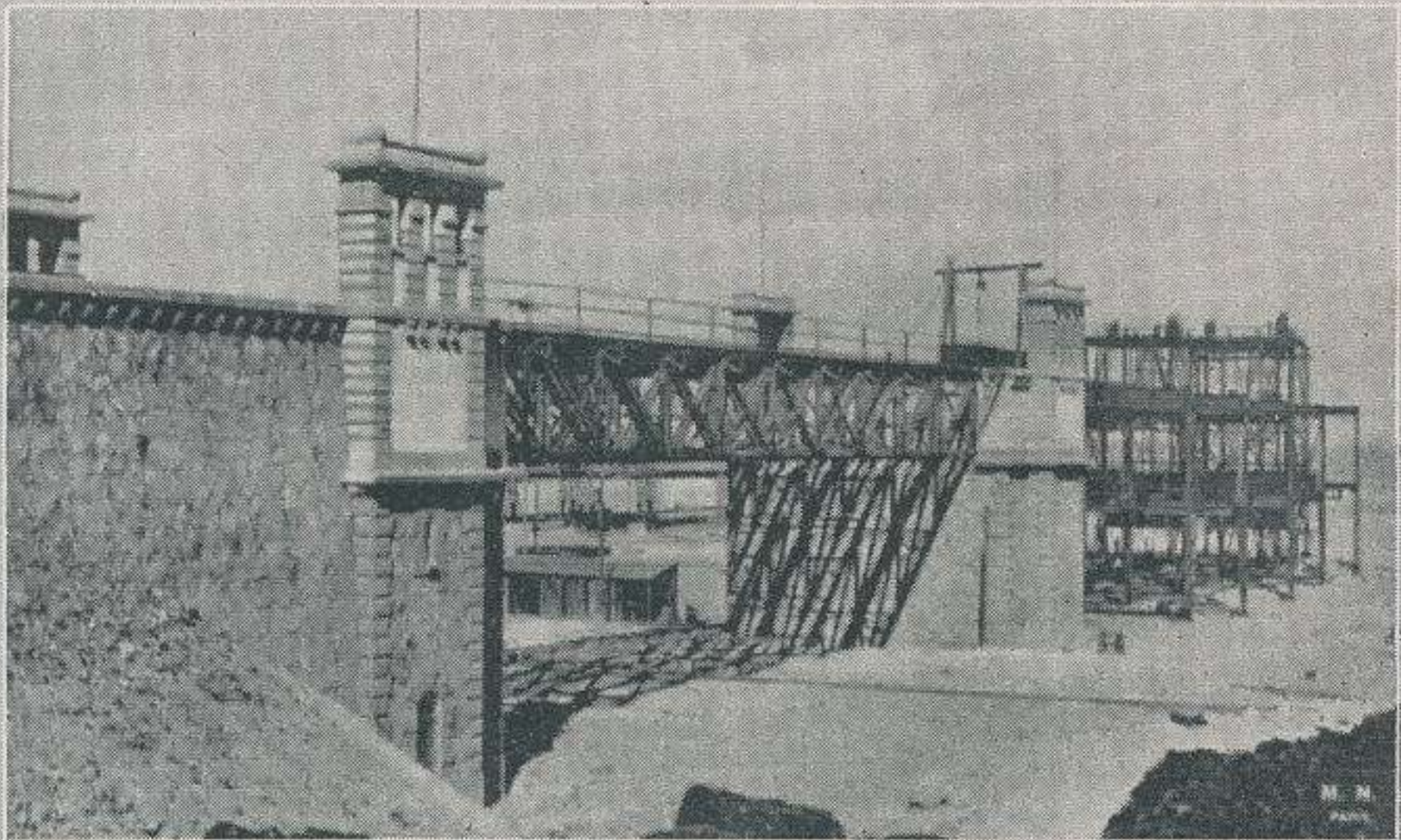
Musel: Puente del cargadero del Sindicato
