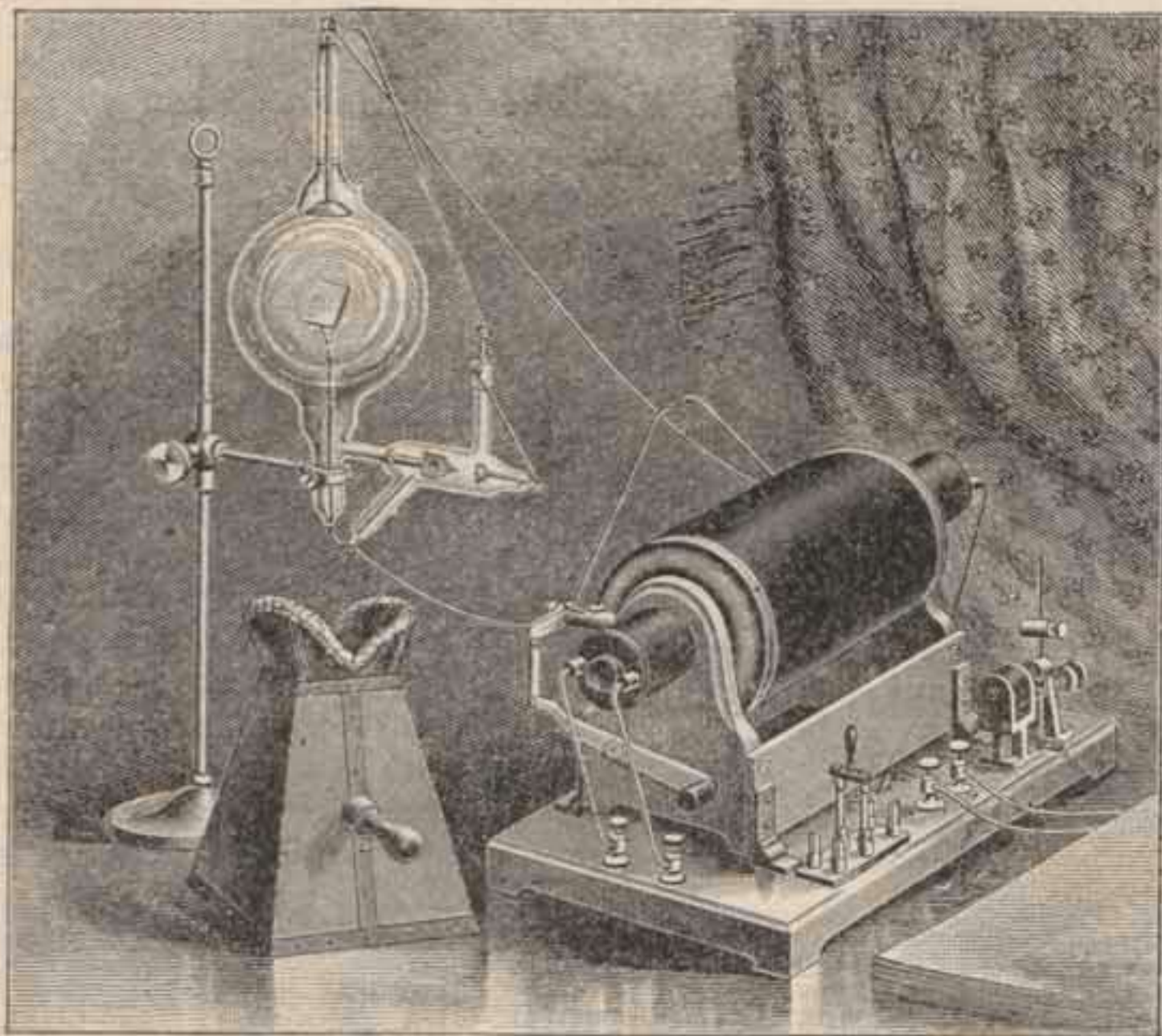
Fig. 534.—APARATOS PARA LOS RAYOS X
