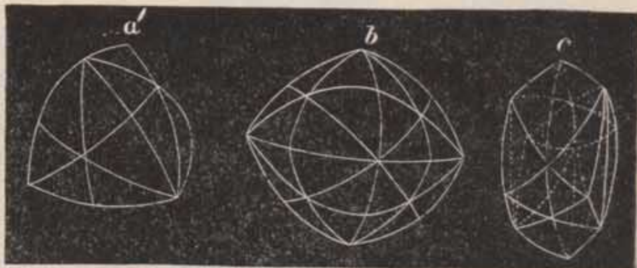
CRISTALES DEL DIAMANTE.
