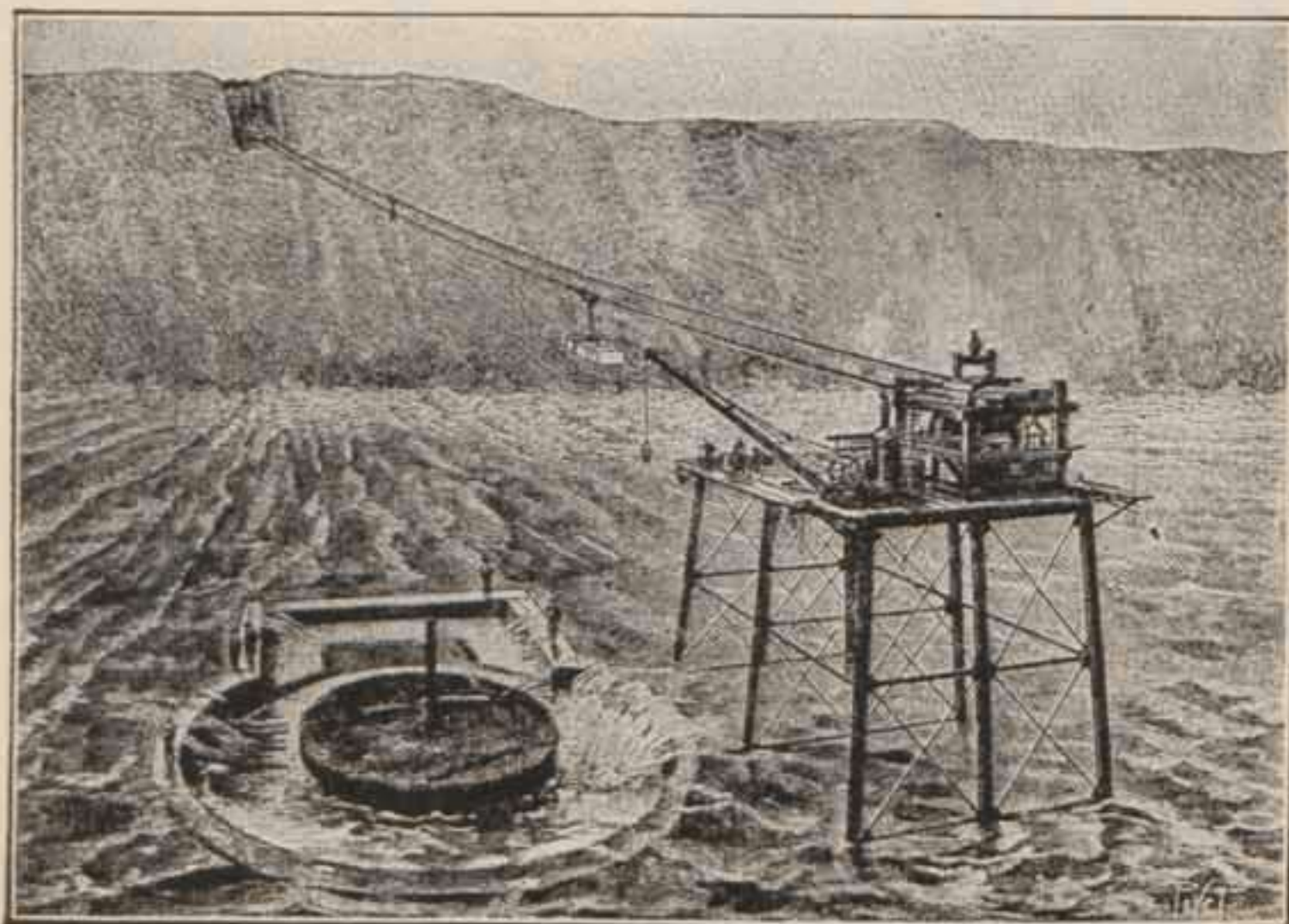
ALAMBRECARRIL PARA CONDUCCIÓN DE MATERIALES
