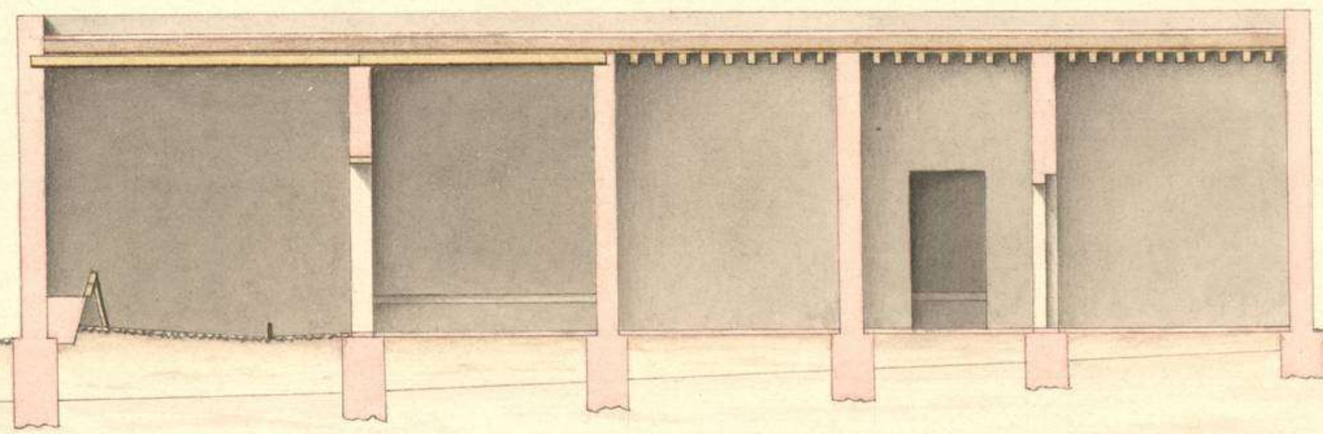
Perfil cortado por la linea A B
